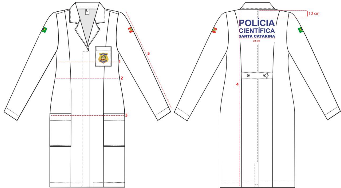
Figura 3: Figura com indicação das medidas básicas do jaleco de microfibra feminino.
