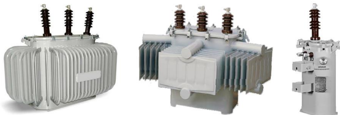
Figura 12 – Transformadores de distribuição de energia elétrica
