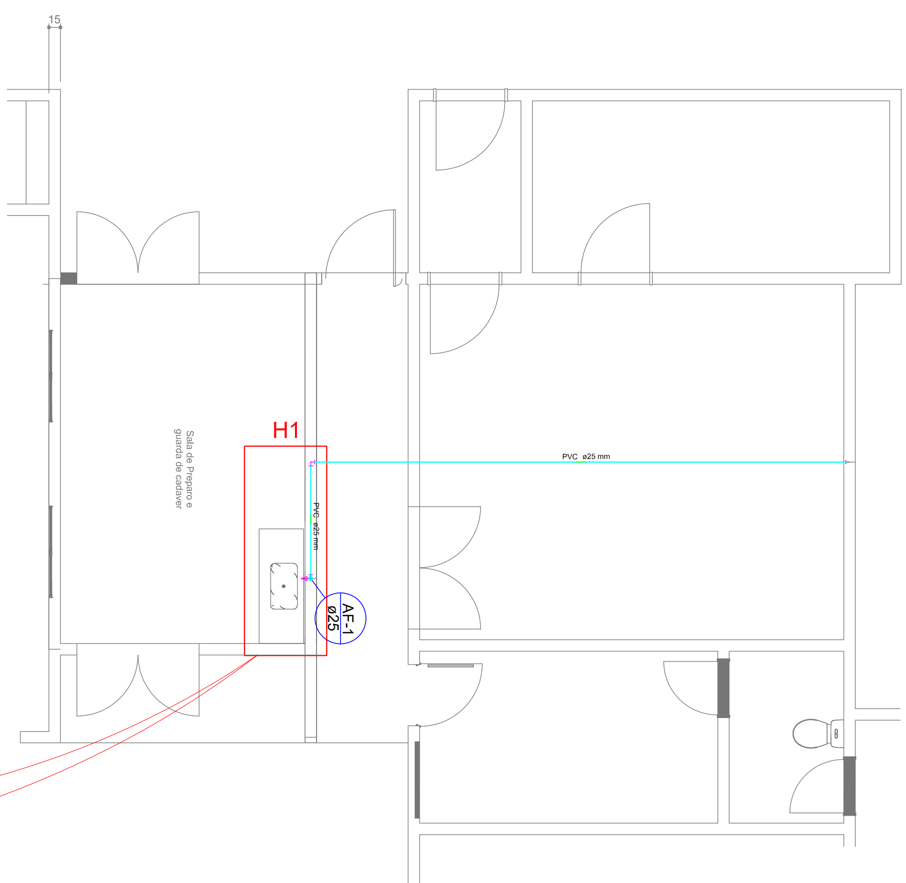
Planta da ampliação escala 1:50
