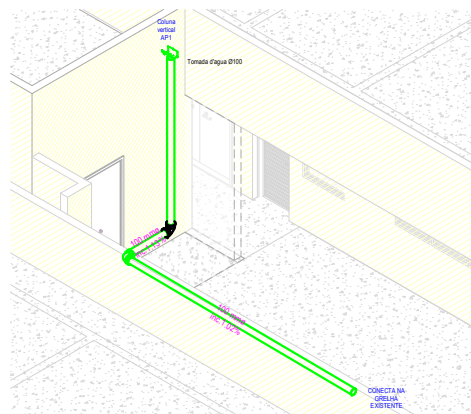
2 Isométrico
