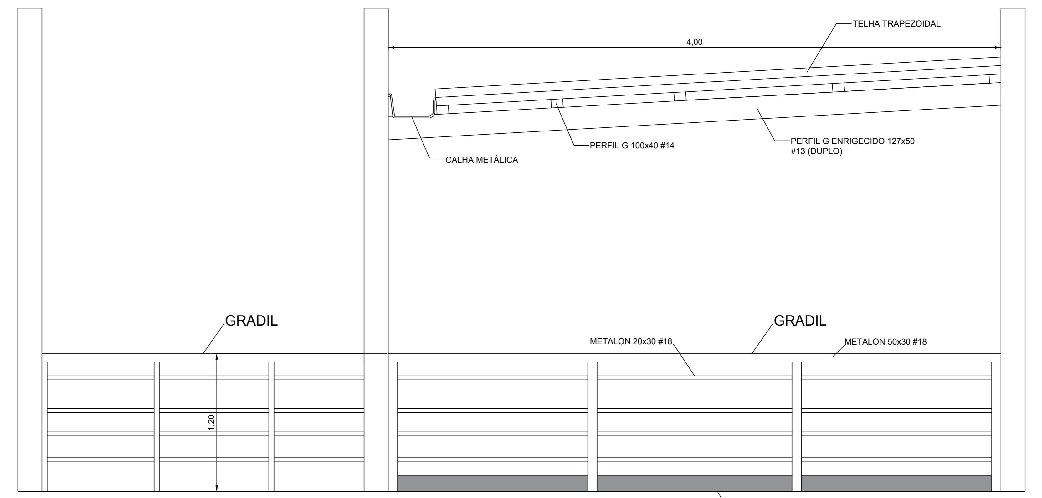
CORTE 1
