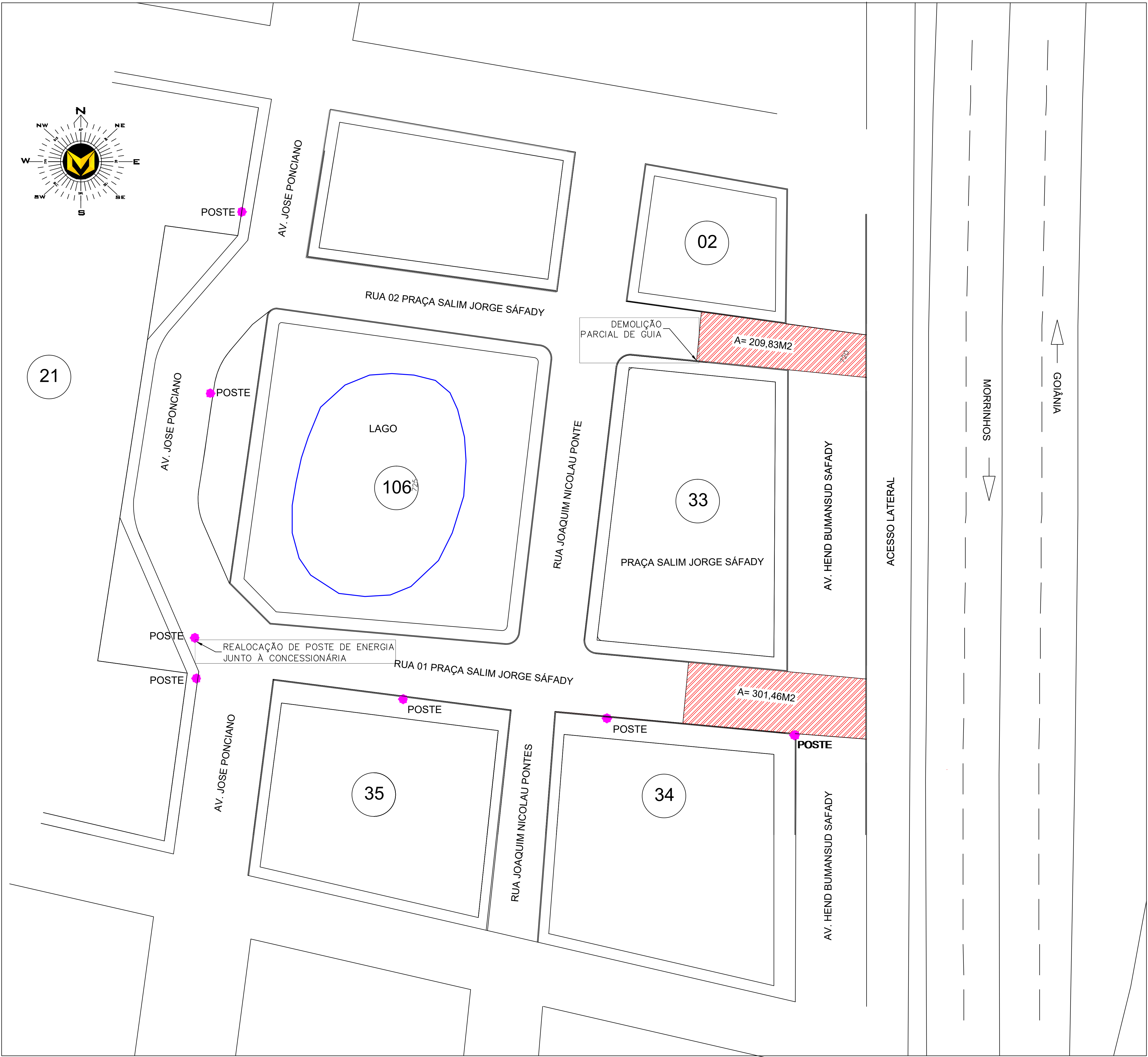
PLANTA BAIXA-DEMOLIÇÕES Esc.: 1:300
