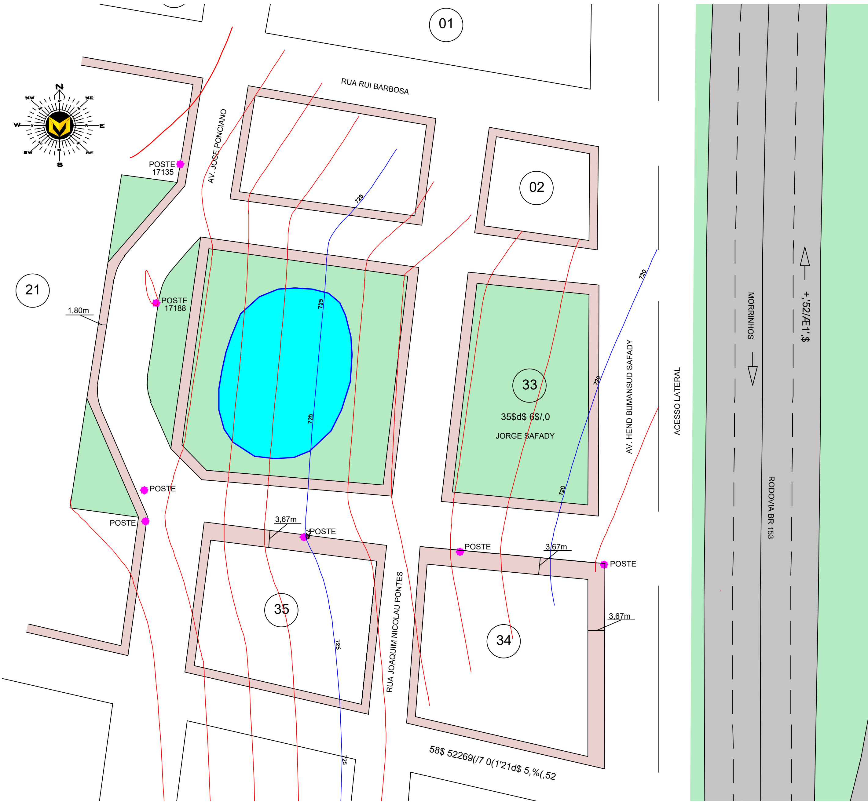
PLANTA DE TOPOGRAFIA Esc.: 1:500
