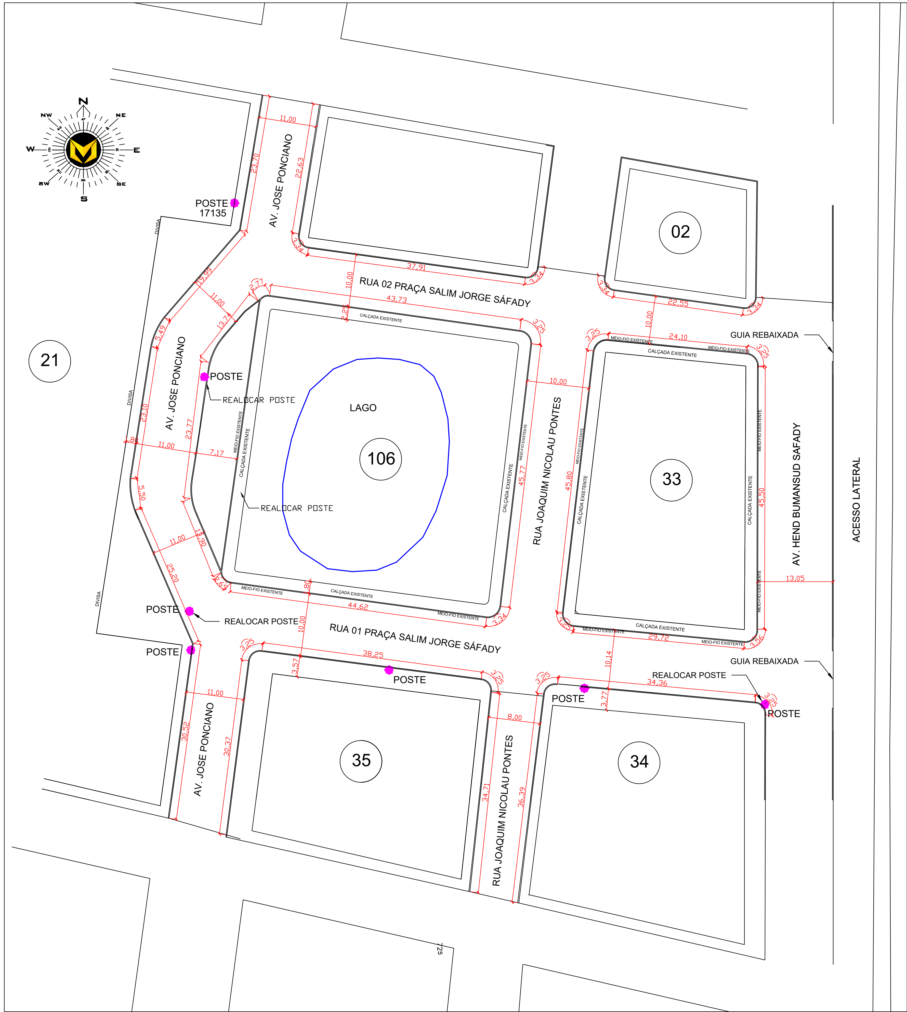
PLANTA BAIXA-PAVIMENTAÇÃO COM COTAS Esc.: 1:500
