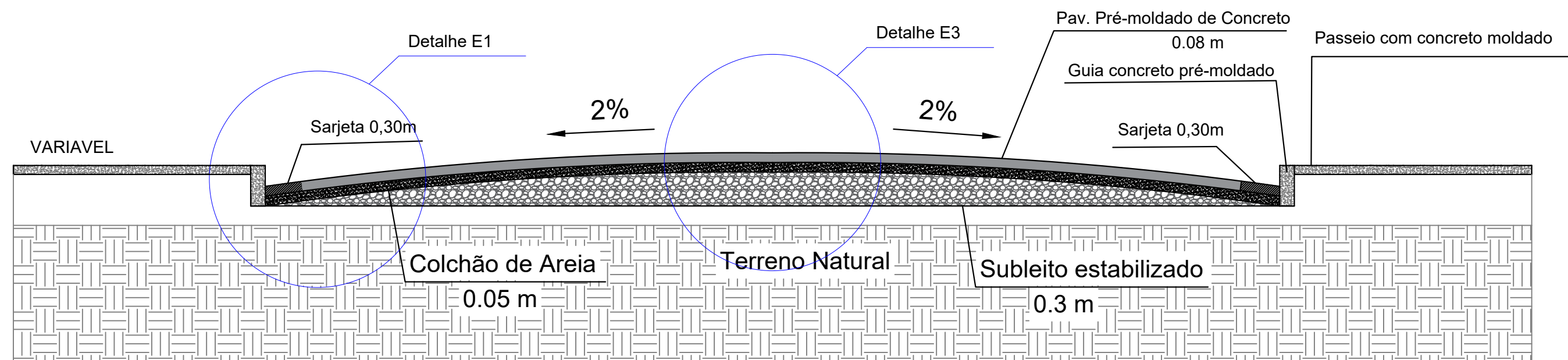
SEÇÃO TRANSVERSAL VIA ABaulada Escala: s/ escala
