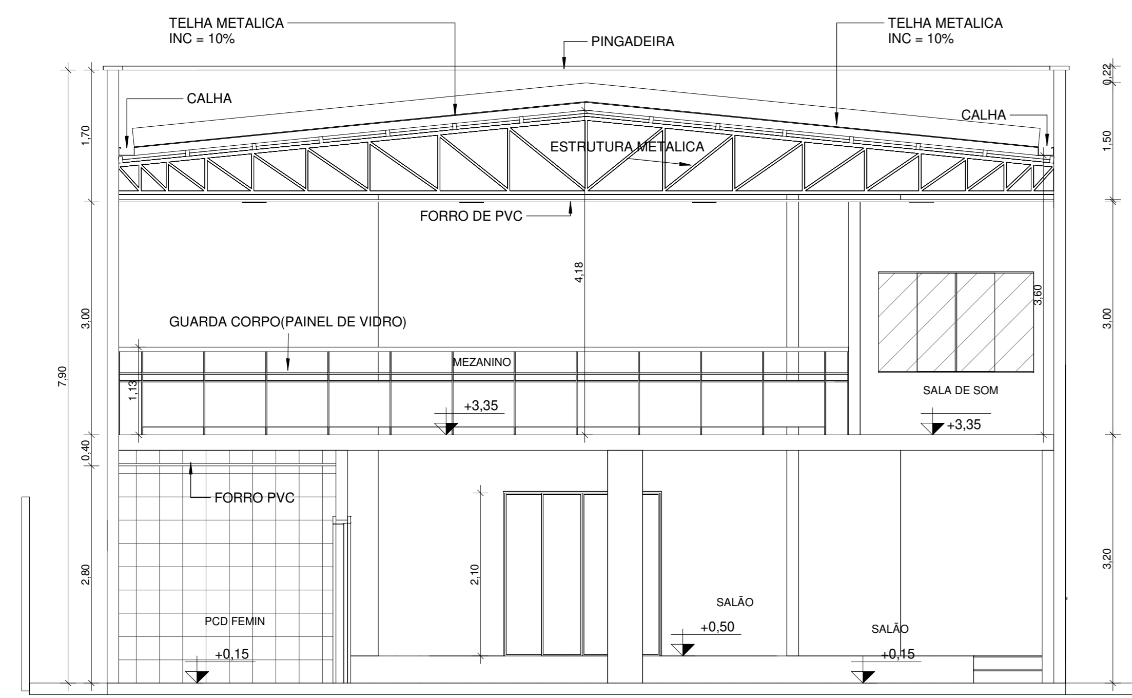
CORTE AA 1:50
