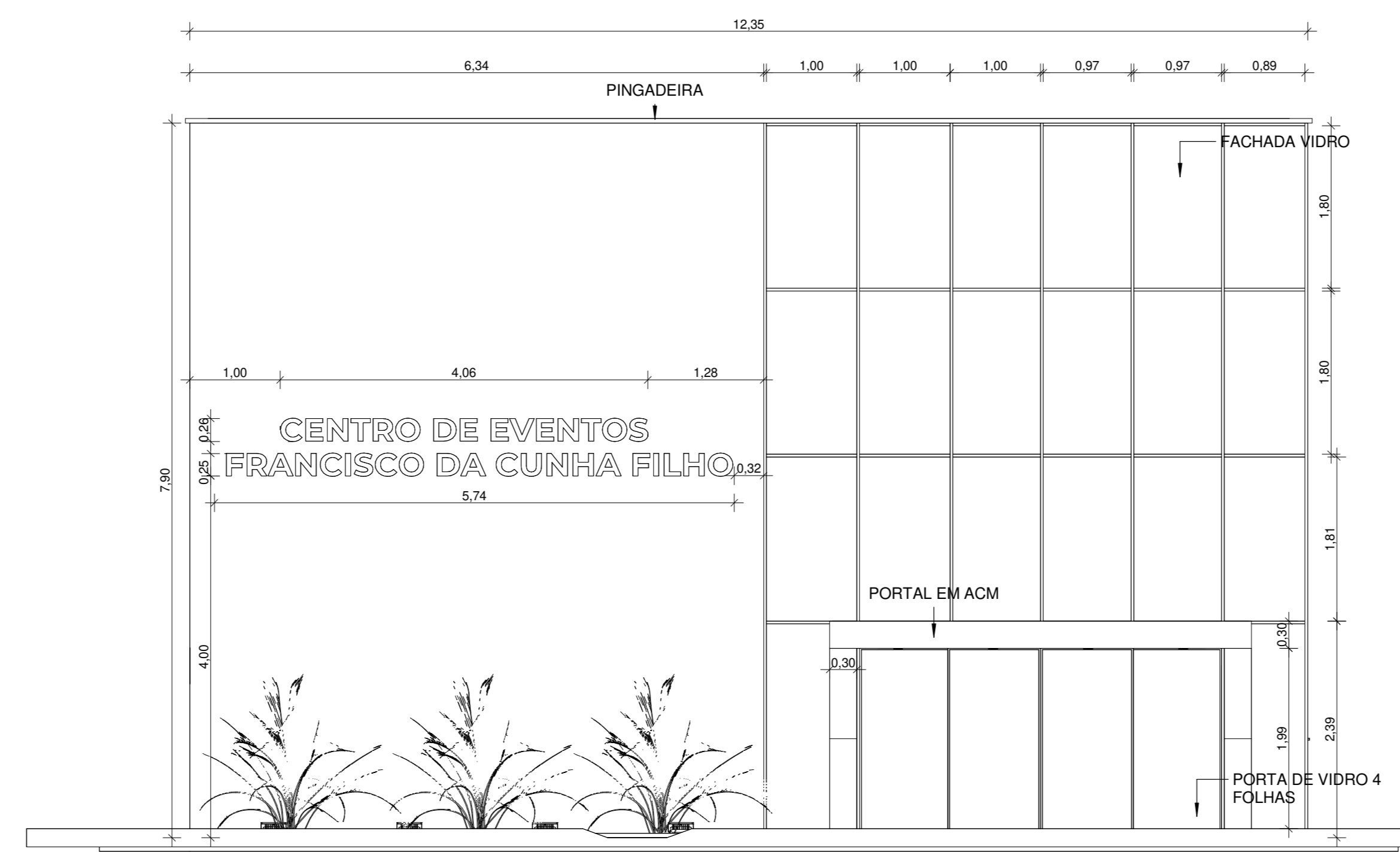
Fachada Frontal 1:50
