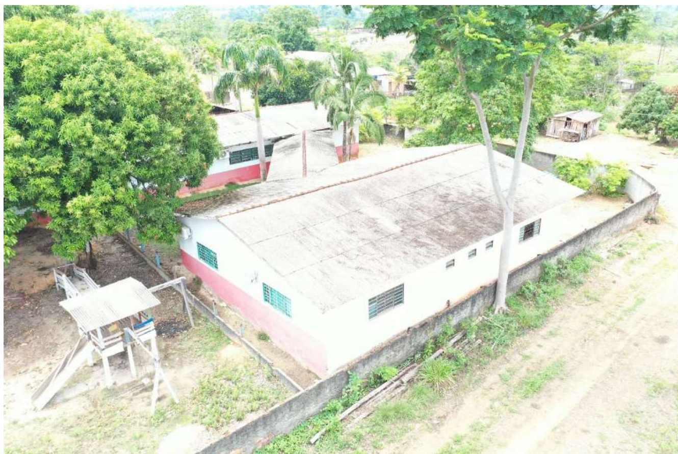
Bloco Salas Fundo existente em Alvenaria – Reformar com troca de pisos, troca de telhado, troca de forro, instalações, adequação de rampas e nova pintura.
