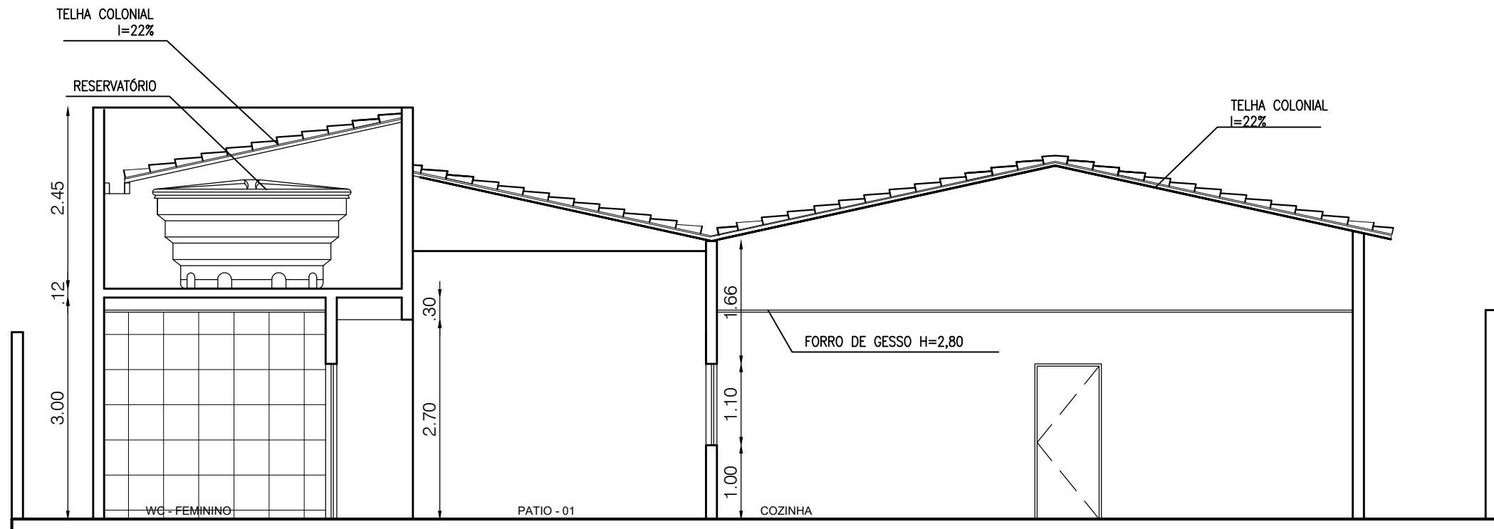
CORTE 02 ESCALA 1/50
