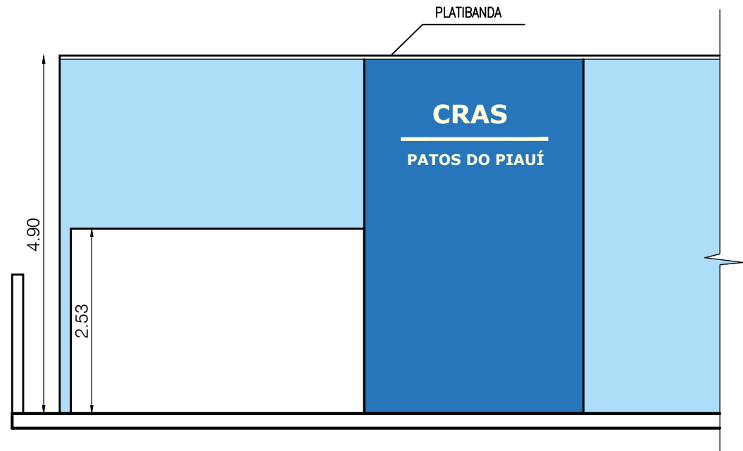
FACHADA 01 ESCALA 1/50
