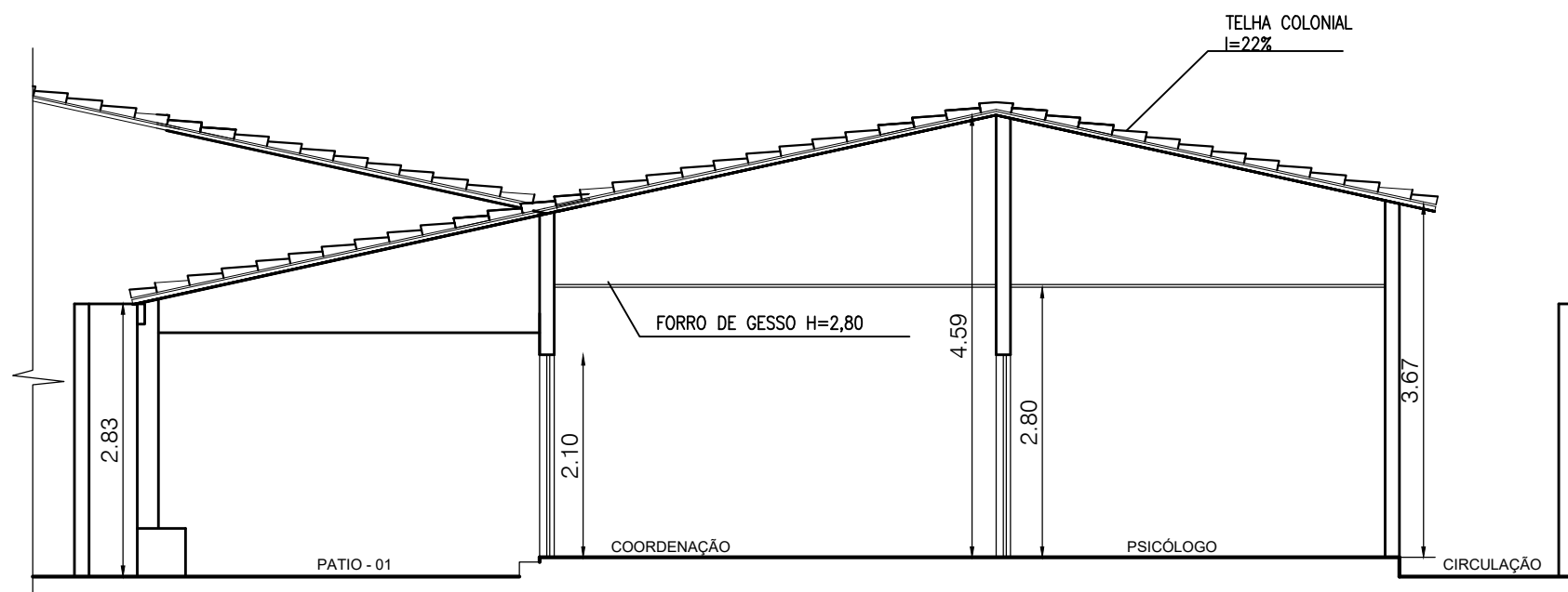
CORTE 01 ESCALA 1/50
