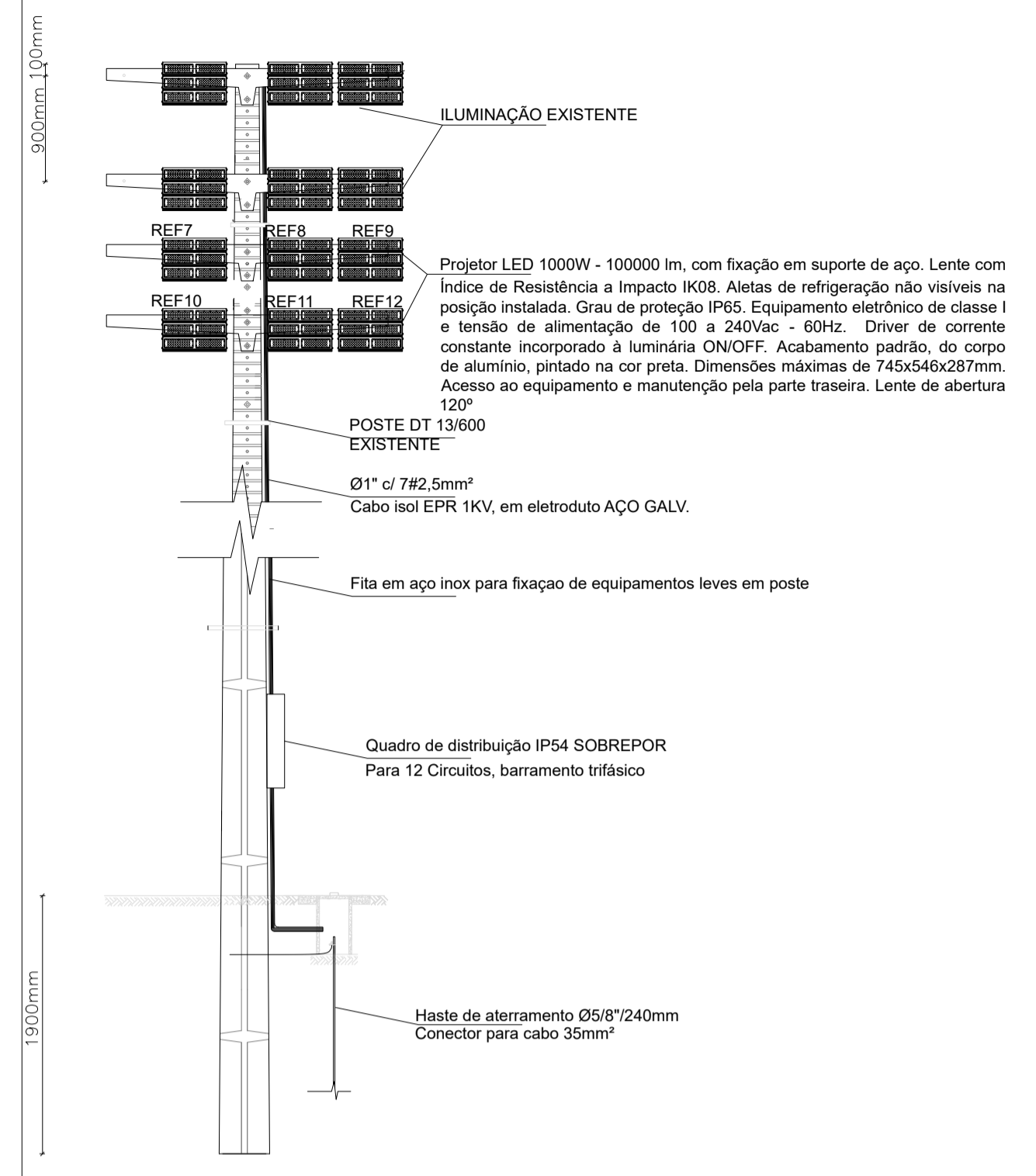
DETALHE 01 - POSTE E REFLETORES Esc. S/ESC.
