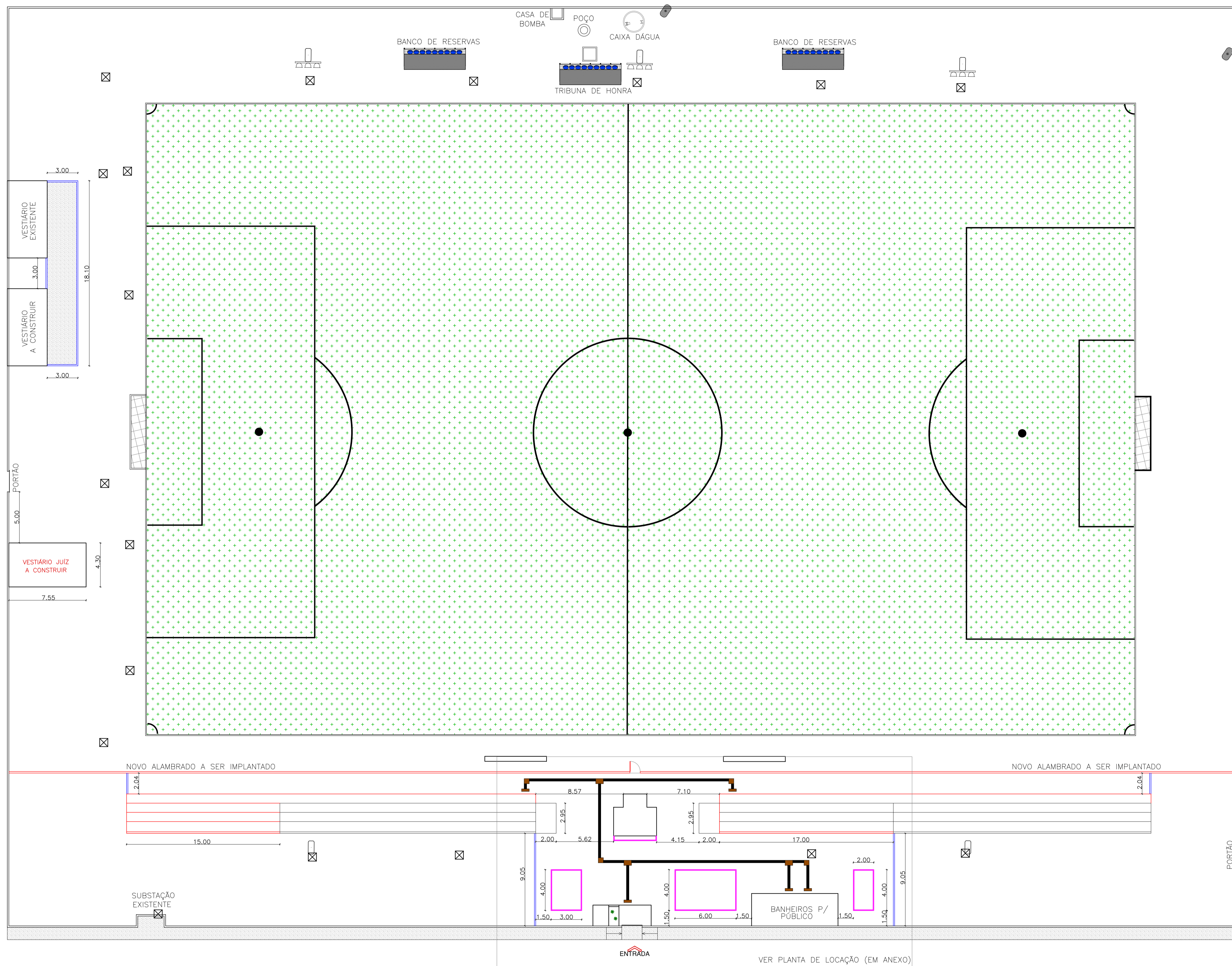
PLANTA BAIXA DE EXECUÇÃO - LOCAÇÃO DE CANTEIROS ESCALA 1/200
