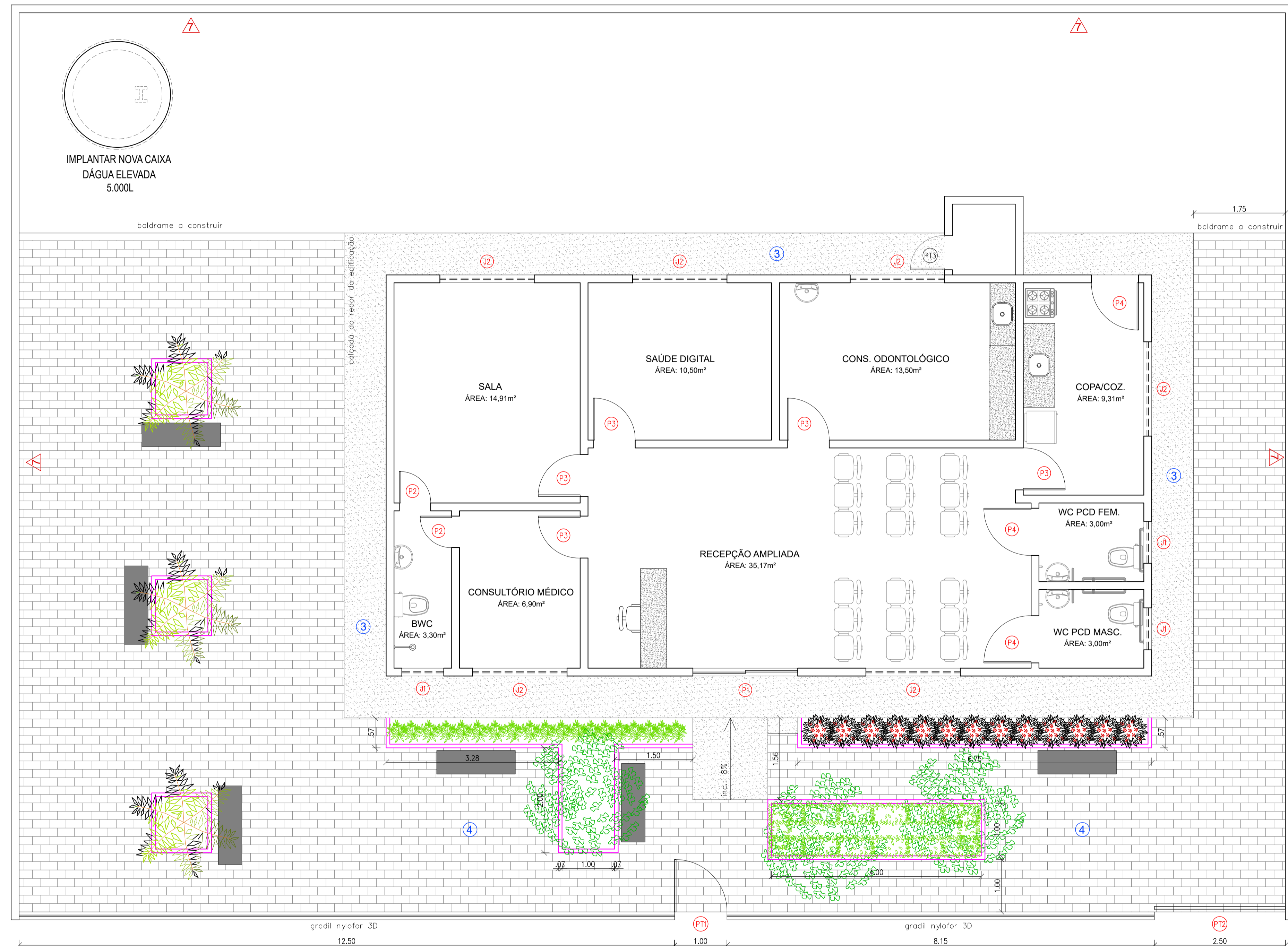
PLANTA DE IMPLANTAÇÃO REFORMADA ESCALA 1/50
