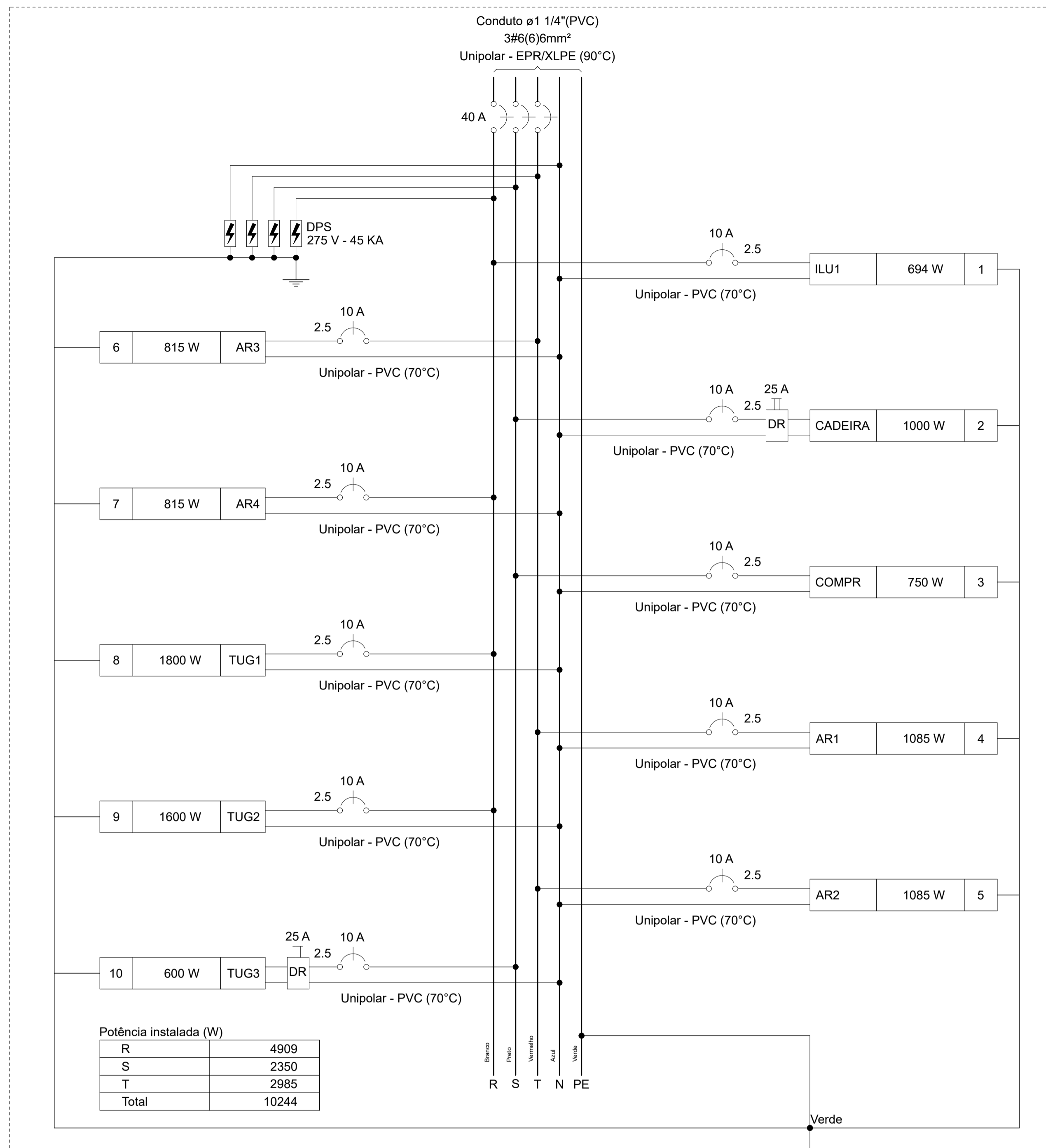
Quadro de Cargas (QDLF) - Pavimento
