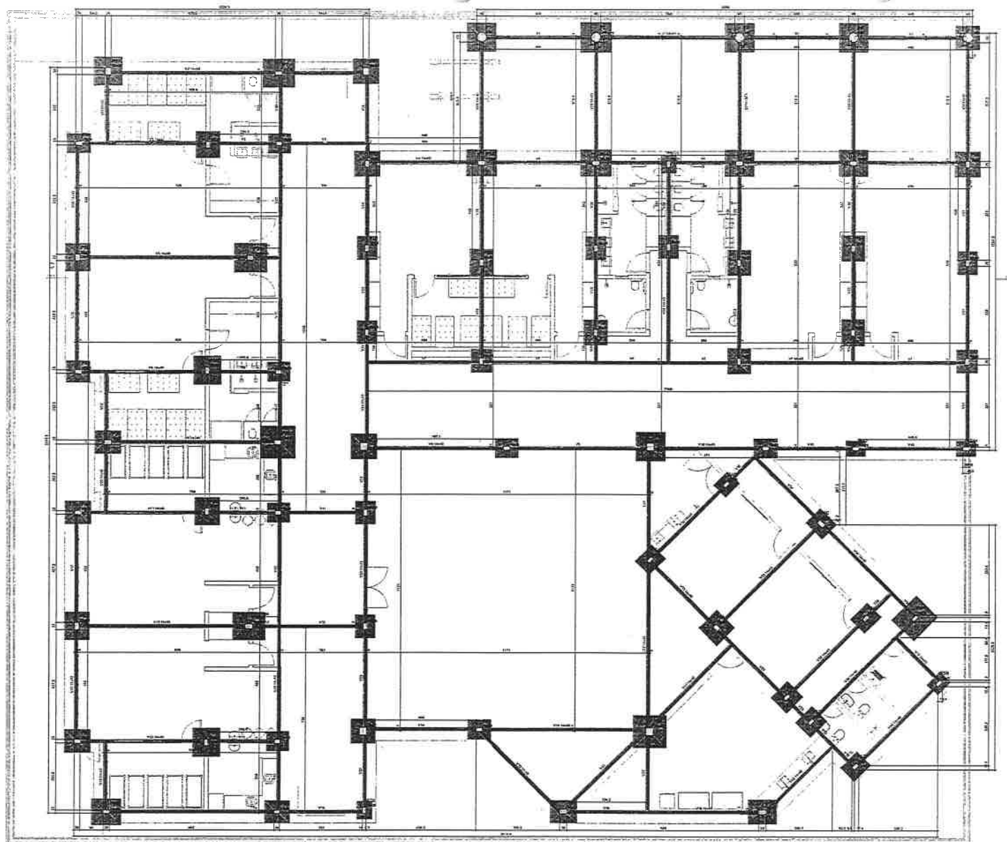
FORMA DO PAVIMENTO TÉRREO (NÍVEL 0)
