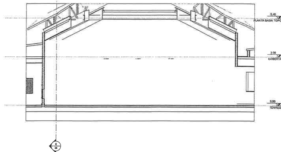
4 CORTE 9-9 1:50
