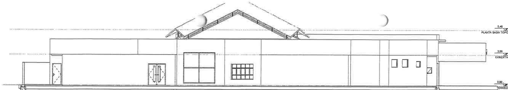
3 ELEVÇÃO FRONTAL 1:75
