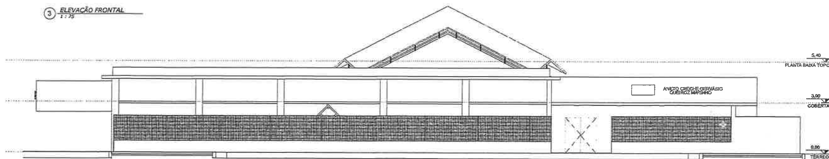
4 ELEVÇÃO POSTERIOR 1:75
