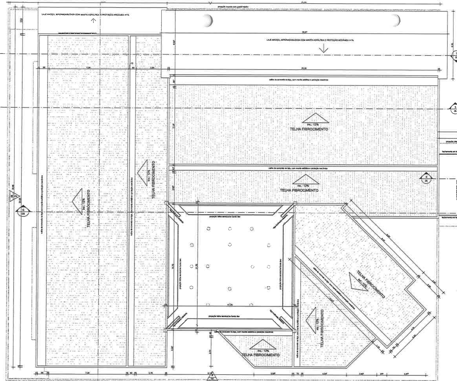
① PLANTA BAIXA COBERTA 1:75
