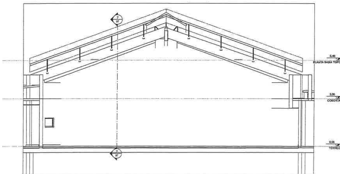
3 CORTE 8-8 1:50
