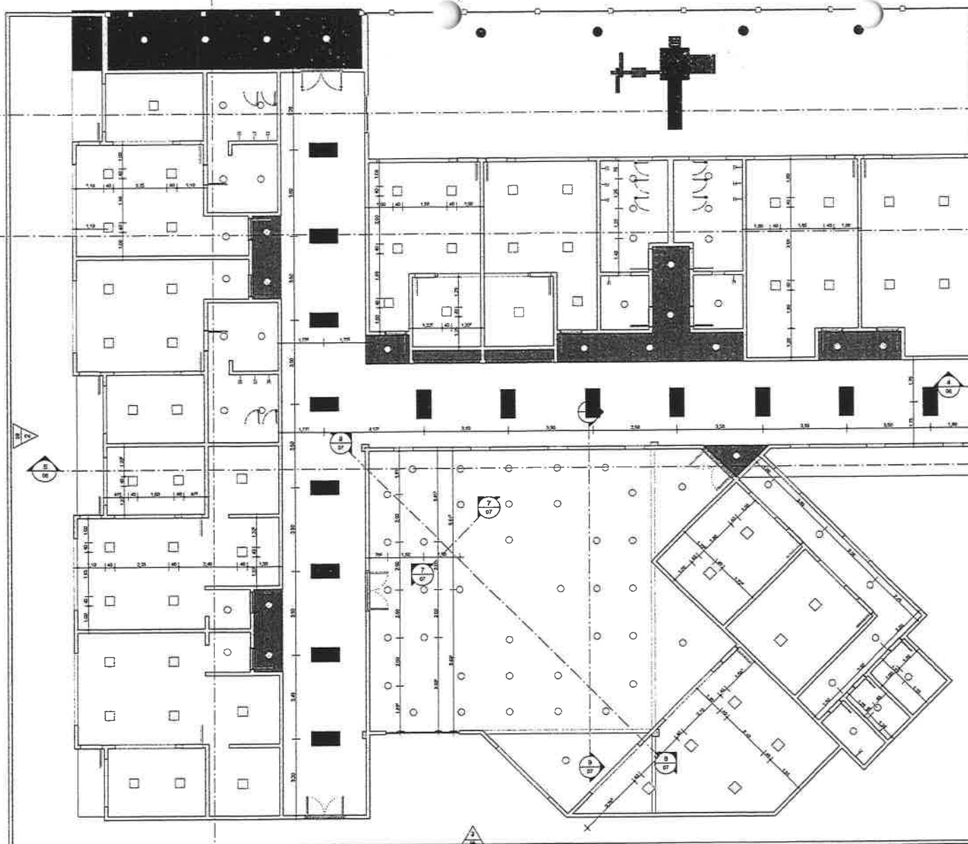
1 PLANTA DE FORRO PAV. TÉRREO 1:75
