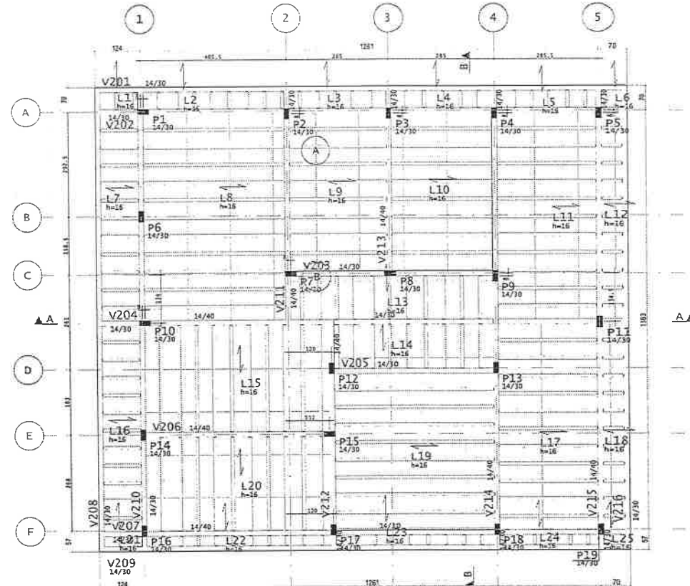
Planta de Formas - Cobertura escala 1:50
