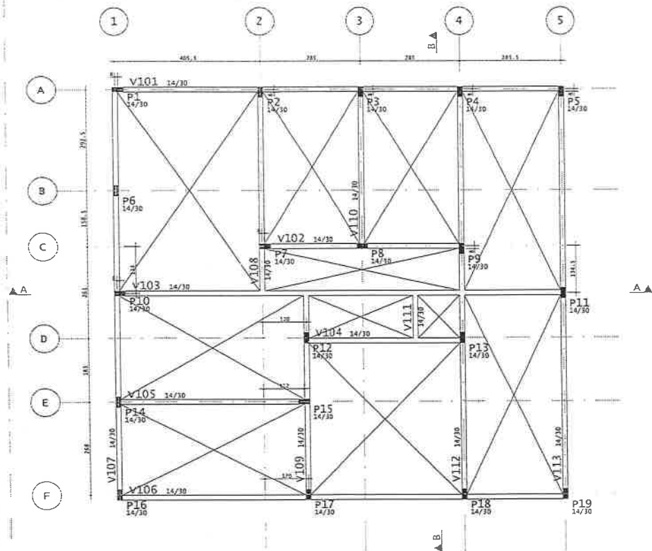
Planta de Formas - Térreo escala 1:50
