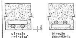
Detalhe genérico do alojamento de armaduras positivas
