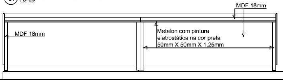
08 DET 2 - BALCÃO - VISTA TRASEIRA Esc: 1/25
