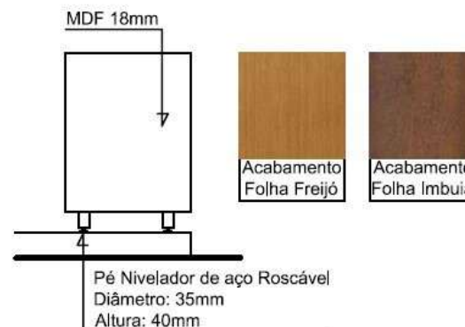
10 DET 2 - BALCÃO - VISTA LATERAL Esc: 1/25
