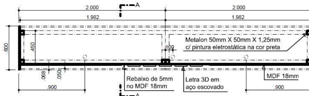
09 DET 2 - BALCÃO - PLANTA BAIXA Esc: 1/25
