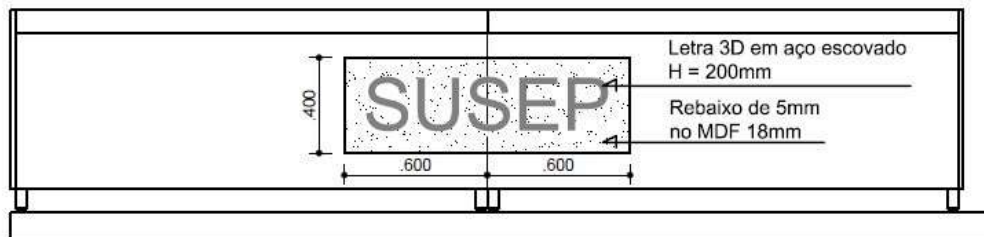
07 DET 2 - BALCÃO - VISTA FRONTAL Esc: 1/25
