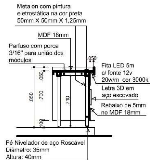
11 DET 2 - BALCÃO - CORTE AA Esc: 1/25
