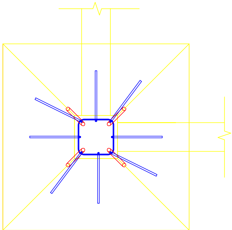
DETALHE TÍPICO DA ARMAÇÃO DOS PILARES P1 42 X
