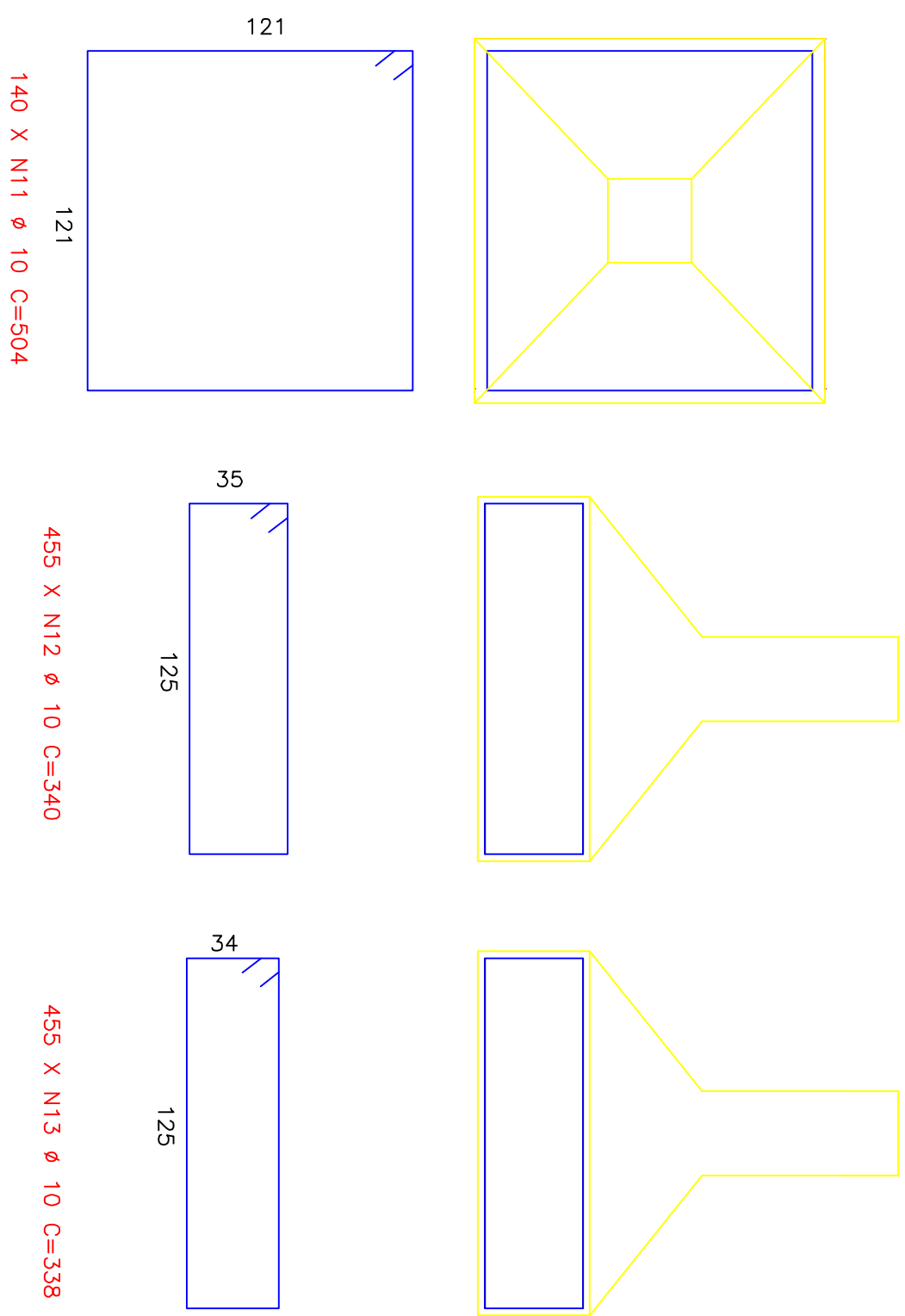
B2 (35x) DETALHE TÍPICO 130x130x40
