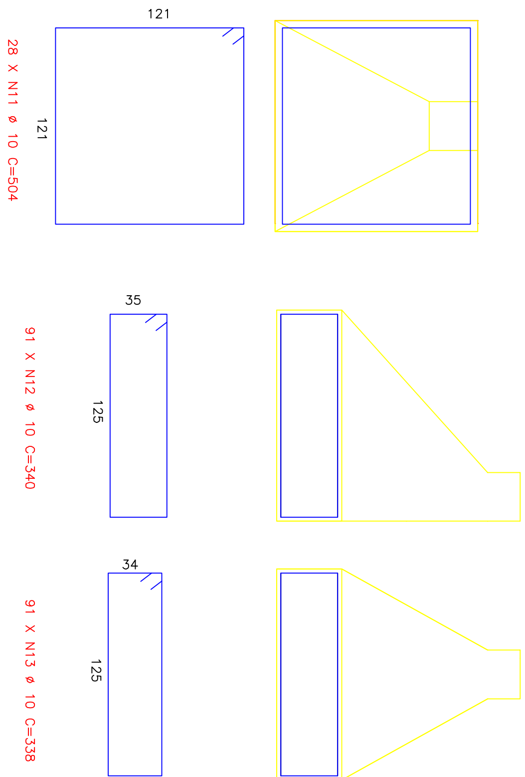
B1 (7x) DETALHE TÍPICO 130x130x40
