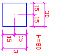
PLANTA 30x30x80 PILAR 30x30
