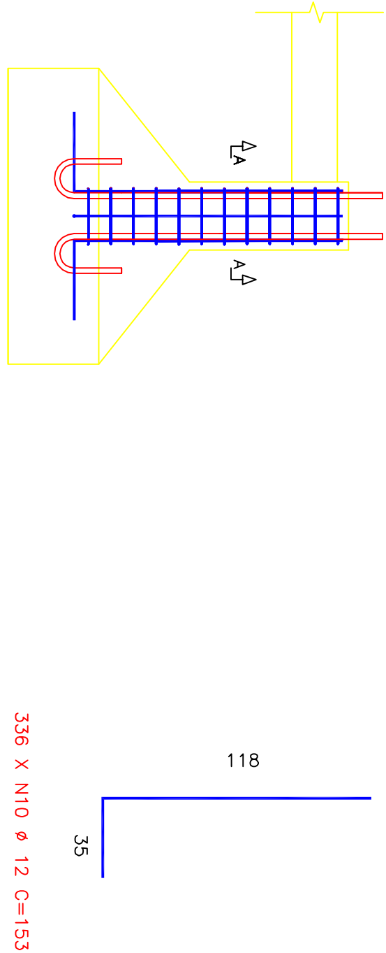
DETALHE TÍPICO DA ARMAÇÃO DOS PILARES P1 42 X
