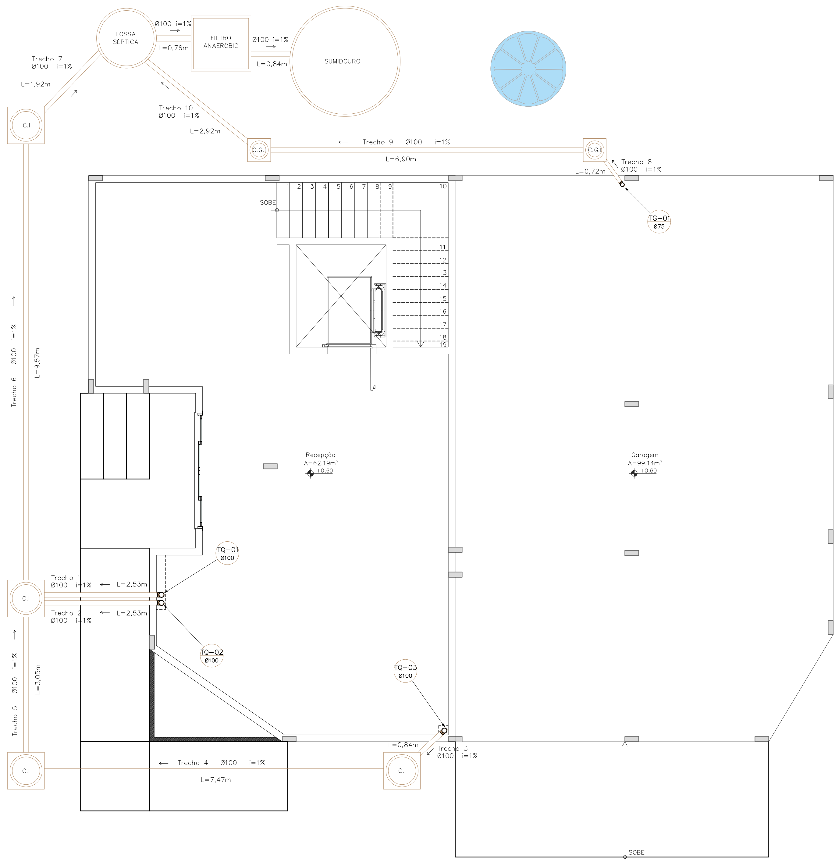
PLANTA BAIXA TÉRREO Esc. 1:50
