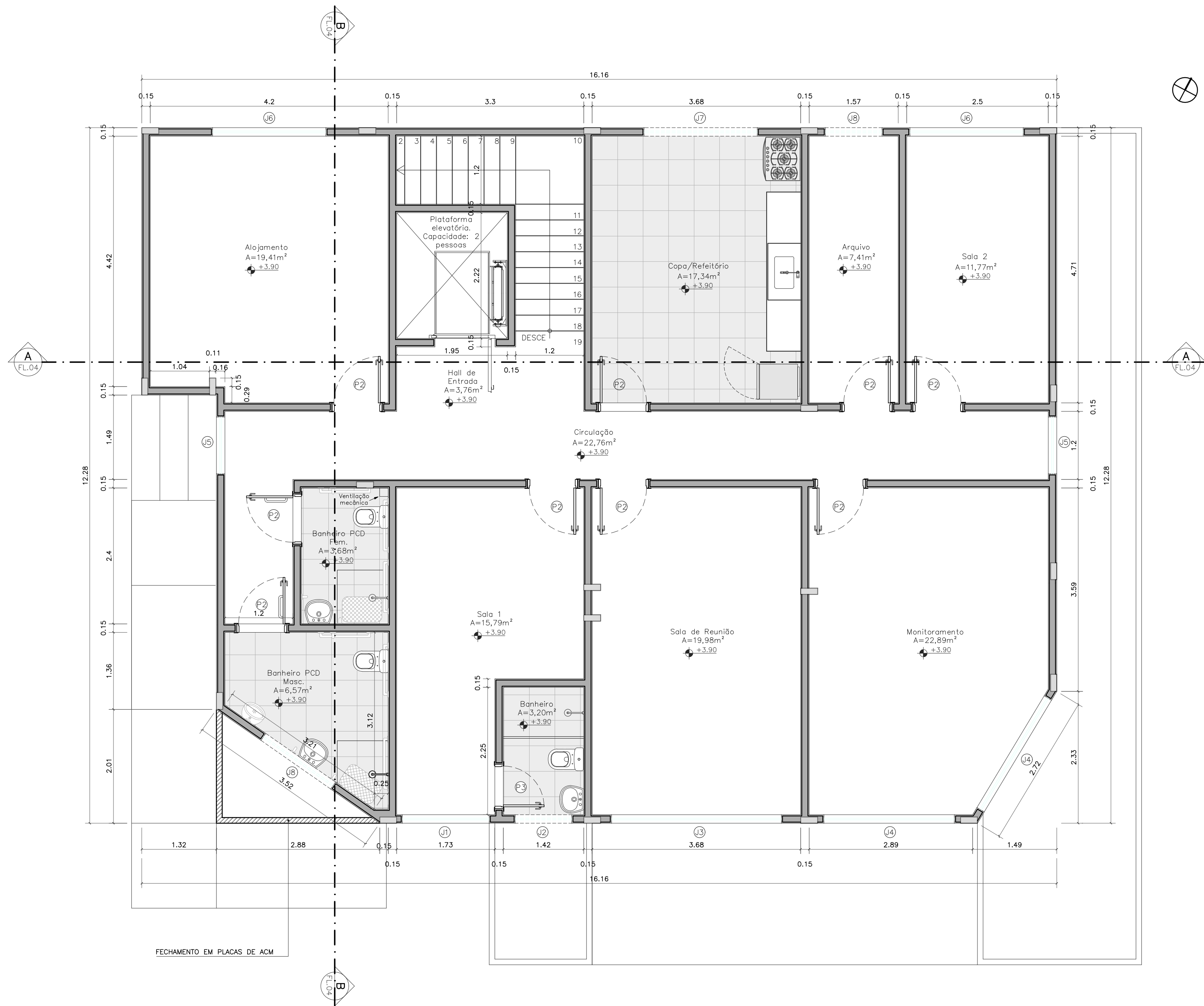
PLANTA BAIXA 1º PAVIMENTO Escala: 1:50
