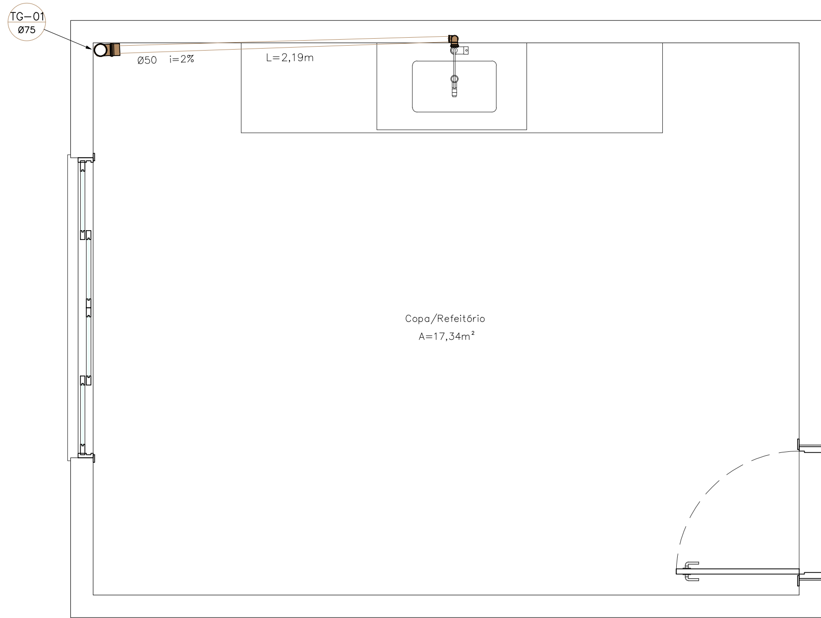
DETALHAMENTO DA COZINHA Esc. 1:25
