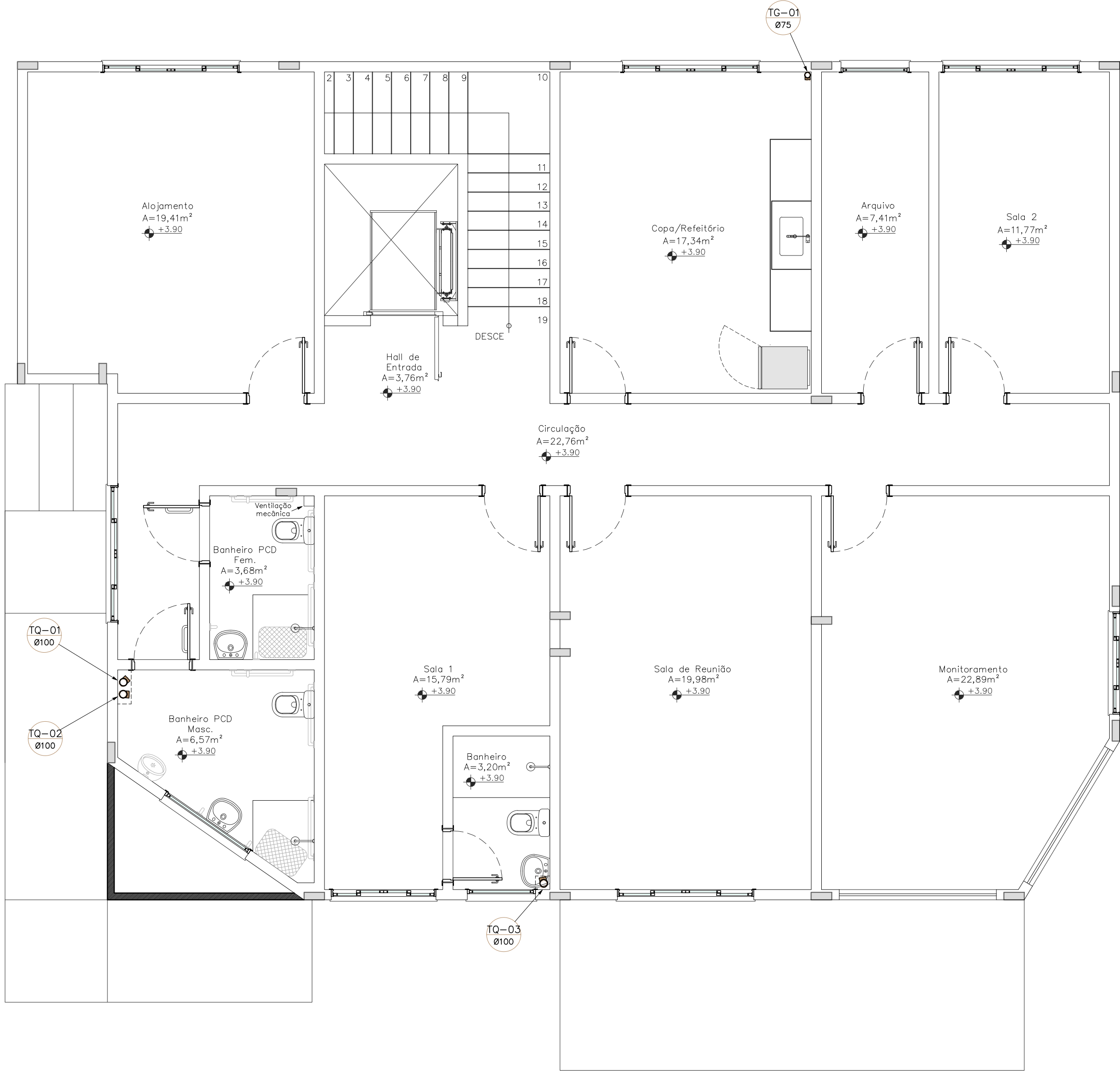
PLANTA BAIXA 1º PAVIMENTO Esc. 1:50
