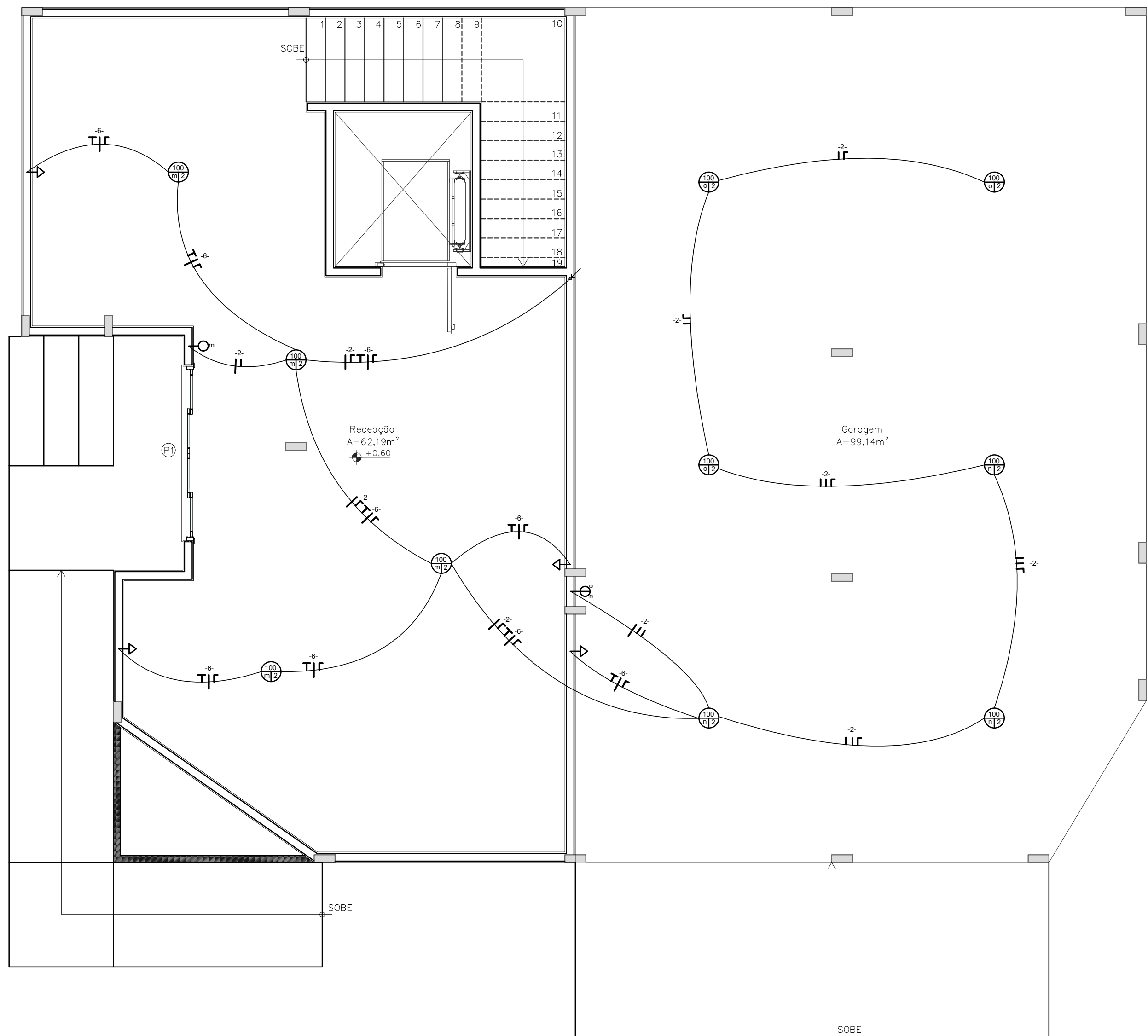
PLANTA BAIXA ELÉTRICA - TÉRREO ESC. 1:50
