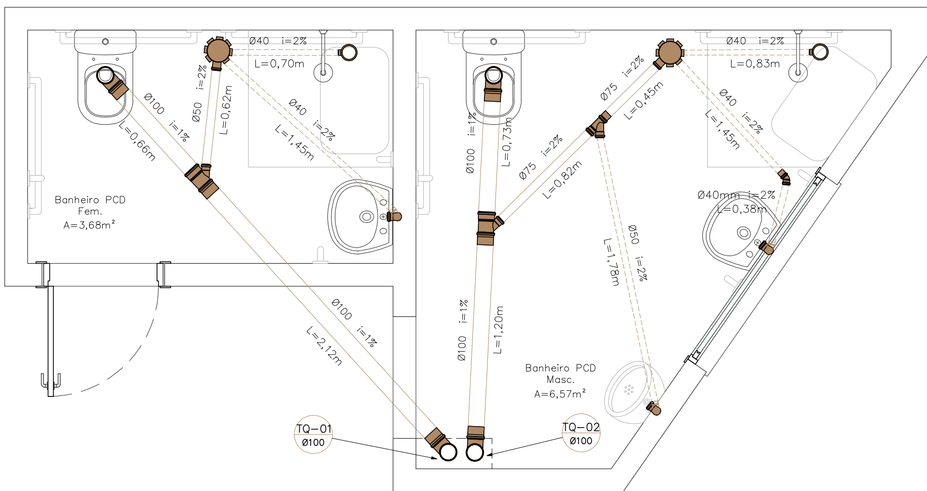
DETALHAMENTO DOS BANHEIROS FEMININO E MASCULINO Esc. 1:25
