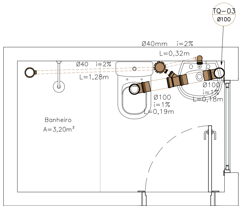
DETALHAMENTO DO BANHEIRO DA SALA 1 Esc. 1:25
