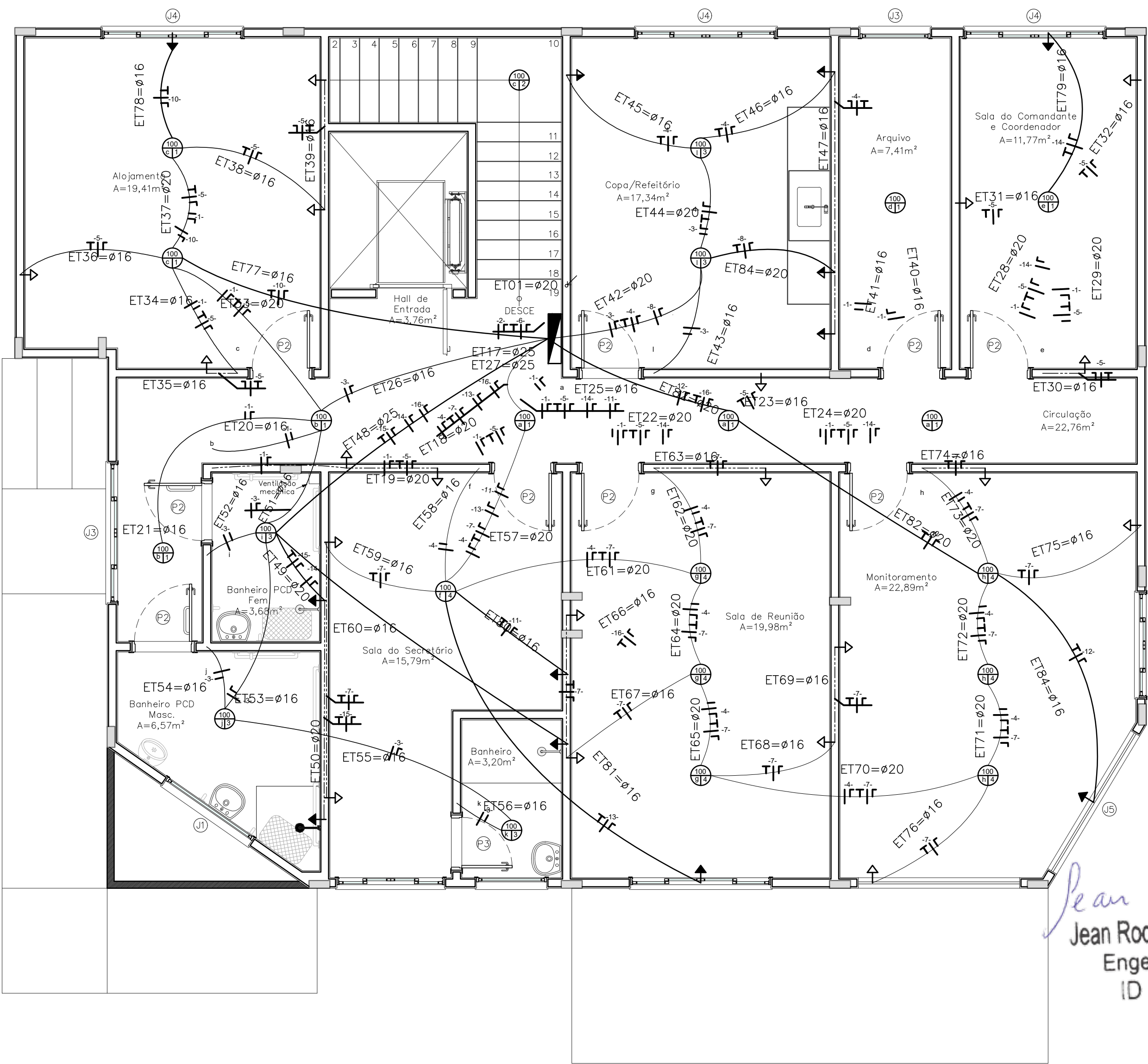
PLANTA BAIXA ELÉTRICA - 1º PAV. ESC. 1:50
