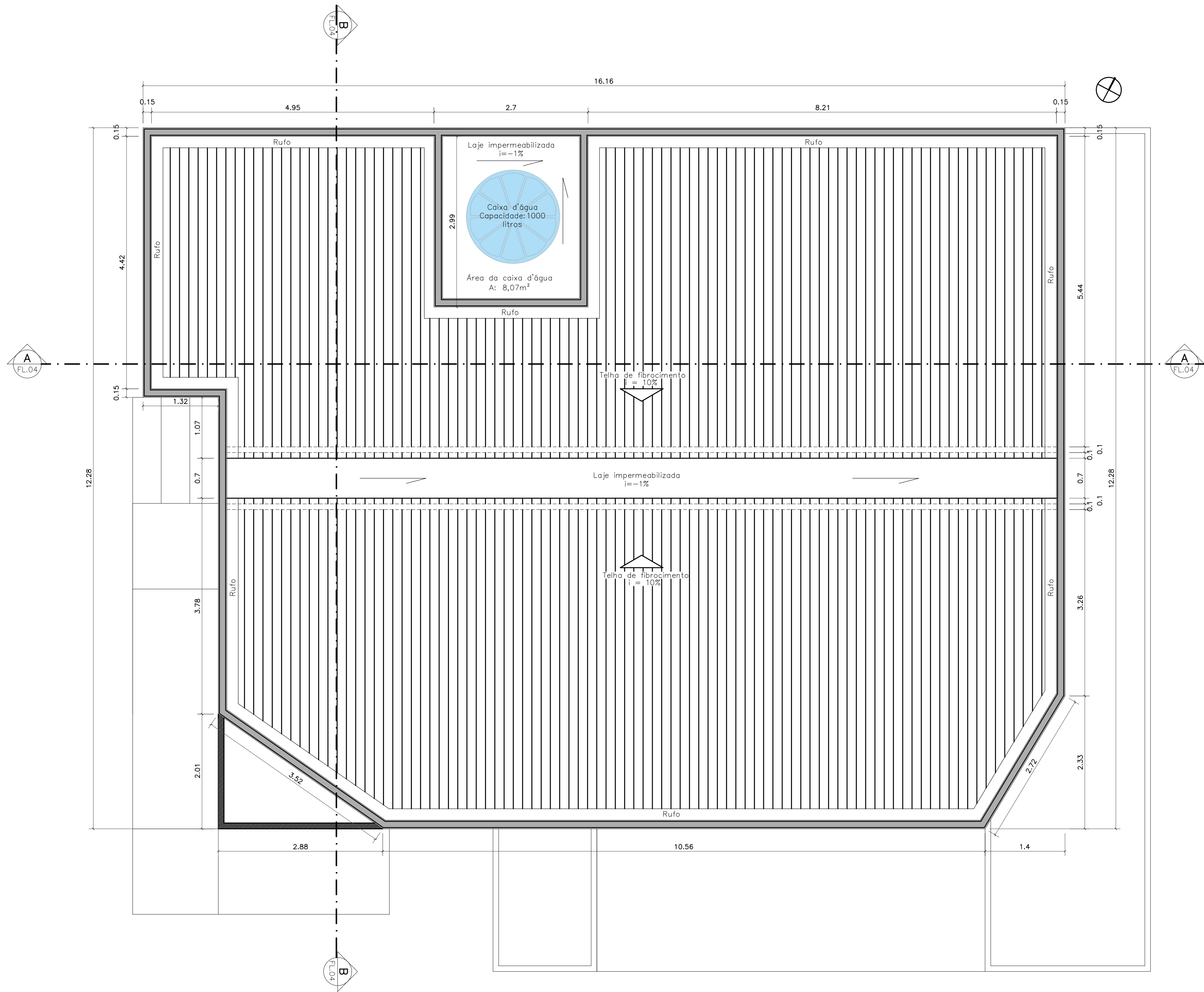
PLANTA DE COBERTURA Esc. 1:50
