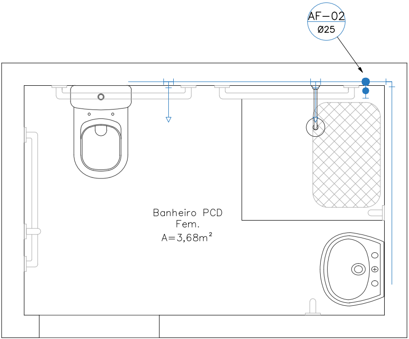
DETALHAMENTO DO BANHEIRO FEMININO Esc.: 1:25
