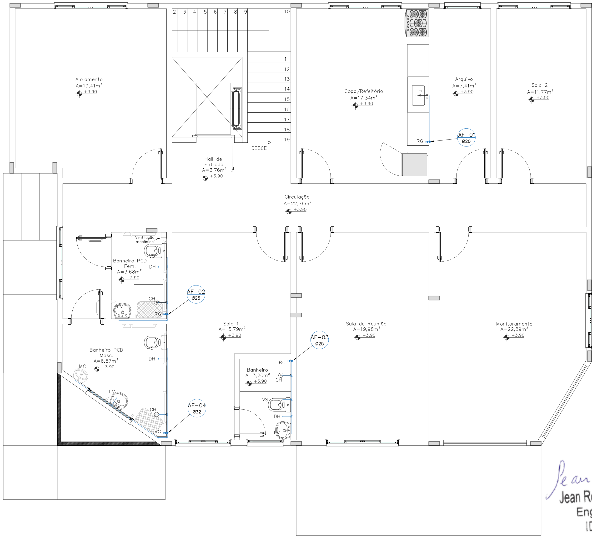
PLANTA BAIXA 1º PAVIMENTO ESC.: 1:50
