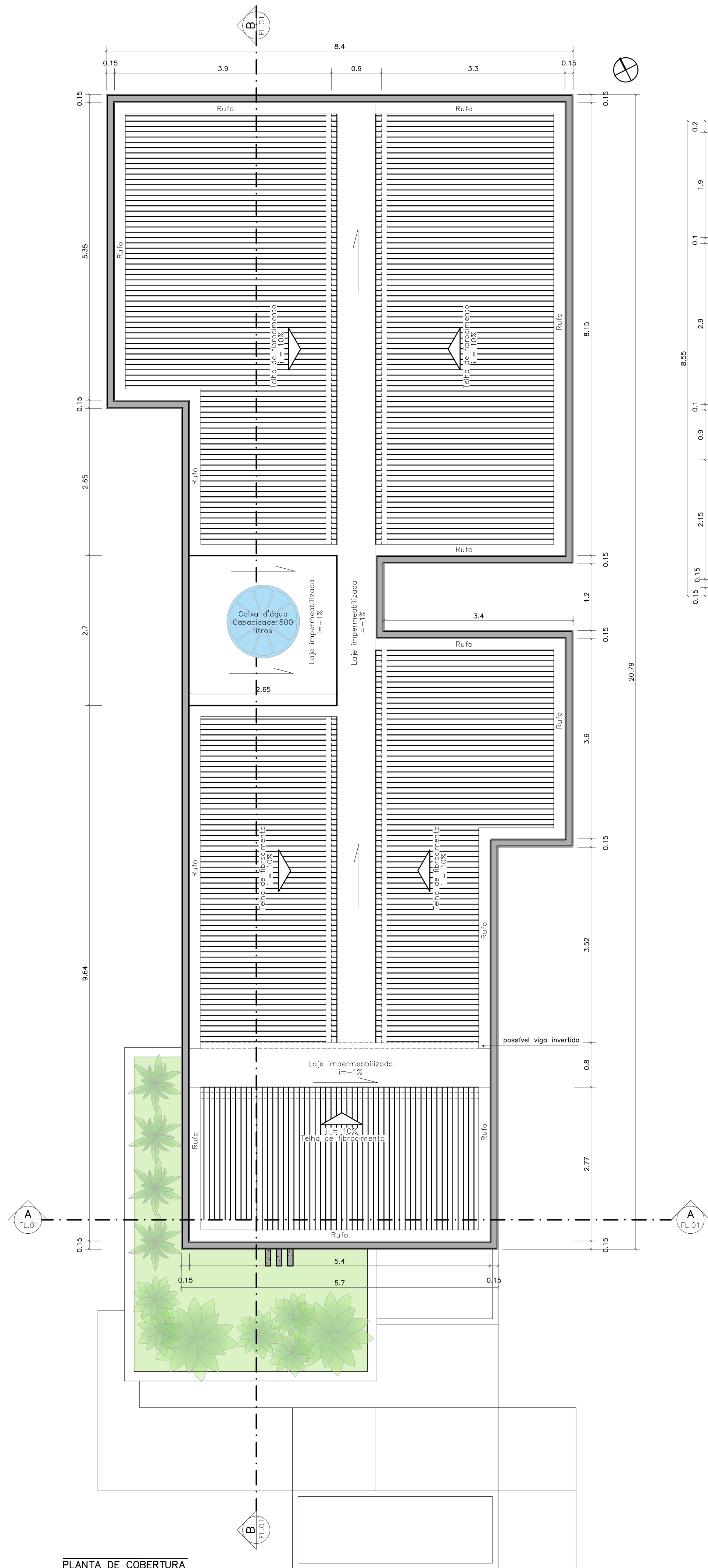
PLANTA DE COBERTURA ESC.: 1:50
