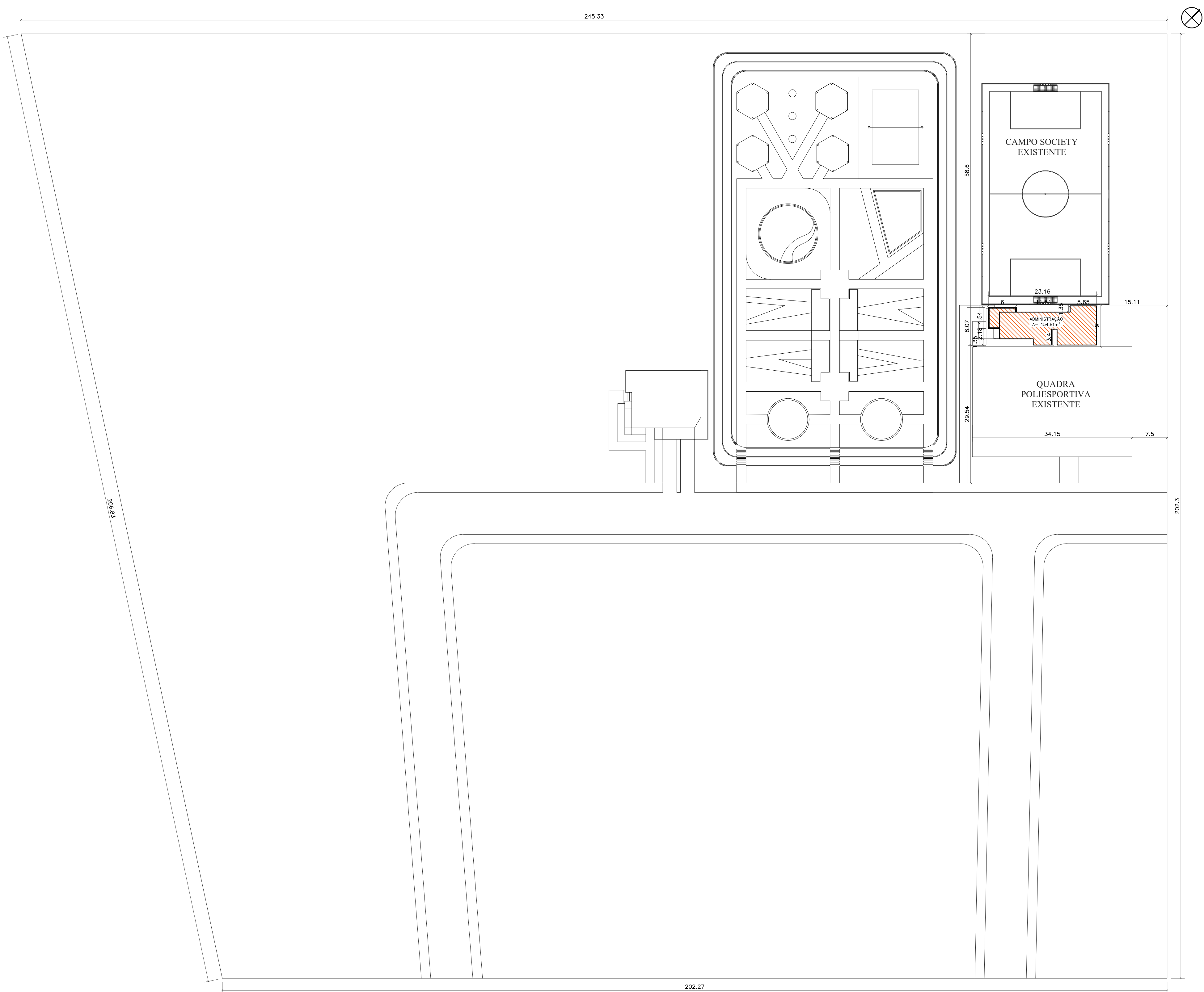
PLANTA DE IMPLANTAÇÃO ESC.: 1:500
