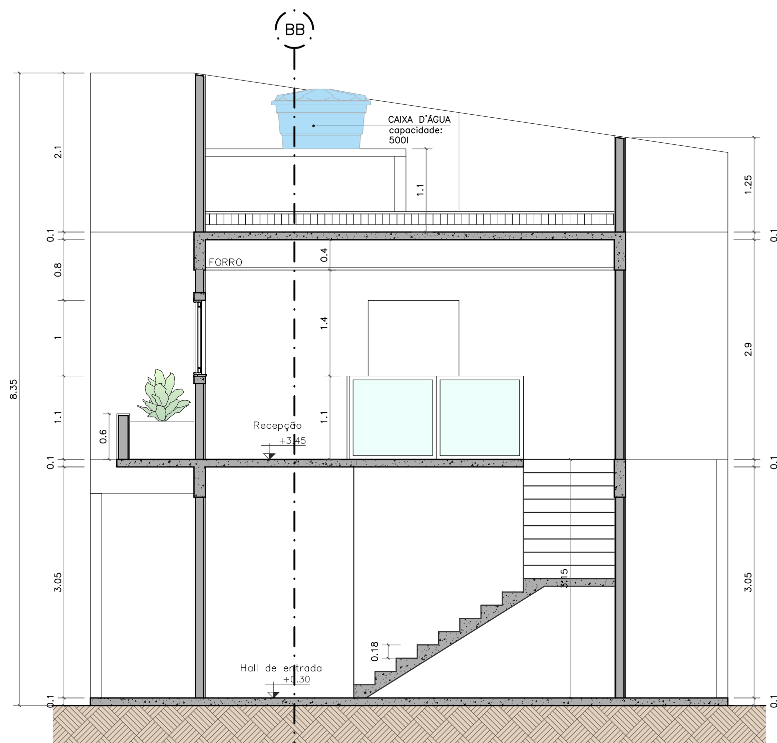
CORTE AA ESC.: 1:50
