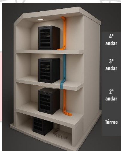
Imagem 2 - Distribuição em rack por pavimento SW CORE para os SW de distribuição
