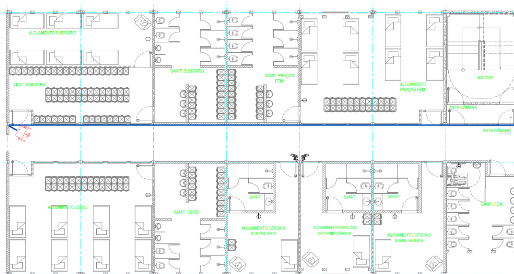
Imagem 9 – Distribuição dos pontos no 3º pavimento lado direito da entrada pela recepção
