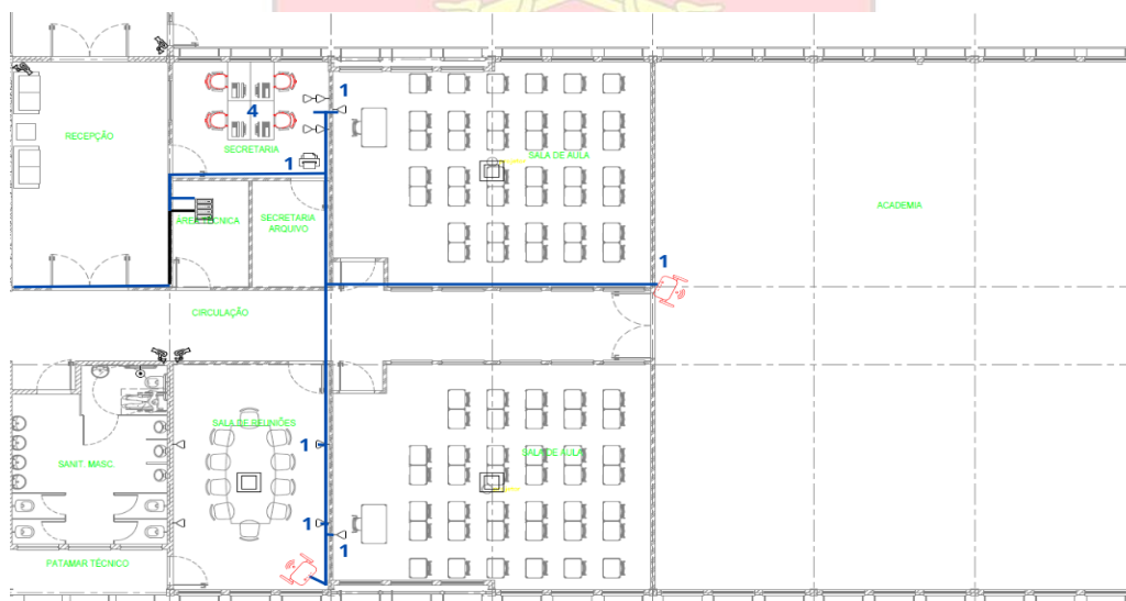
Imagem 10 – Distribuição dos pontos no 4º pavimento lado esquerdo da entrada pela recepção
