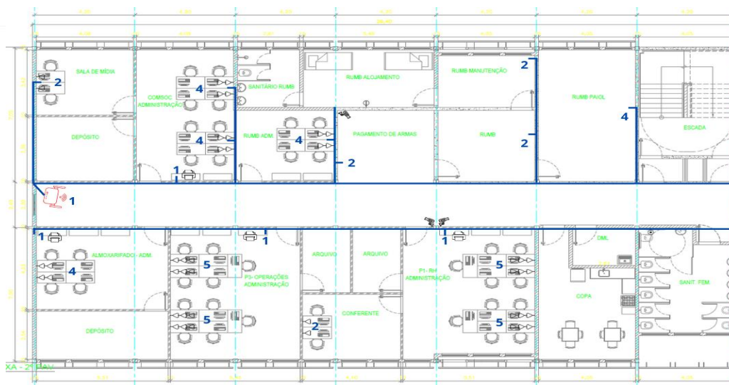
Imagem 7 – Distribuição dos pontos no 2º pavimento lado direito da entrada pela recepção
