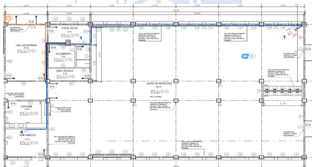
Imagem 4 - Distribuição dos pontos no térreo lado esquerdo do Hall de Entrada
