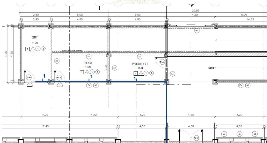
Imagem 3 – Distribuição dos pontos no Prédio anexo
