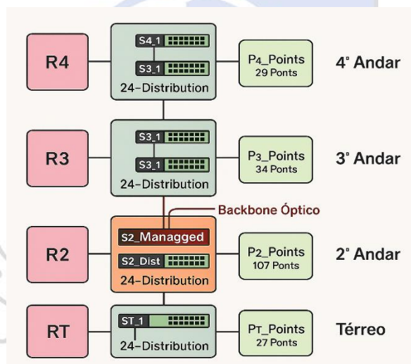
Imagem 1 - Distribuição do entroncamento em fibra do SW CORE para os SW de distribuição
