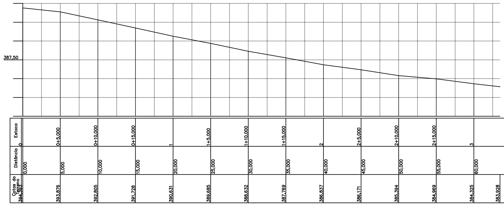
PERFIL LONGITUDINAL ESCALA: h=1:250 v=1:250
