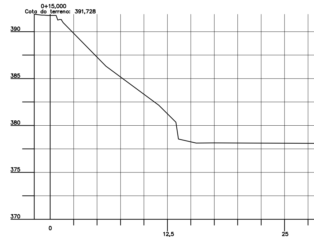
SEÇÕES TRANSVERSAIS ESCALA: 1:250
