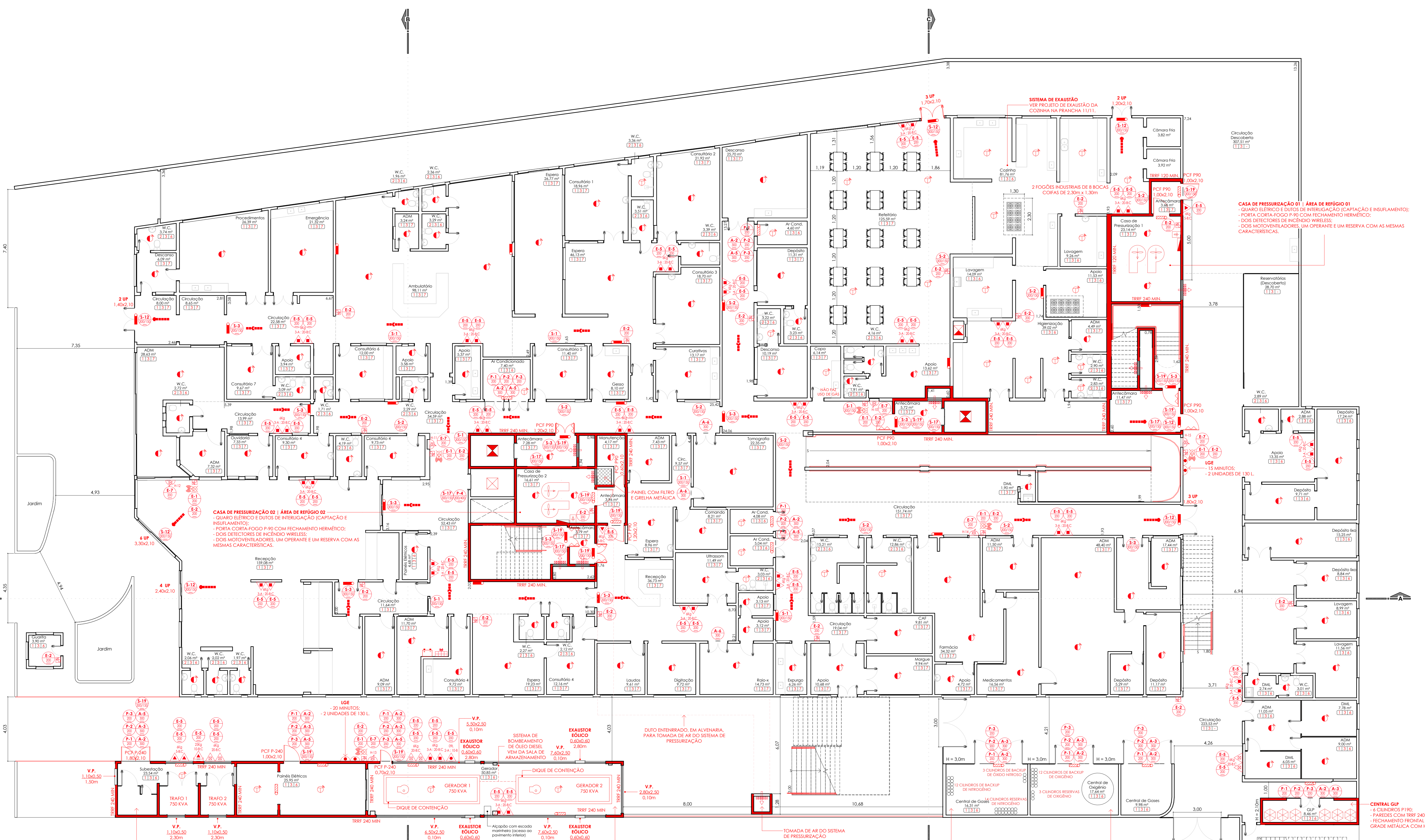
PAVIMENTO TÉRREO ESC: 1 : 100
