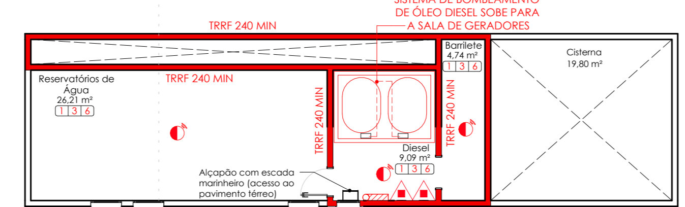
PAVIMENTO INFERIOR ESC: 1 : 100
