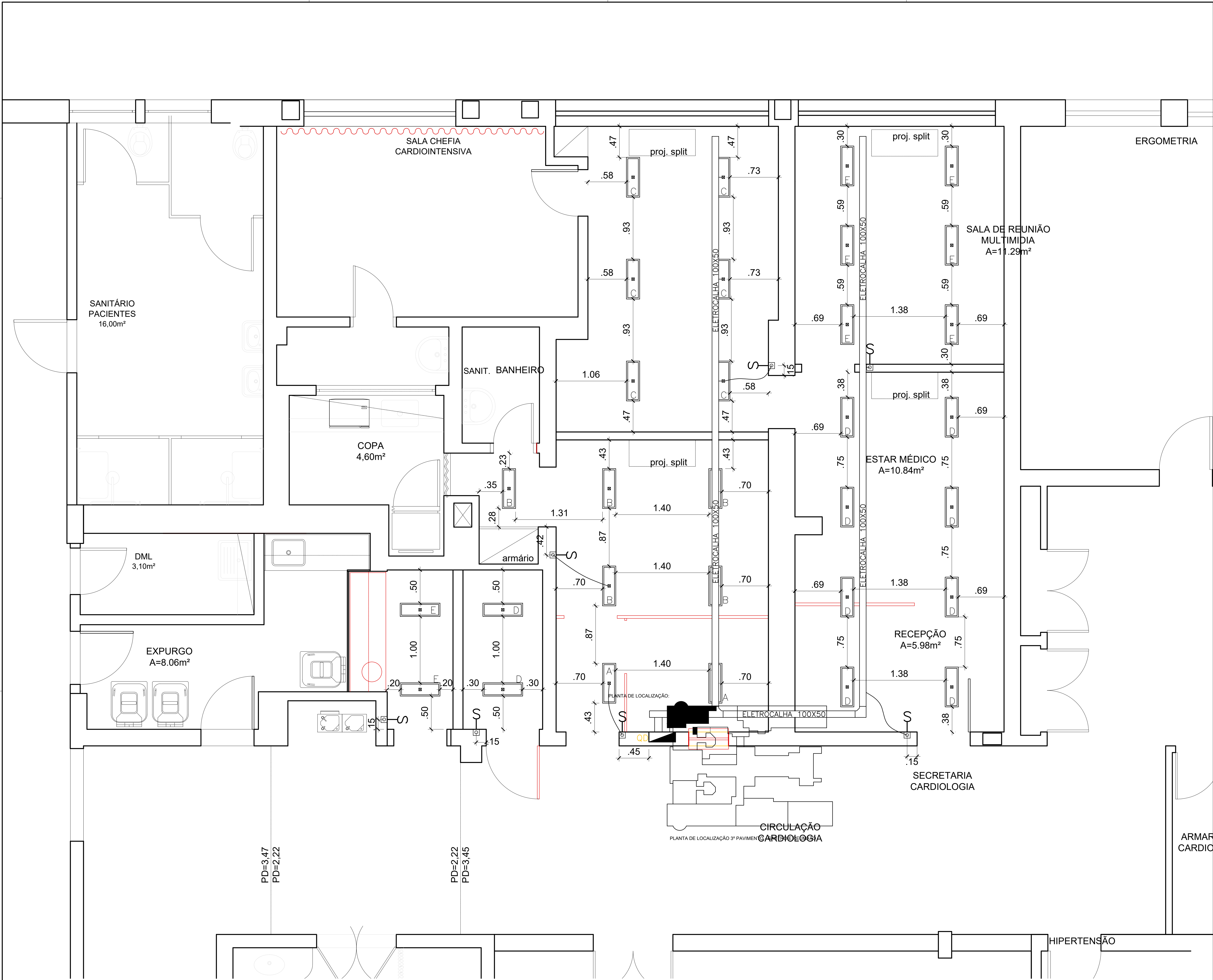
01 PALNTA BAIXA - ELÉTRICA ESCALA: 1/25
