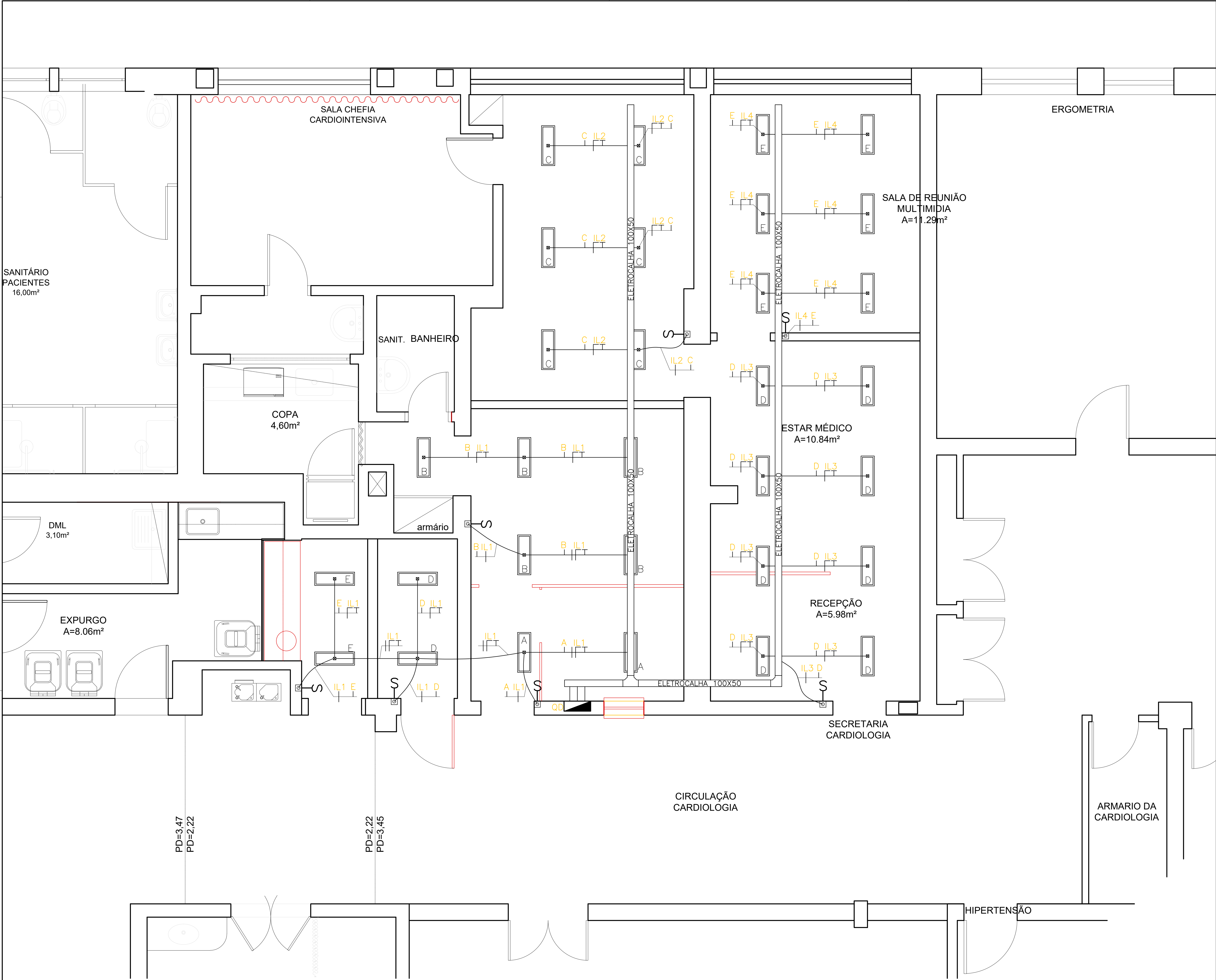
01 PLANTA BAIXA - ELÉTRICA ESCALA: 1/25
