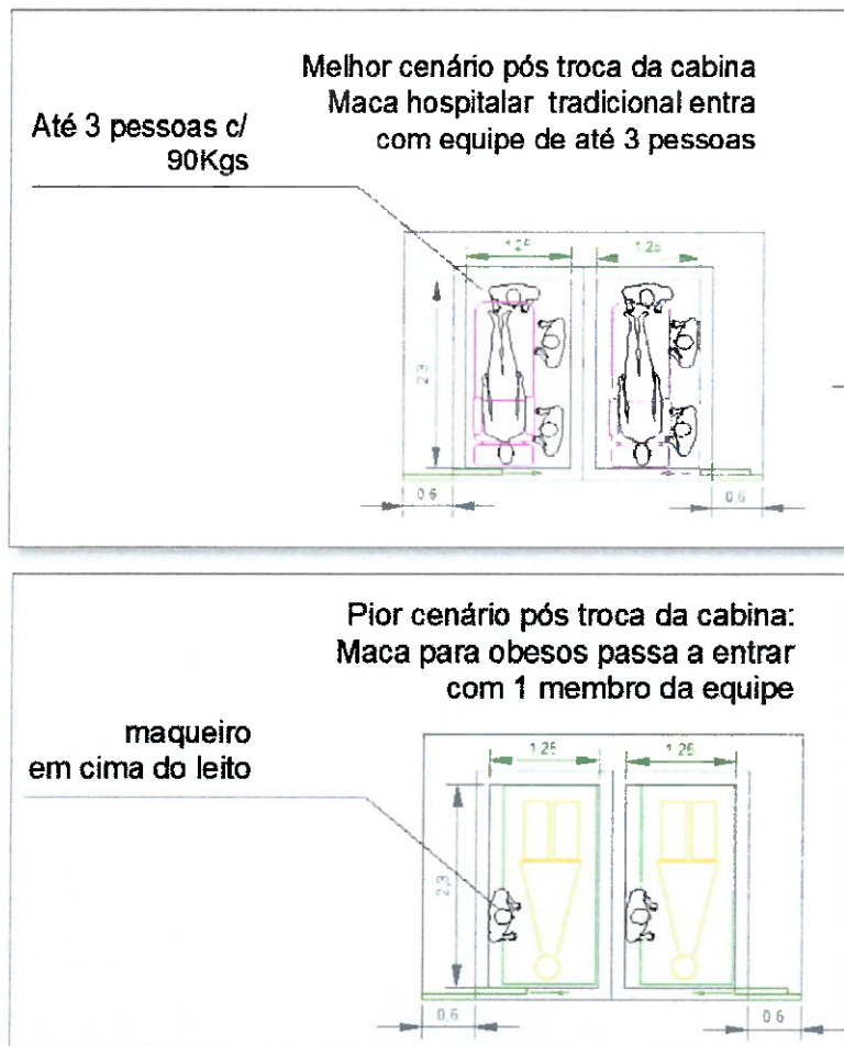
Figura 04 a) e b)– Elevadores do grupo 2 com a cabina trocada (cenários de operação)
