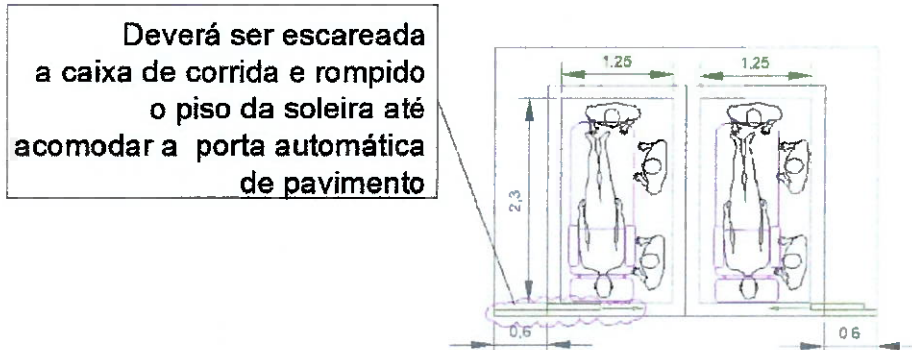
Figura 05: Instalação das novas porta de pavimento com a nova cabina
