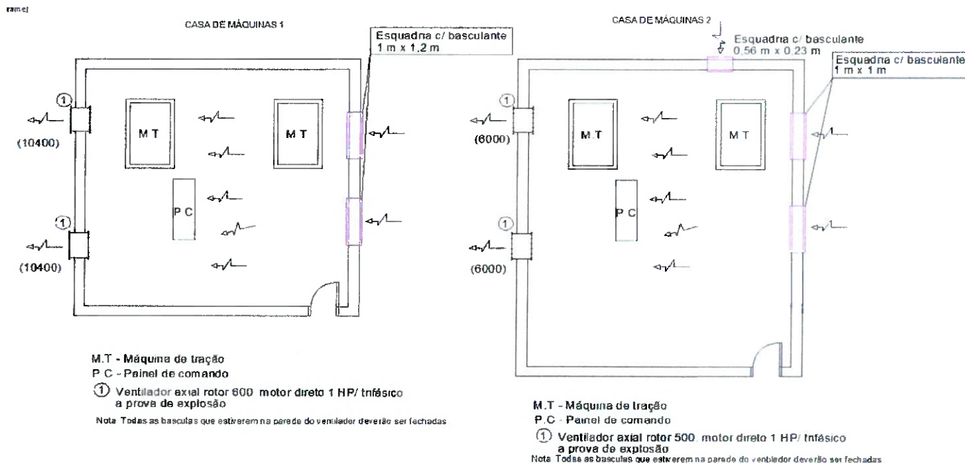
Figura 08: Solução de ventilação cruzada
