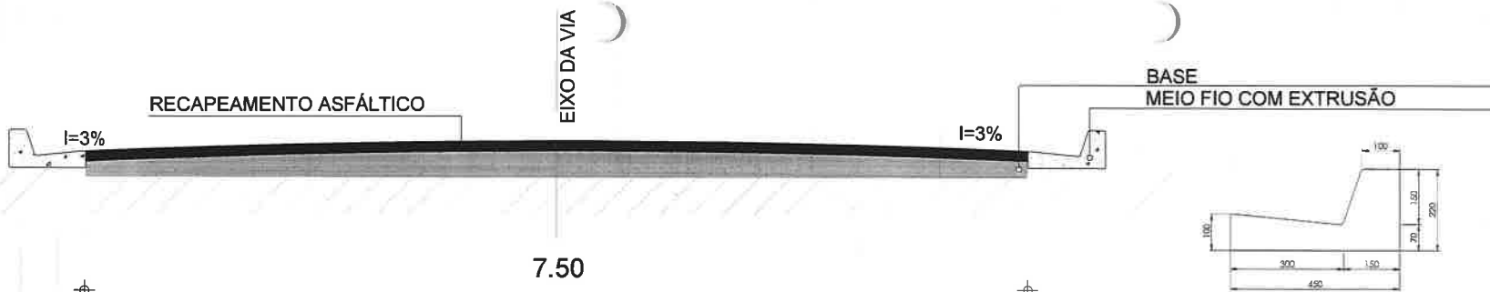
01 DET. SEÇÃO DA VIA - TIPO 1 ESCALA S/E
