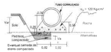
Detalhe do bargo sobre solo ou rocha
