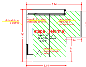
4 PLANTA GUARITA ESC. 1:175
