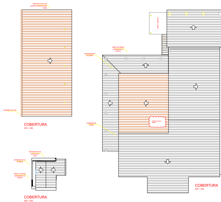
6 PLANTA DE TELHADO ESC. 1:175
