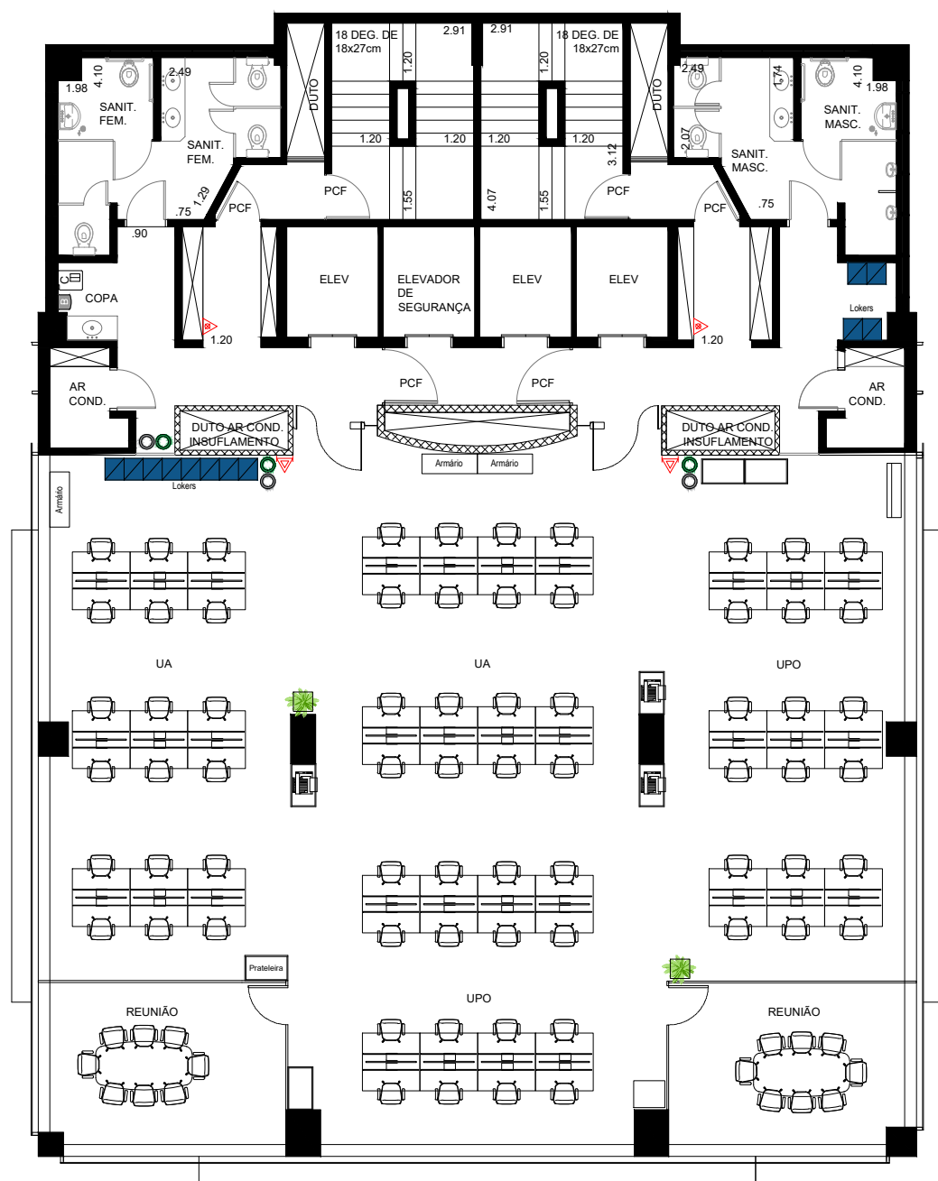
PLANTA DO 9º PAVIMENTO Layout existente
