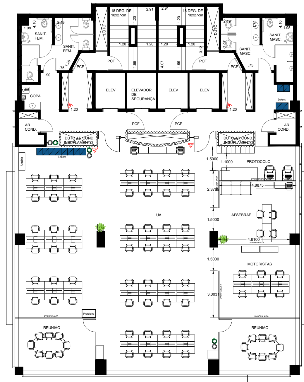
PLANTA DO 9º PAVIMENTO Layout proposto JUL/2026
