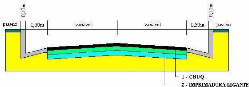
Figura 2 - Corte típico de recapeamento
