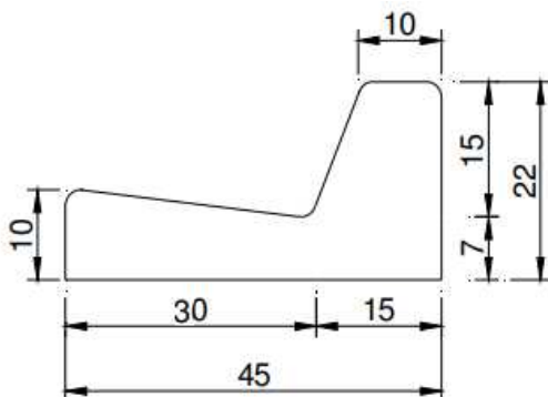
Figura 1 - Corte Típico
