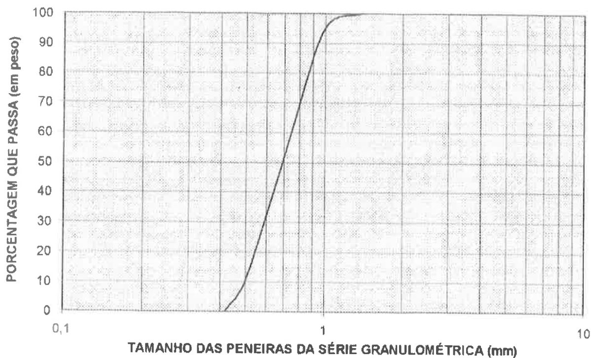
Figura 2 - Curva granulométrica da Areia
