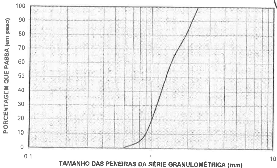
Figura 1 - Curva granulométrica do Antracito
