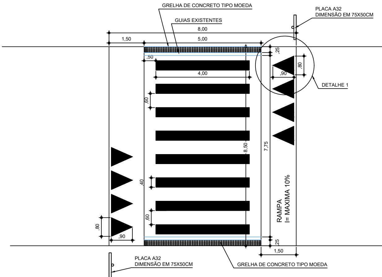
FAIXA ELEVADA - PLANTA ESC. 1:100
