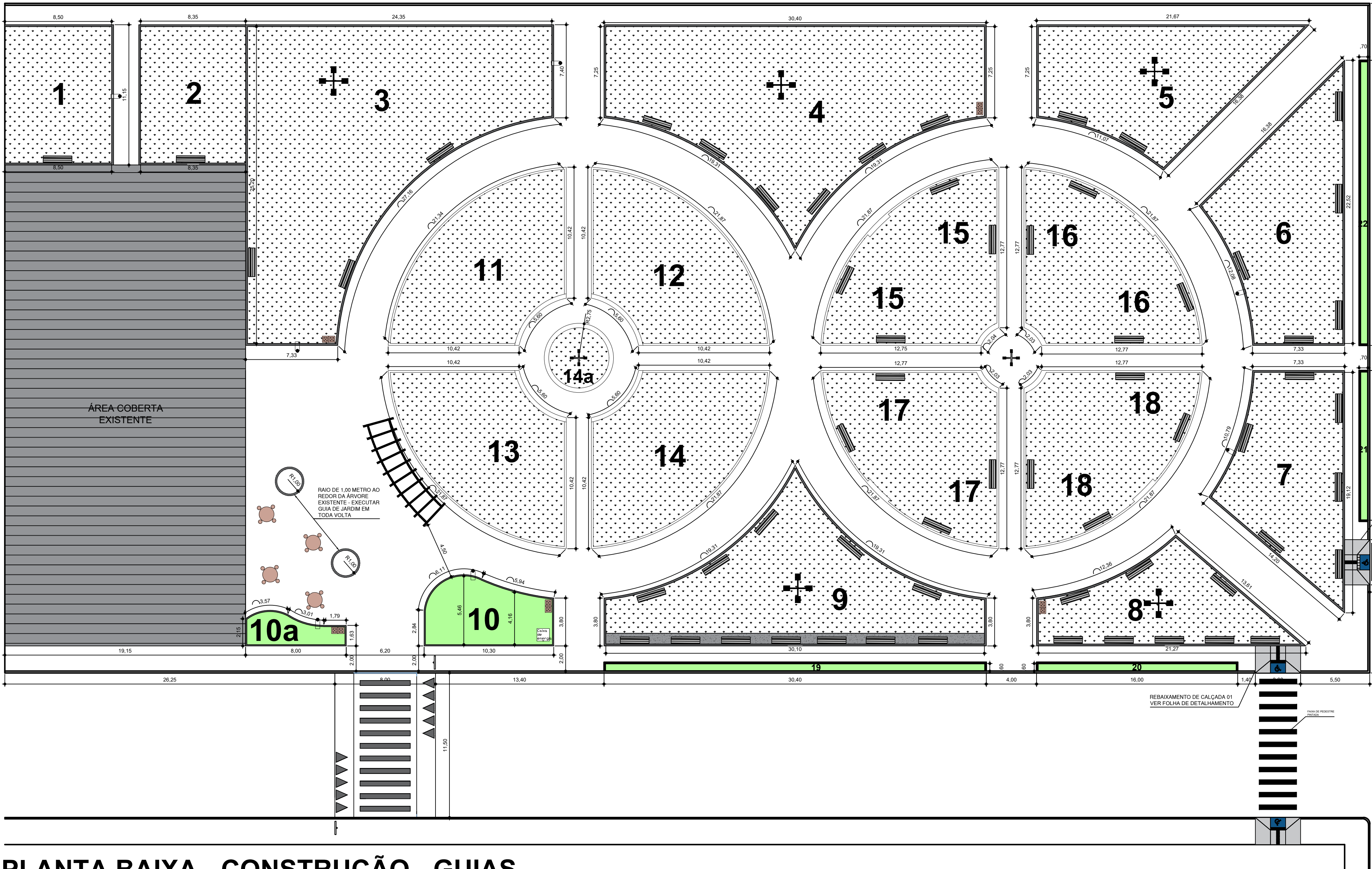
PLANTA BAIXA - CONSTRUÇÃO - GUIAS ESCALA 1:200
