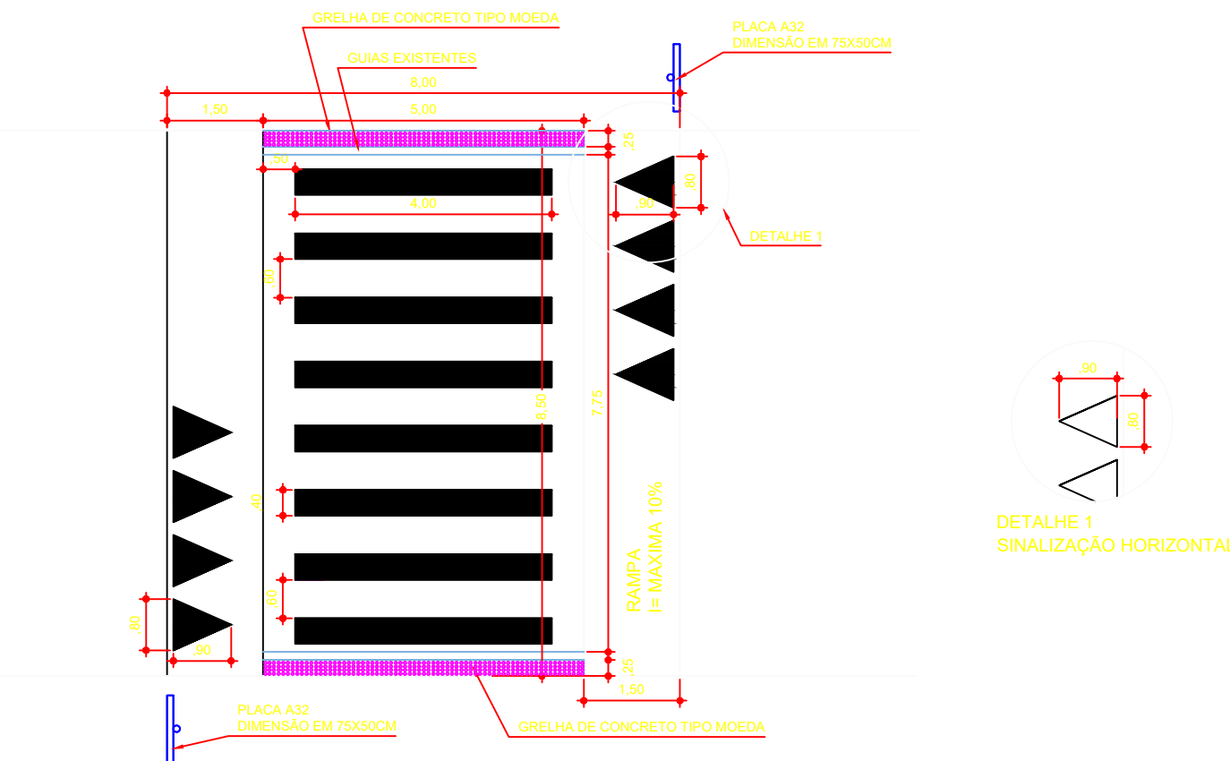
FAIXA ELEVADA - PLANTA ESC. 1:100
