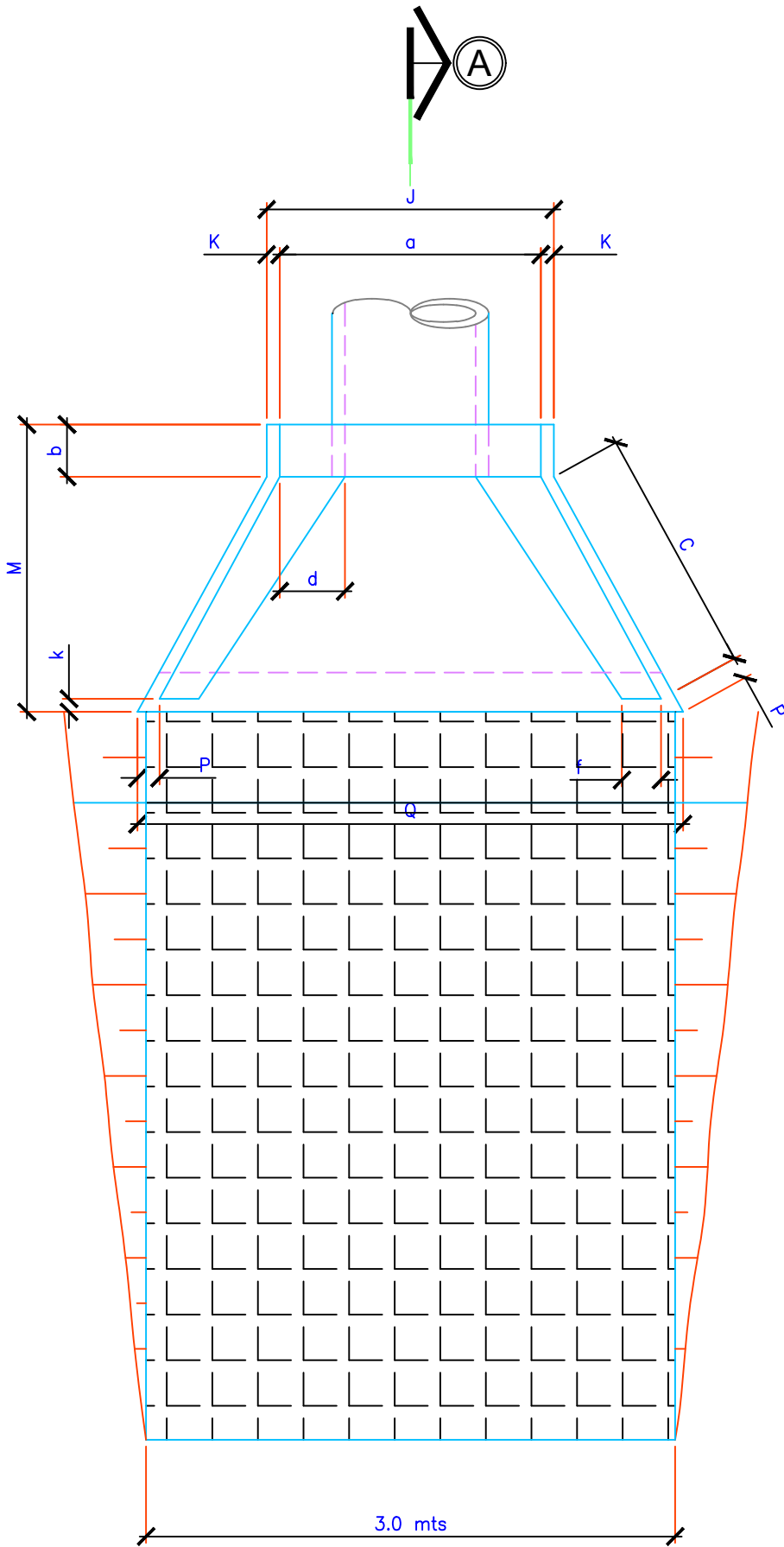
Planta ESCALA 1 : 50
