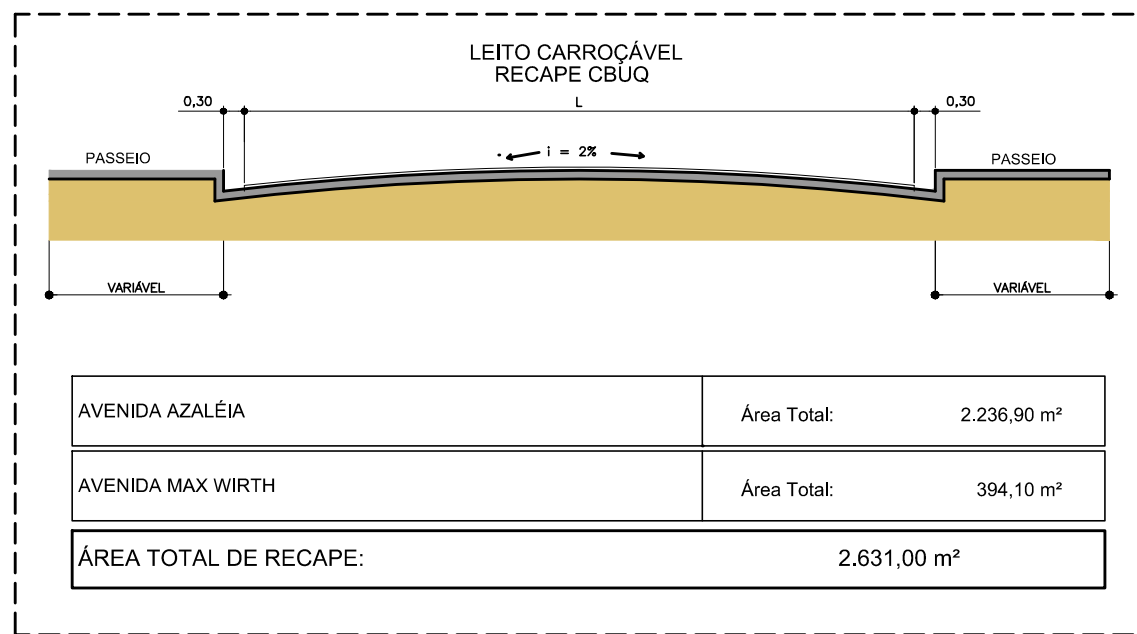
SECÇÃO TRANSVERSAL TÍPICA - RELAÇÃO DE RUAS E ÁREAS S/ESC.
