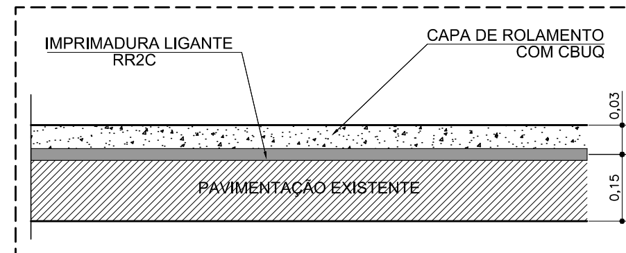
DETALHE - TÍPICO PERFIL DE RECAPEAMENTO EM CBUQ S/ESC.
