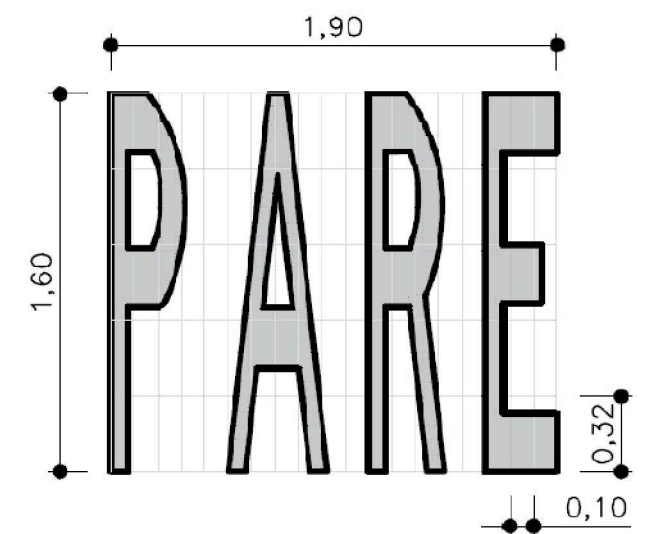
DETALHE TÍPICO - PARE SINALIZAÇÃO HORIZONTAL S/ESC.
