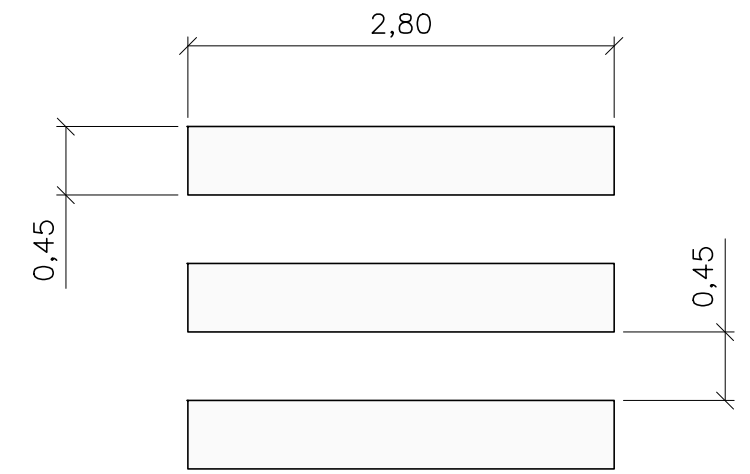
DETALHE TÍPICO FAIXAS DE PEDESTRE S/ESC.
