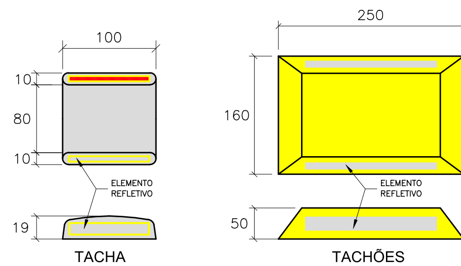
DETALHE - TACHÕES S/ESC. MEDIDAS EM mm.
