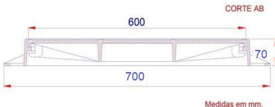
Figura 1. Layout com medidas MÍNIMAS.
