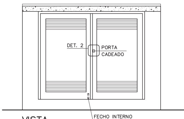
VISTA ESC. 1: 20
