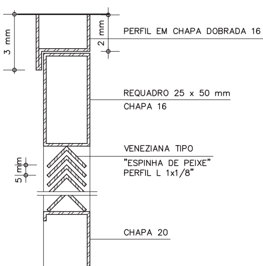
DETALHE 1 ESC. 1: 2
