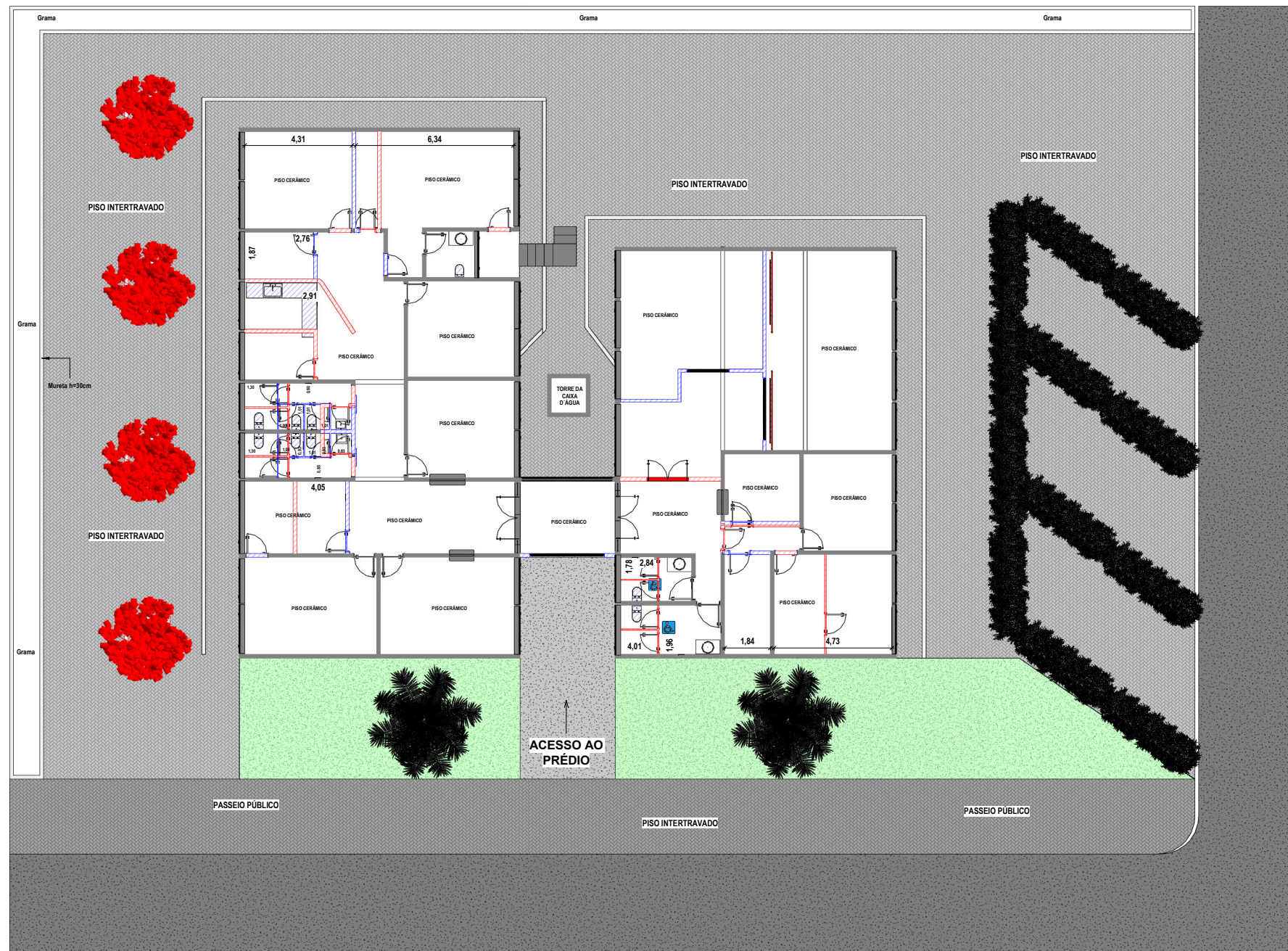
2 PLANTA BAIXA - REFORMA 1 : 100
