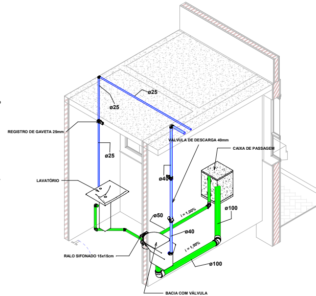
2 VISTA ISOMÉTRICA - BANHEIRO GABINETE
