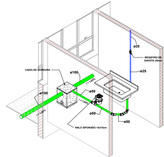
3 VISTA ISOMÉTRICA - COZINHA
