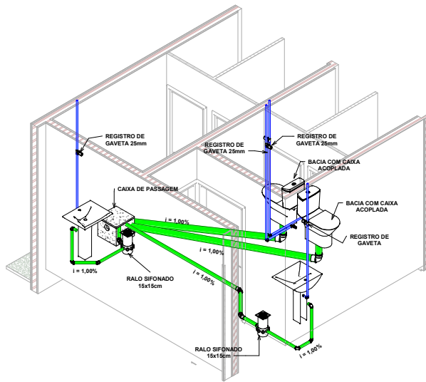
4 VISTA ISOMÉTRICA - BANHEIRO PCD
