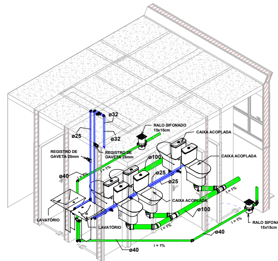
2 VISTA ISOMÉTRICA - BANHEIRO GABINETE
