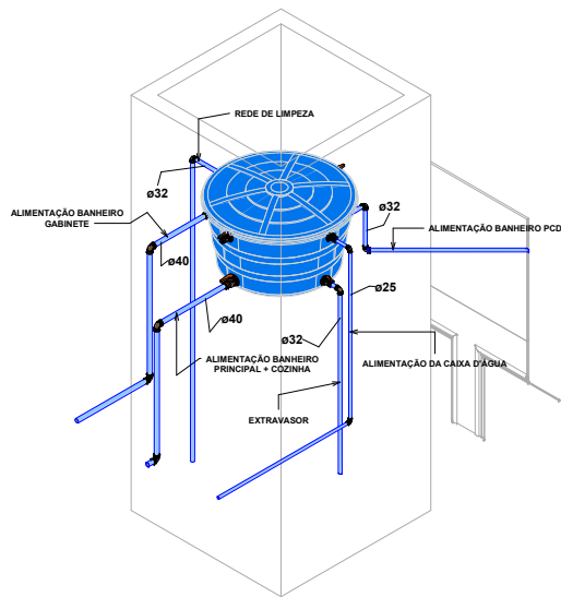
1 ISOMÉTRICO DA CAIXA D'ÁGUA
