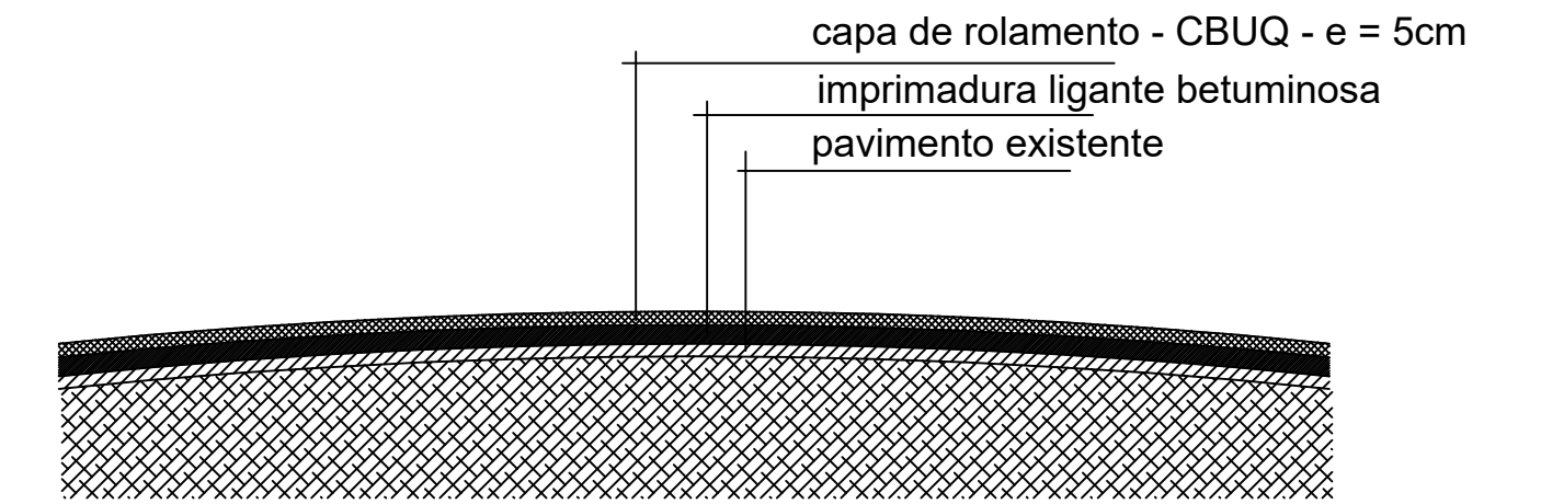
SEÇÃO TRANSVERSAL - DETALHES DAS CAMADAS
