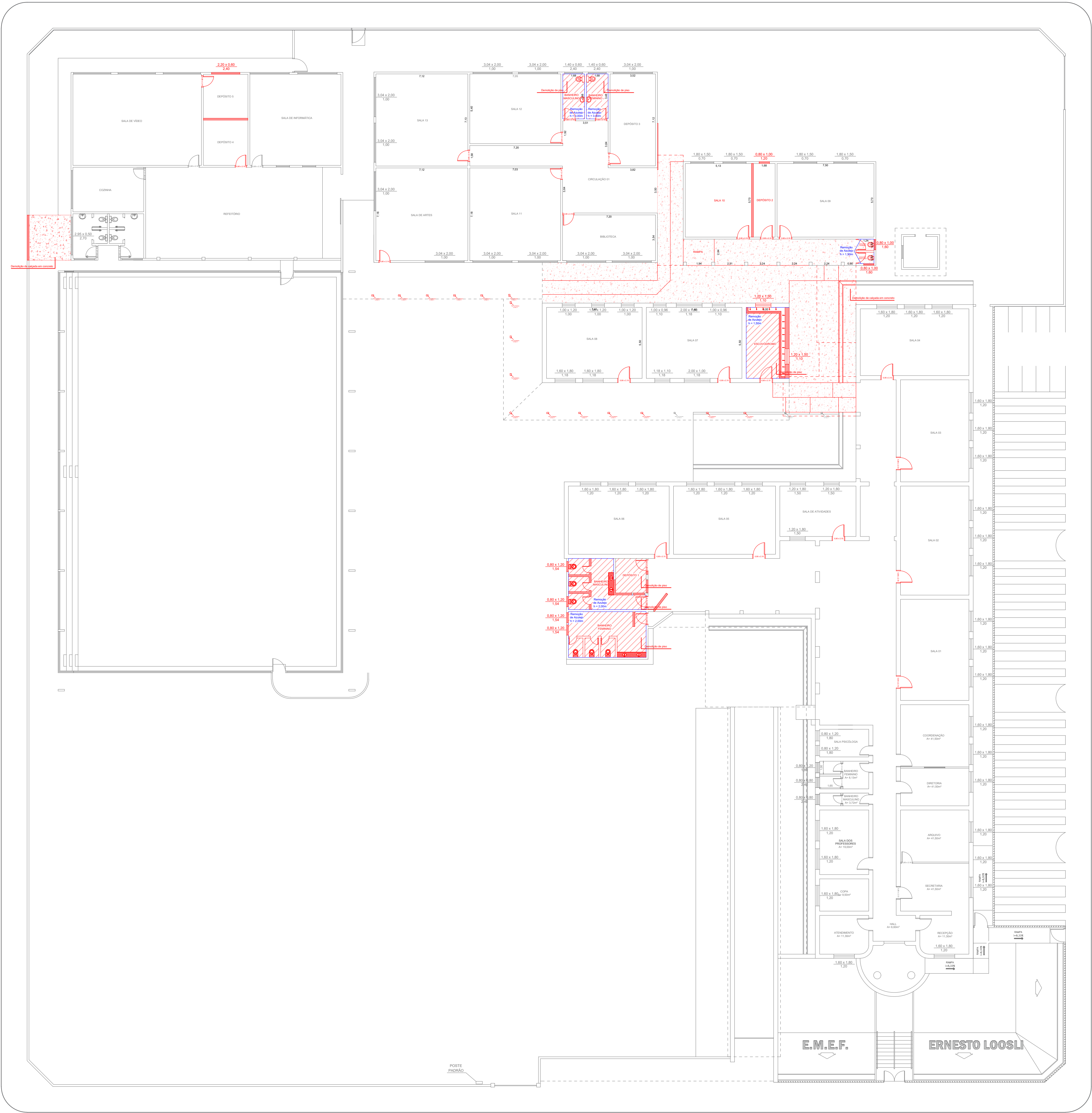
PLANTA BAIXA - DEMOLIR ESCALA 1:175
