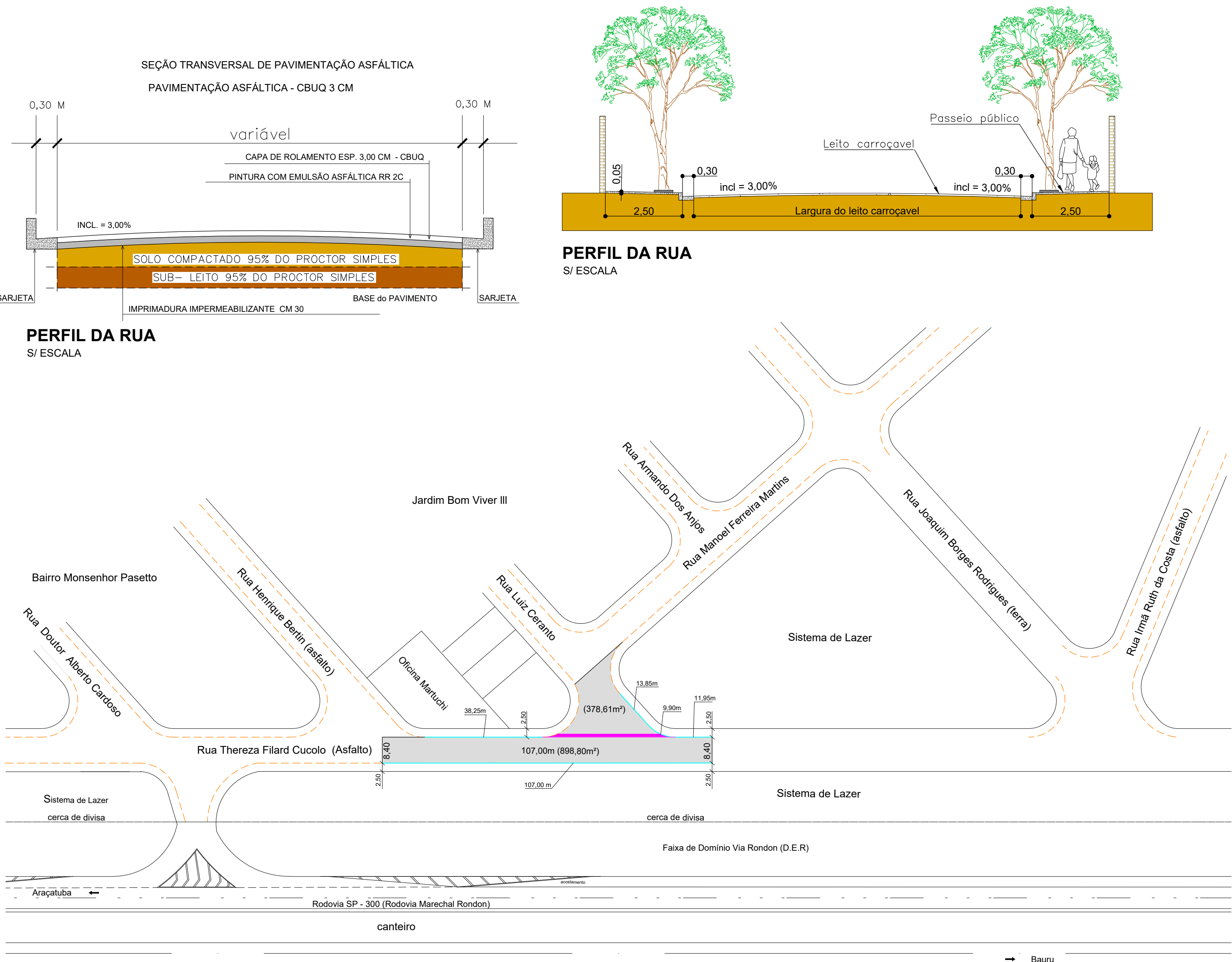
Pavimentação Asfáltica - CBUQ 3 cm Rua Thereza Filard Cucolo e Luiz Ceranto ESC. = 1:1000
