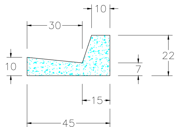
DETALHAMENTO - GUIAS E SARJETAS S/ESC
