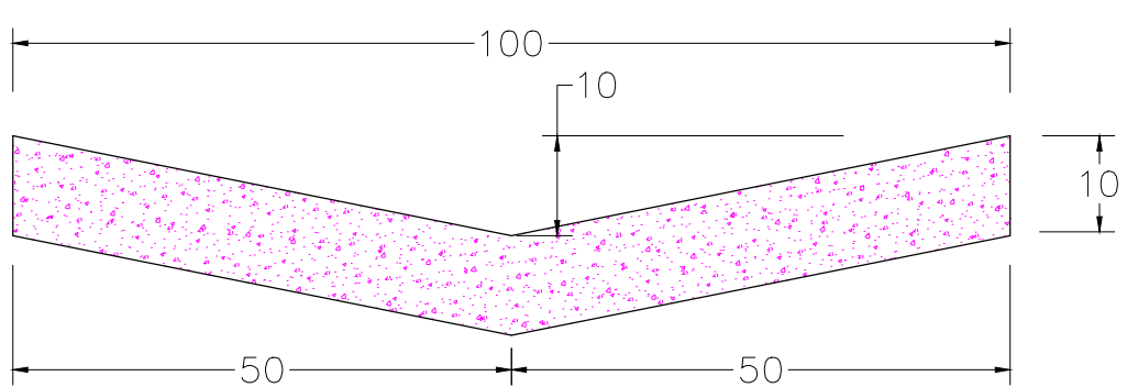
DETALHAMENTO - SARJETÃO S/ESC
