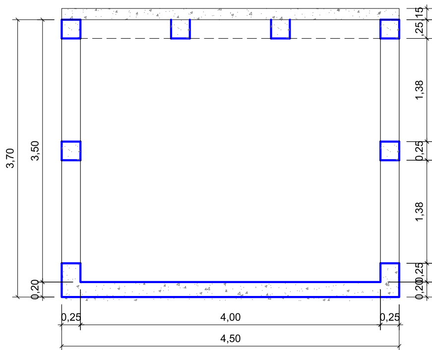
Corte AA
