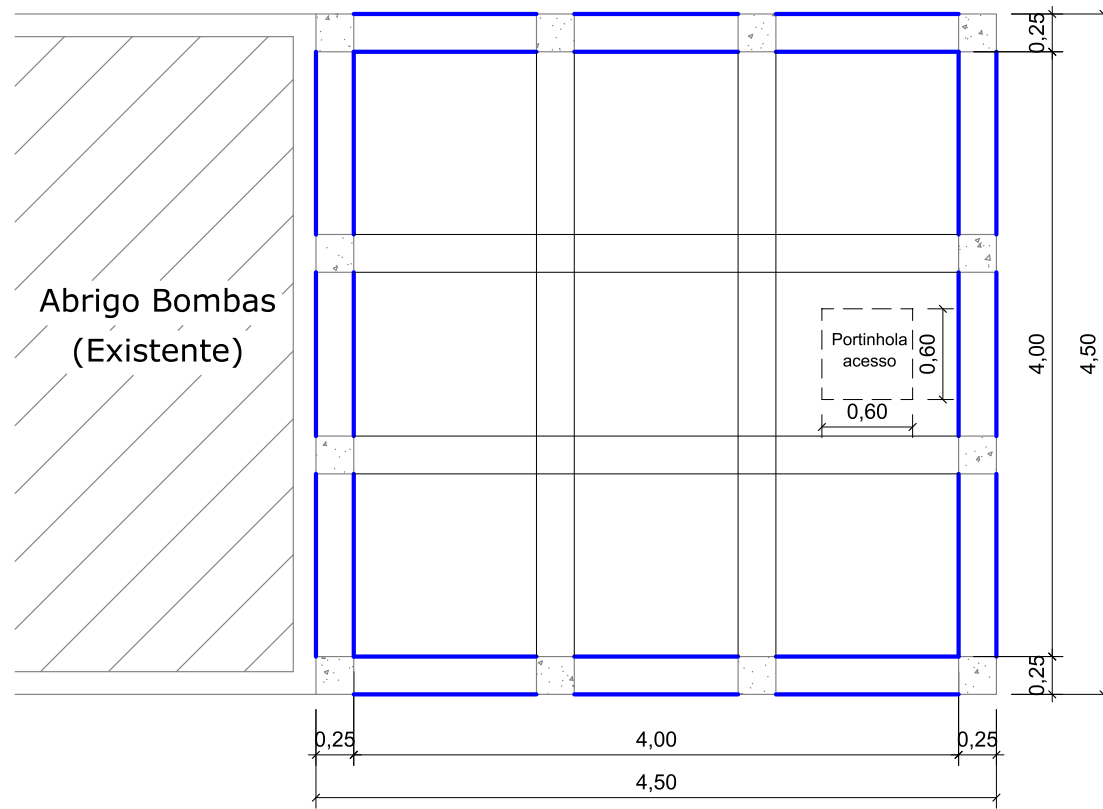
Detalhe viga respaldo
