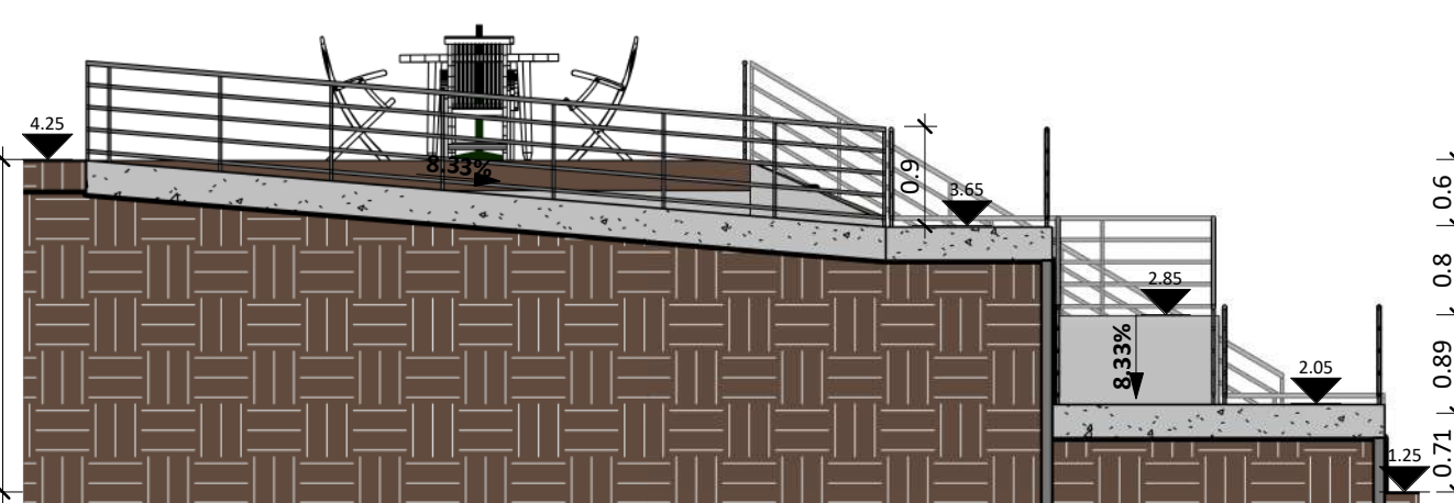
DET. RAMPA ESC: 1:75
