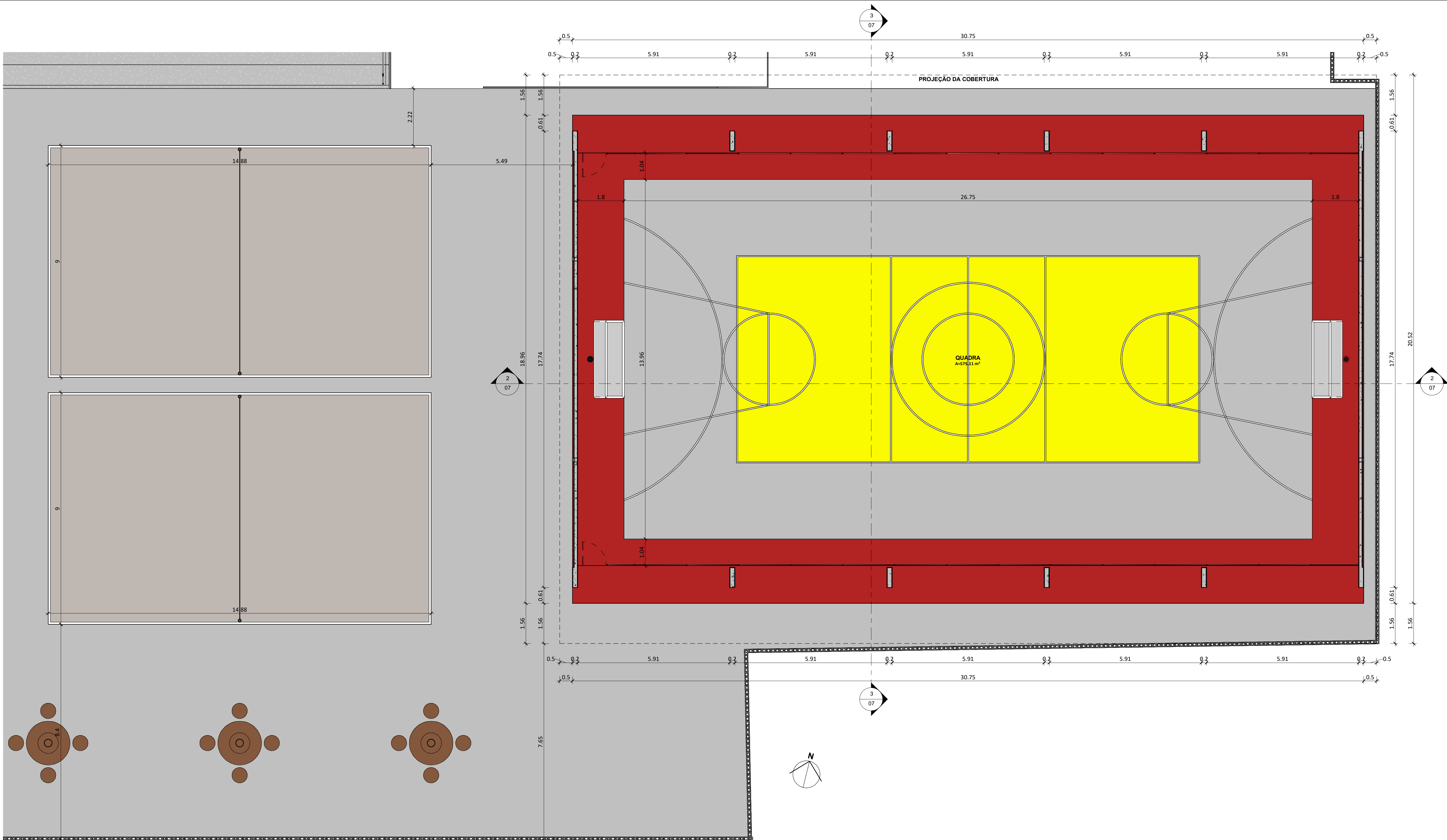
PLANTA QUADRA ESC: 1:75
