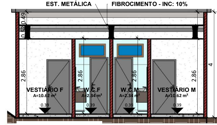
CORTE E ESC: 1:75
