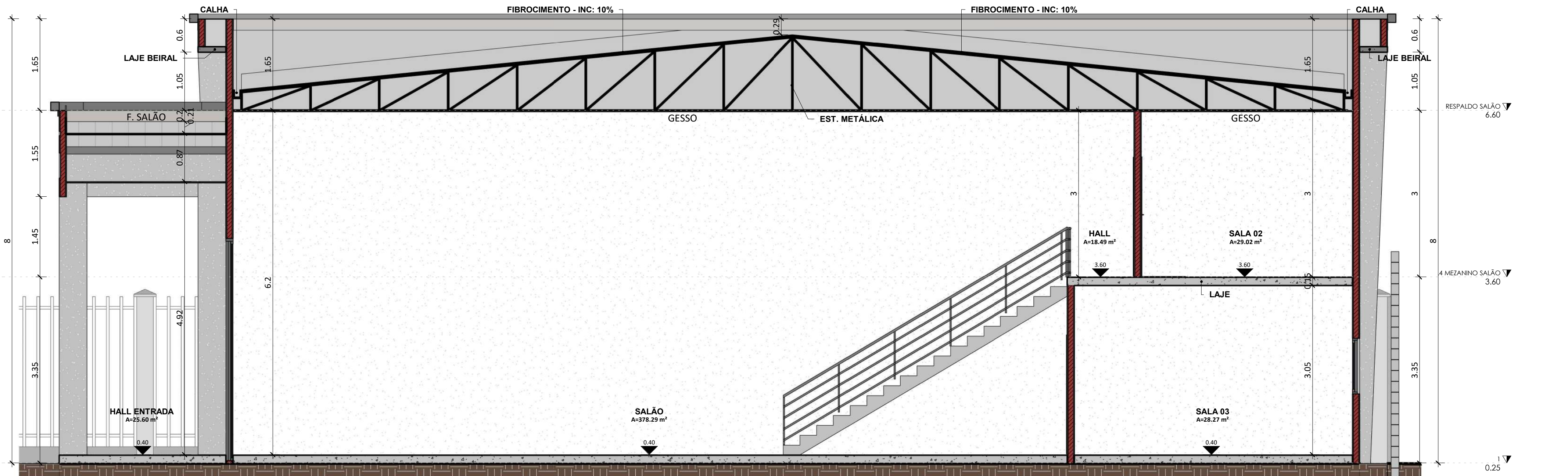
CORTE A ESC: 1:50
