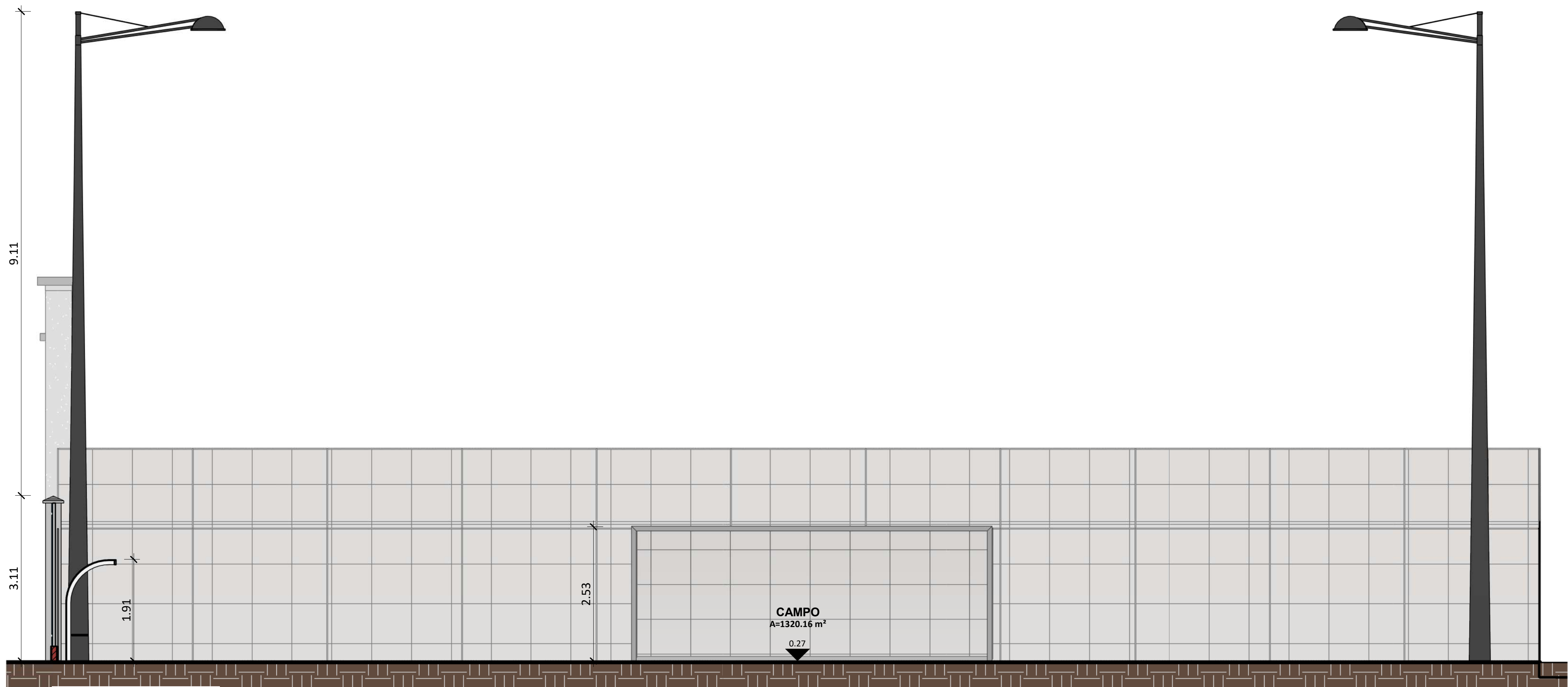
CORTE J ESC: 1:75
