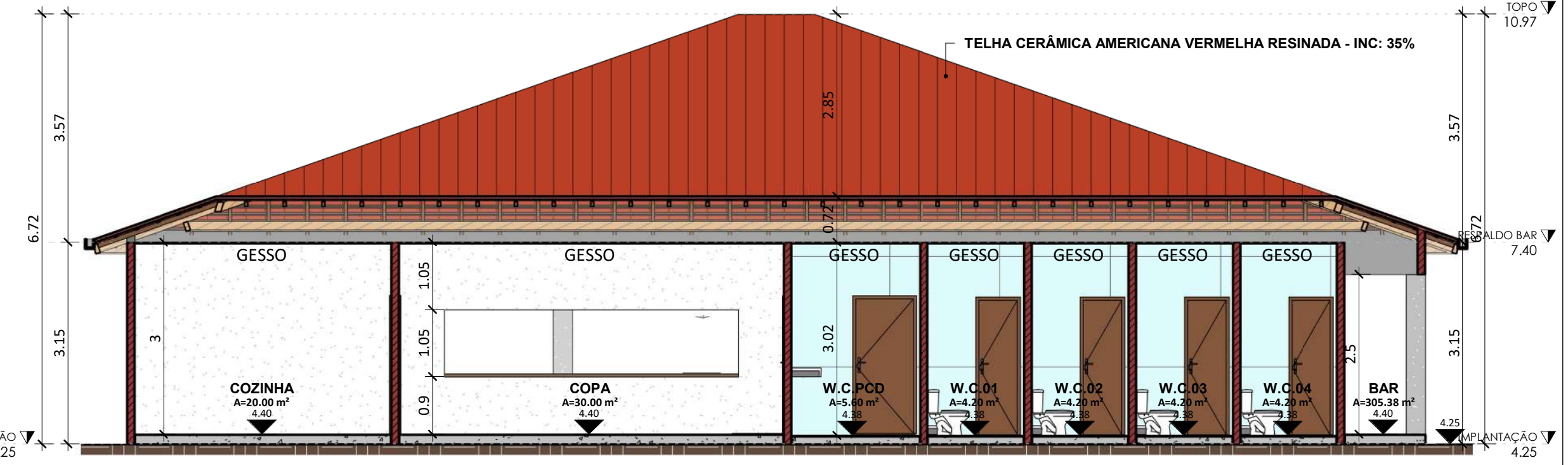
CORTE H ESC: 1:75
