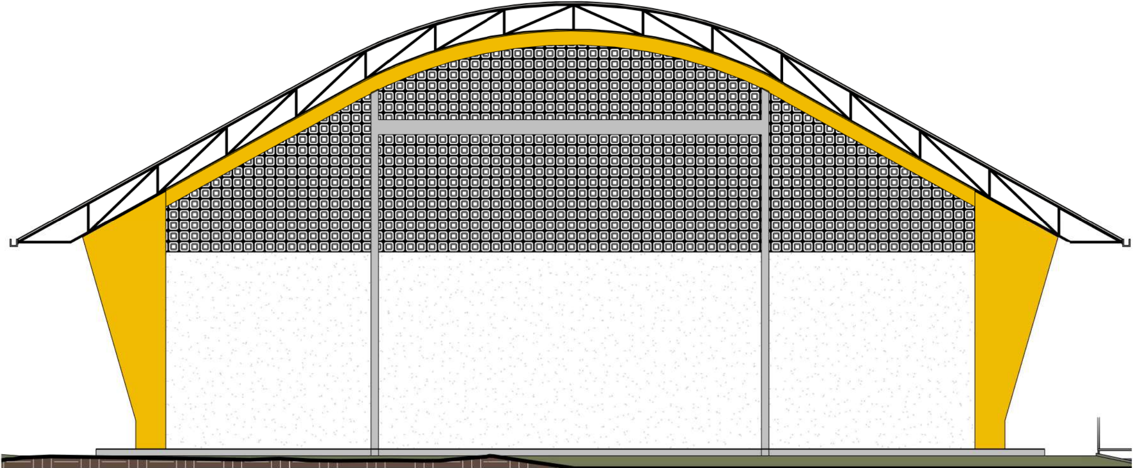
FACHADA POSTERIOR - QUADRA ESC: 1:75
