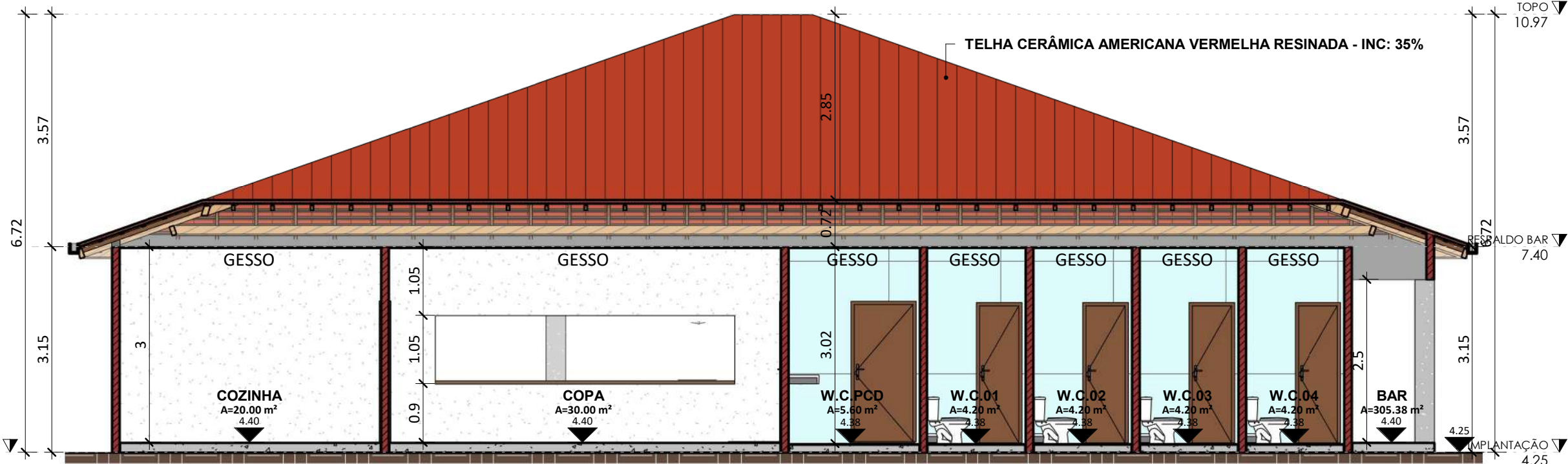
CORTE H ESC: 1:75
