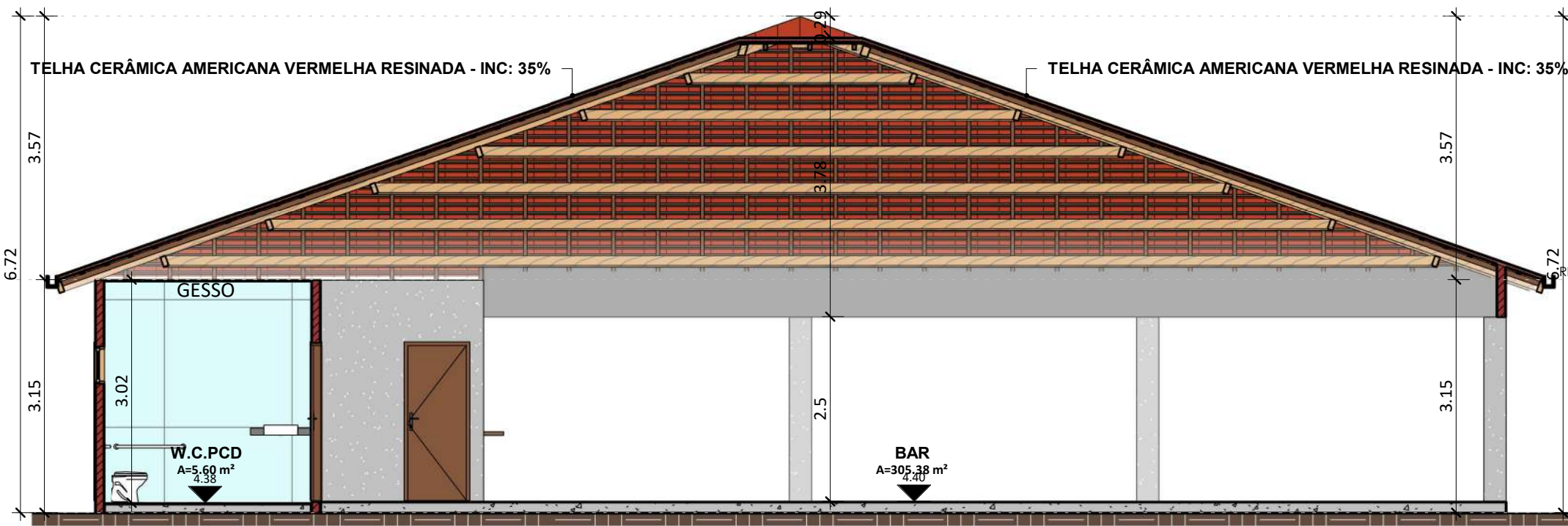
CORTE G ESC: 1:75
