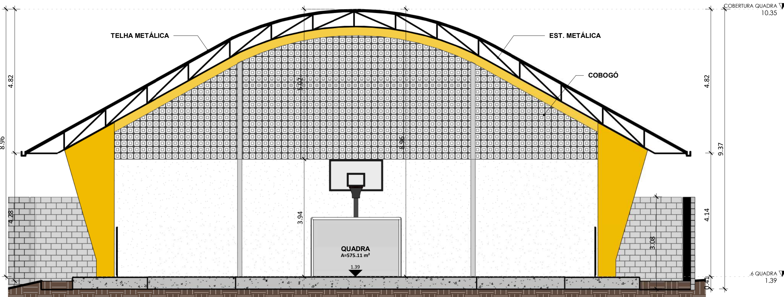
CORTE L ESC: 1:75
