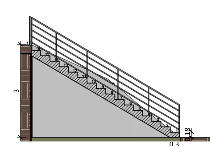
DET. ESCADA ESC: 1:75
