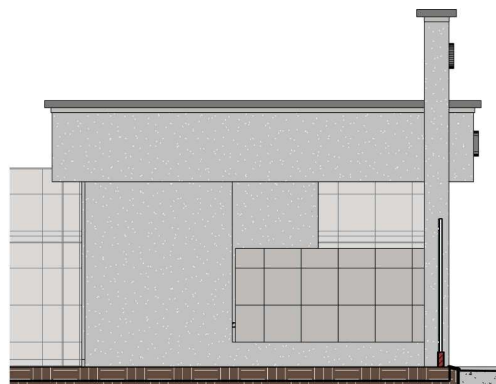
FACHADA L. ESQUERDA - GUARITA ESC: 1:75
