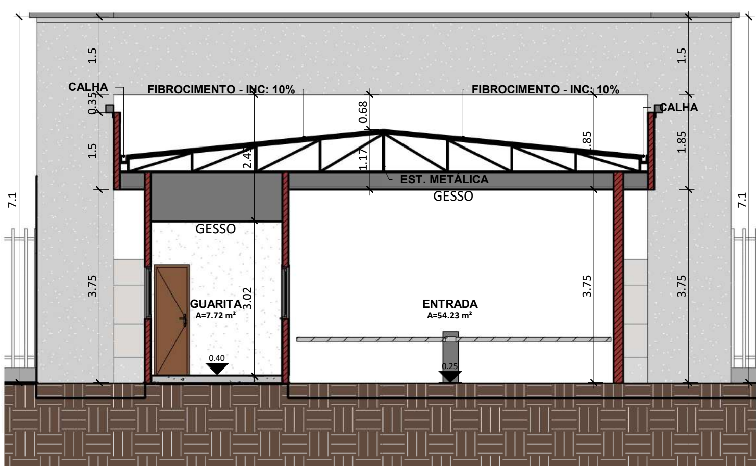
CORTE C ESC: 1:75
