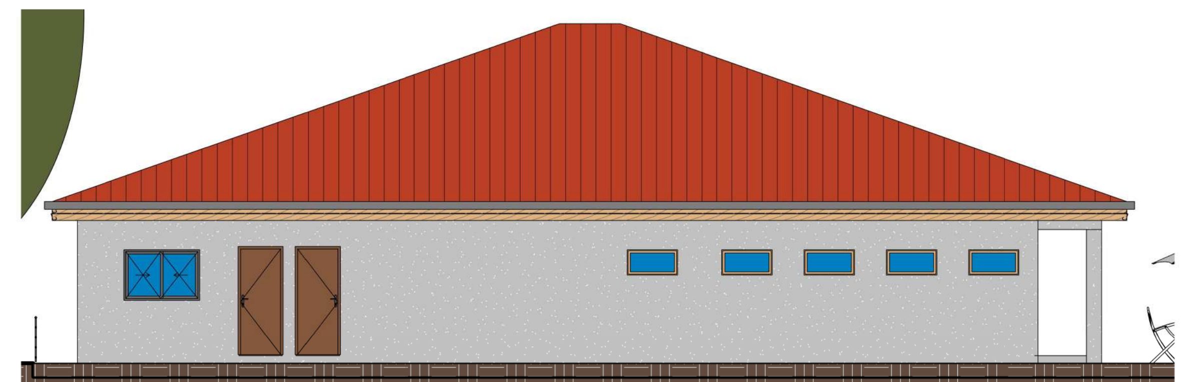
FACHADA POSTERIOR - BAR ESC: 1:75
