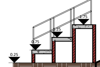
ARQUIBANCADA ESC: 1:75
