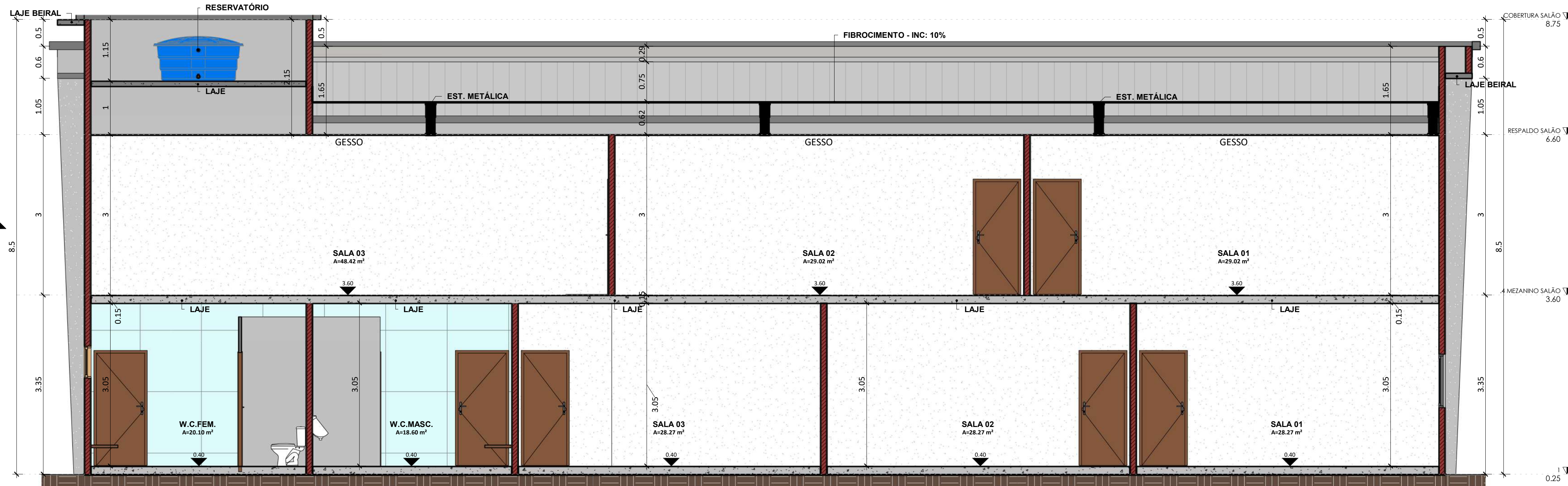
CORTE B ESC: 1:50
