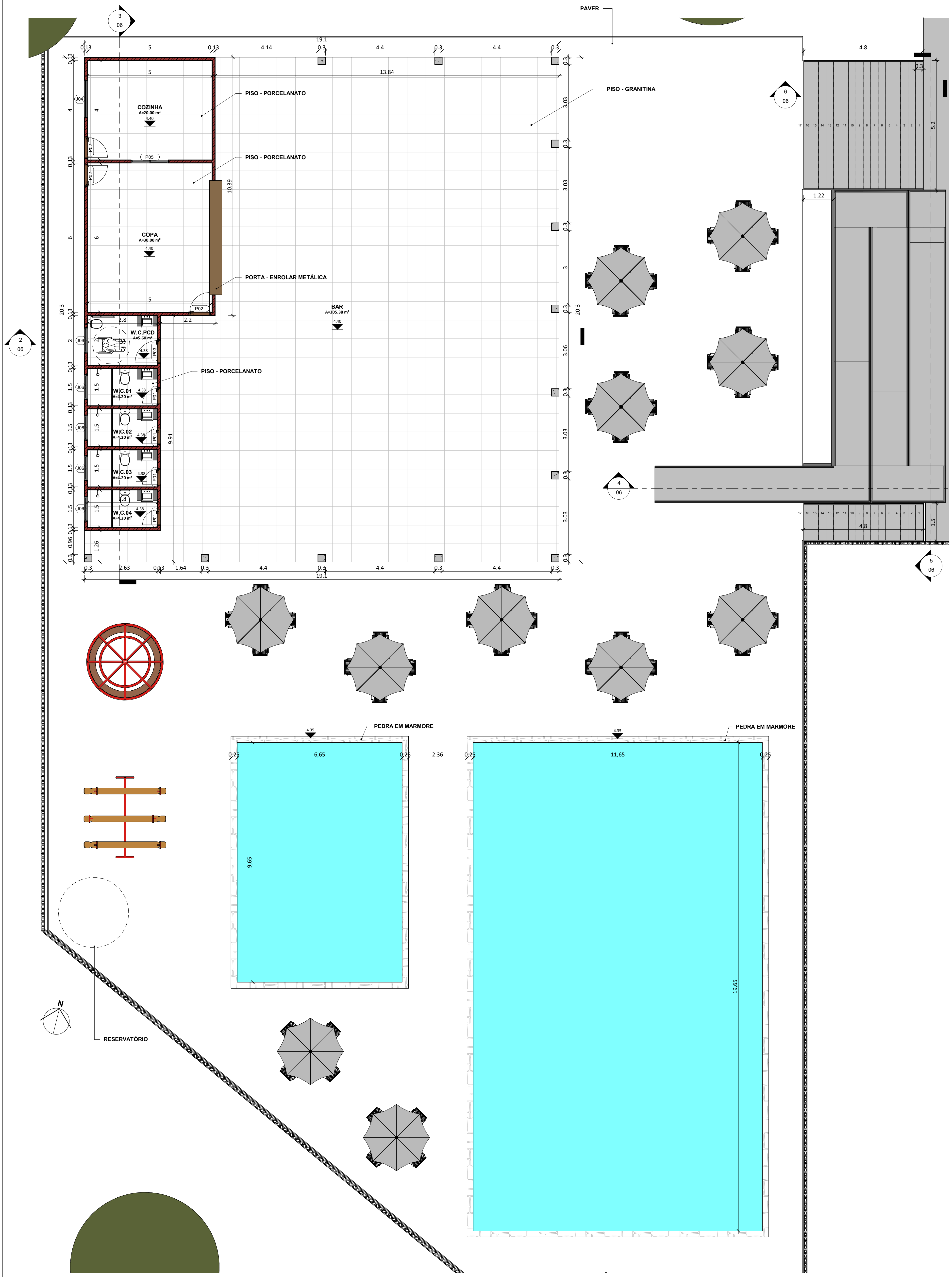
PLANTA LANCHONETE ESC: 1:75
