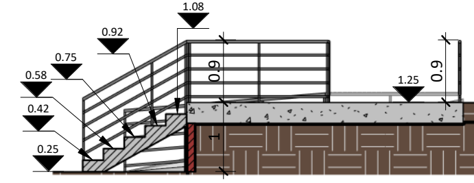
DET. RAMPA ESC: 1:75
