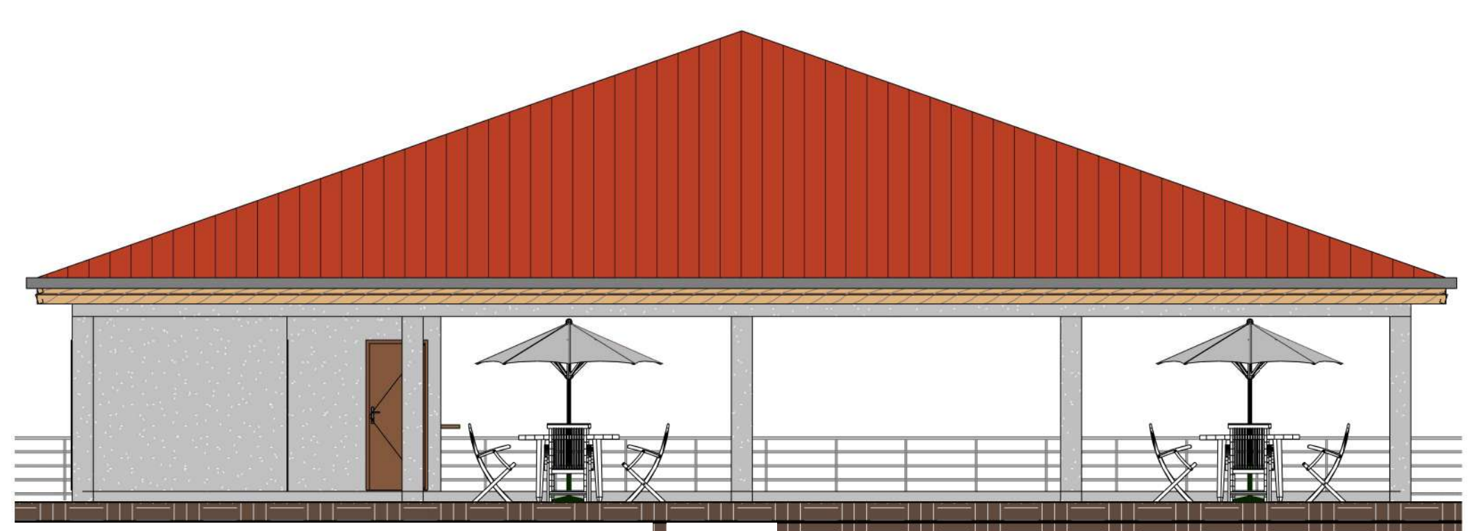
FACHADA L. ESQUERDA - BAR ESC: 1:75
