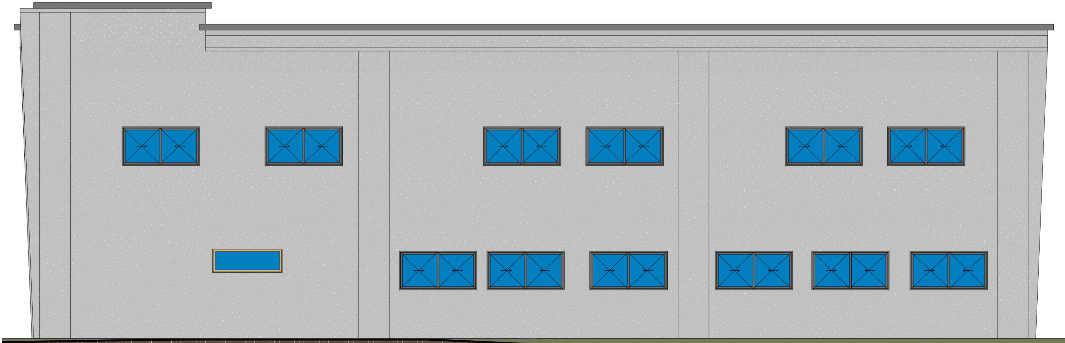
FACHADA POSTERIOR - SALÃO ESC: 1:50
