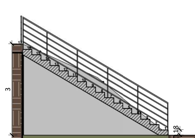
DET. ESCADA ESC: 1:75
