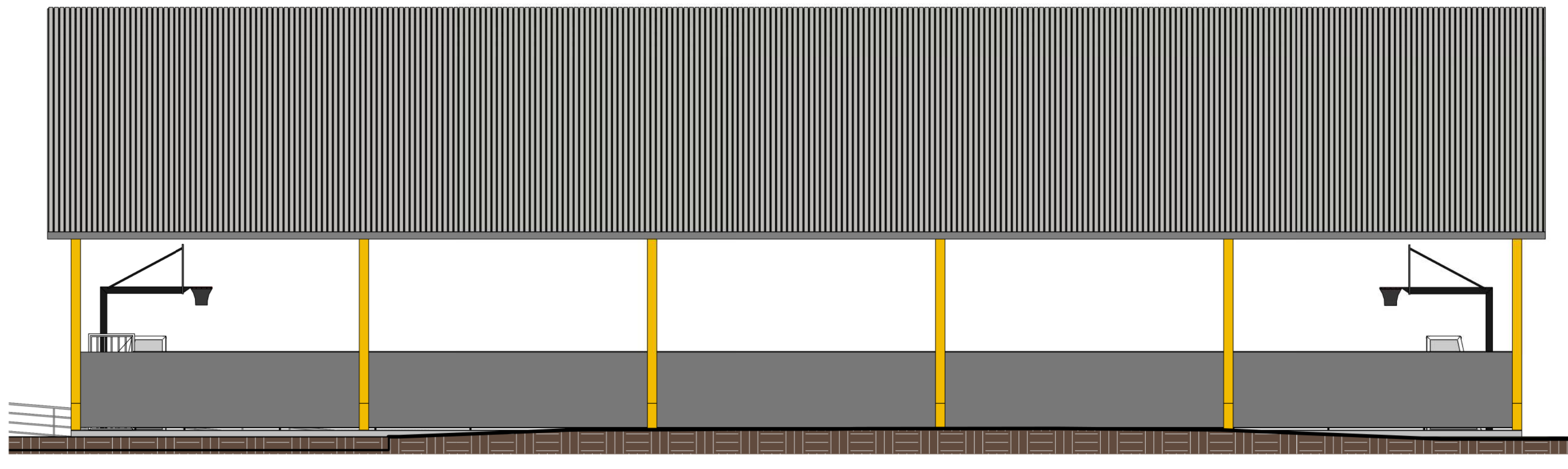
FACHADA L. DIREITA - QUADRA ESC: 1:75
