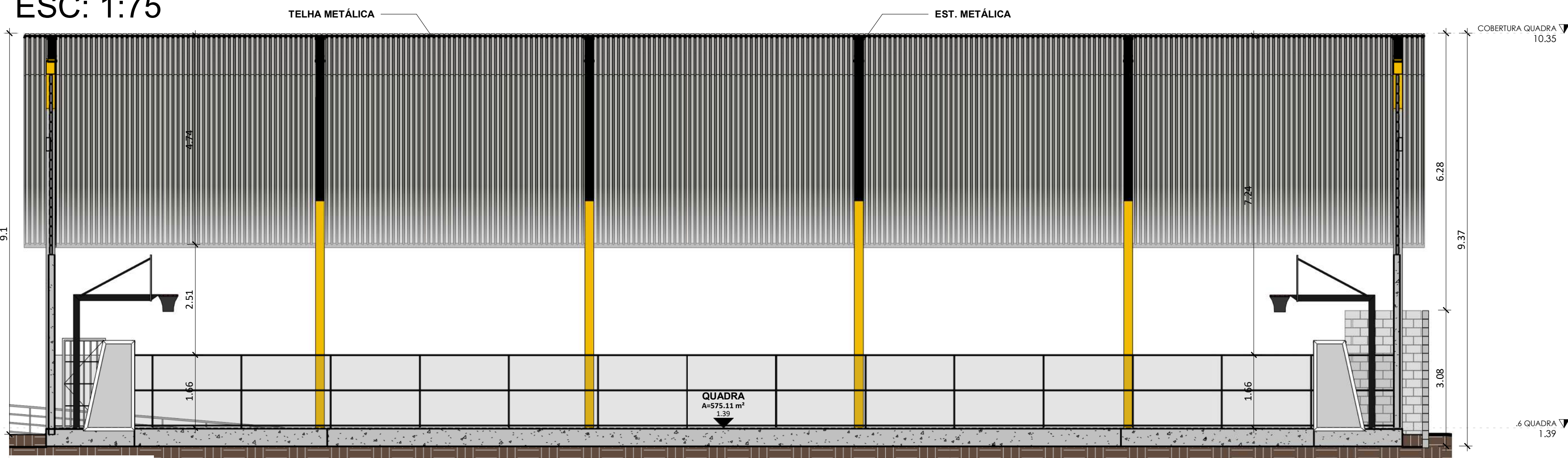
CORTE K ESC: 1:75
