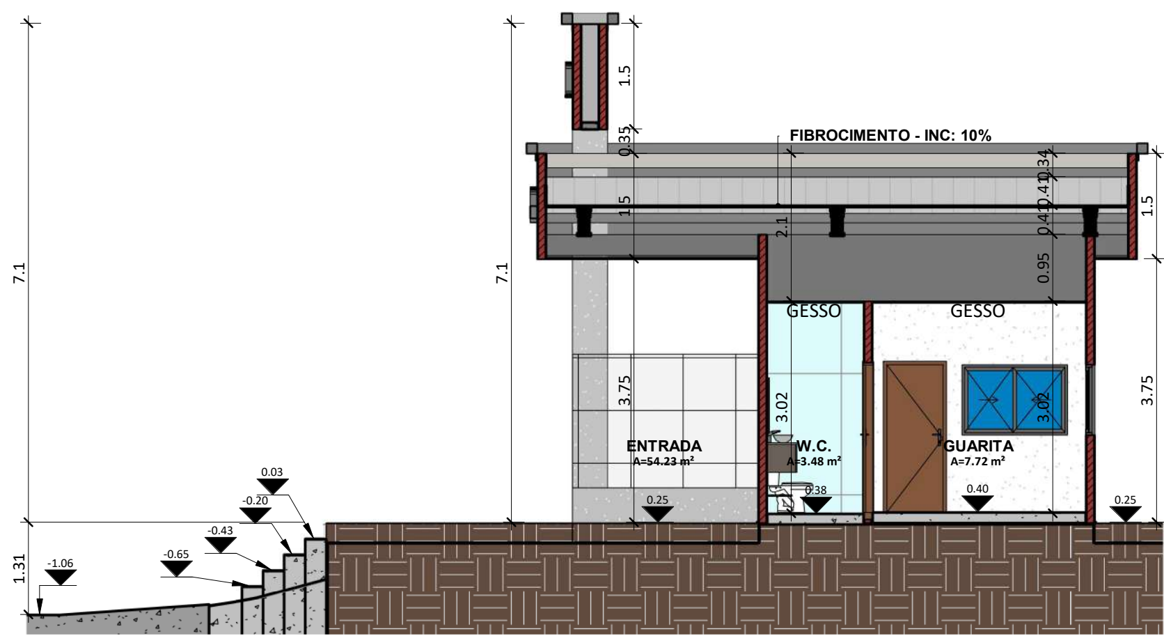
CORTE D ESC: 1:75
