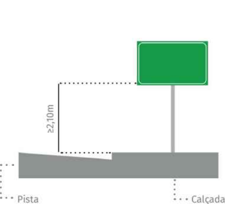
SUPORTES | ALTURA GUIA BRASILEIRO DE SINALIZAÇÃO TURÍSTICA
