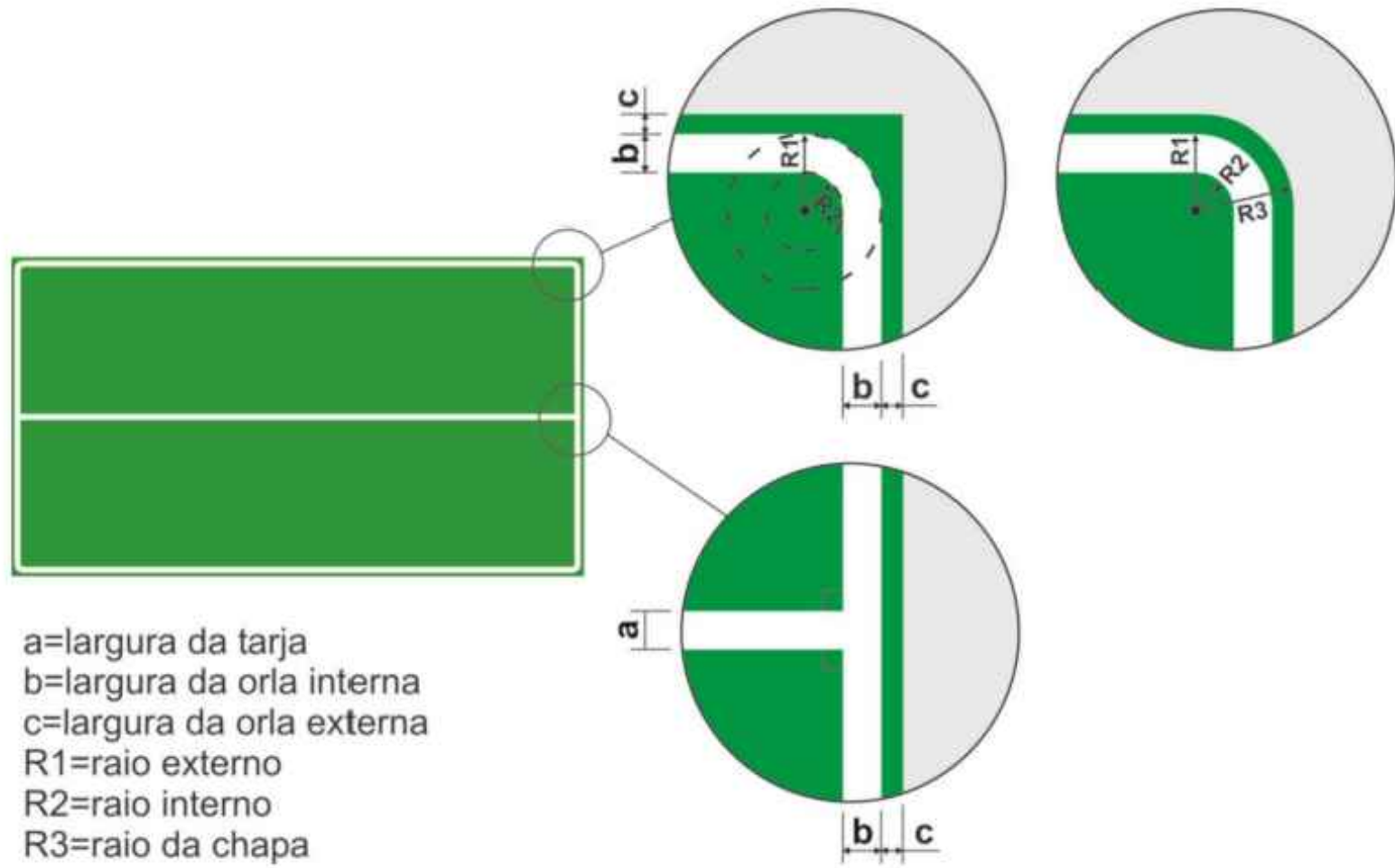
DIMENSIONAMENTO DE ORLAS E TARJAS GUIA BRASILEIRO DE SINALIZAÇÃO TURÍSTICA
