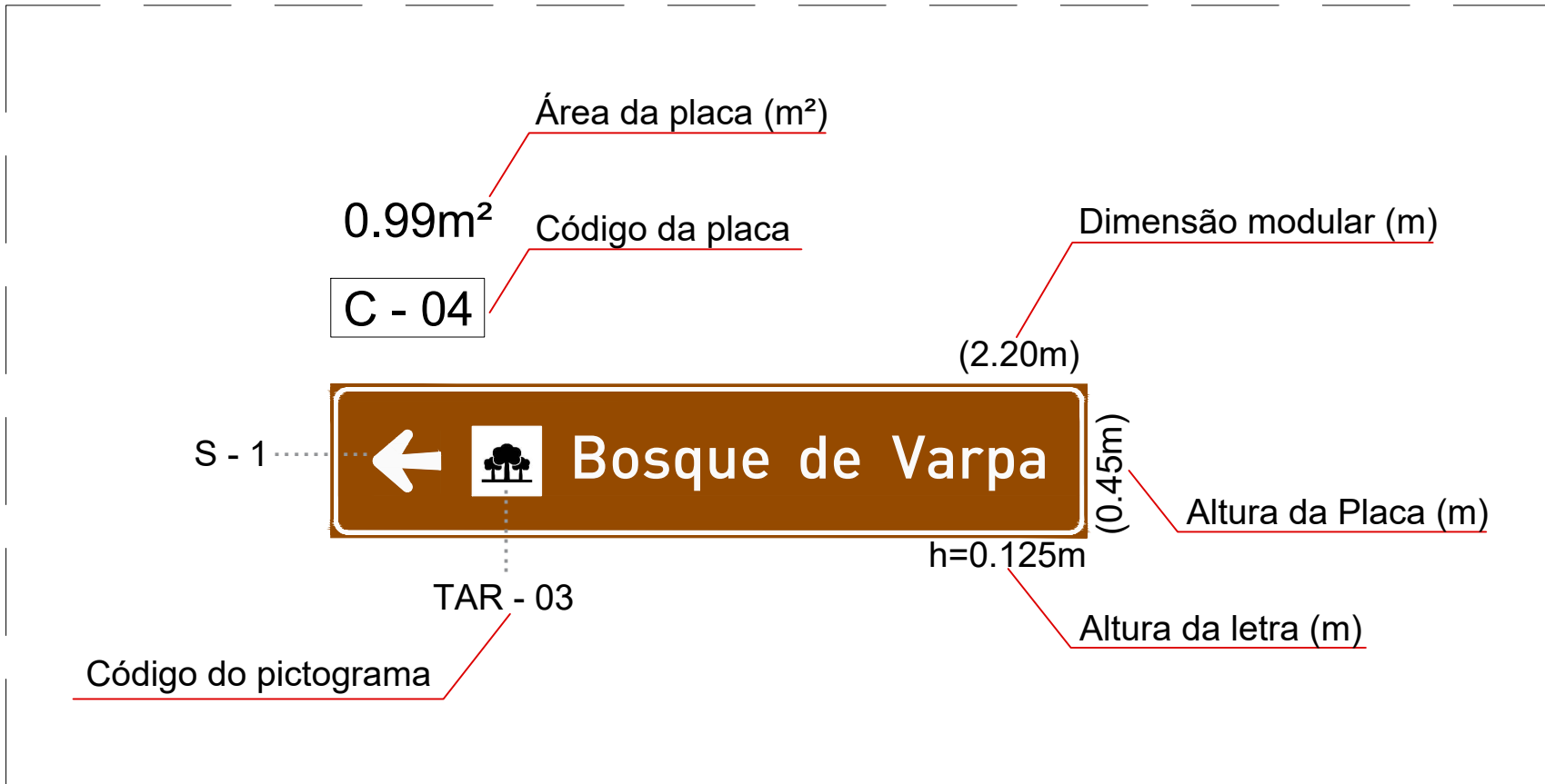
DIAGRAMAÇÃO DAS PLACAS
