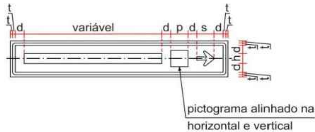
COMPOSIÇÃO VISUAL E ALINHAMENTO GUIA BRASILEIRO DE SINALIZAÇÃO TURÍSTICA
