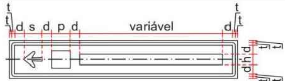
COMPOSIÇÃO VISUAL E ALINHAMENTO GUIA BRASILEIRO DE SINALIZAÇÃO TURÍSTICA
