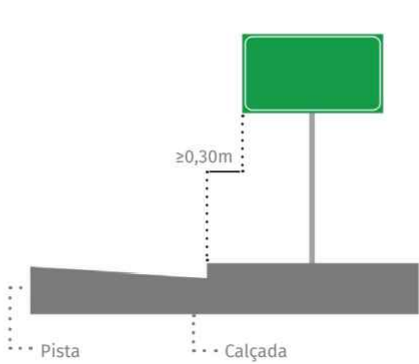
SUPORTES | AFASTAMENTO LATERAL GUIA BRASILEIRO DE SINALIZAÇÃO TURÍSTICA
