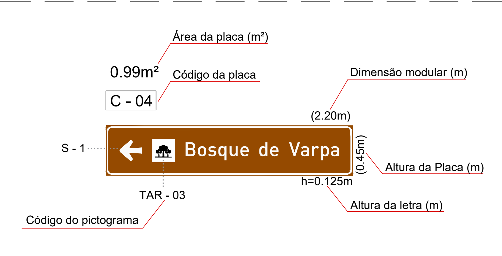
DIAGRAMAÇÃO DAS PLACAS ESCALA: 1/20
