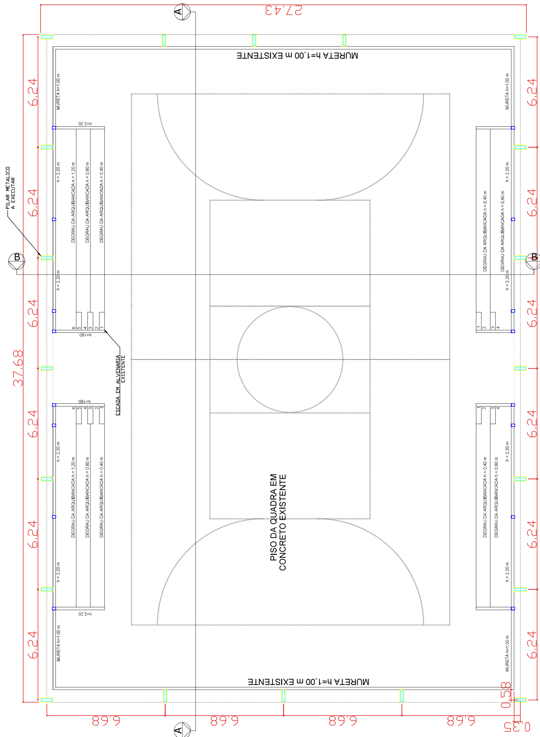
PLANTA PROPOSTA ESC. 1 : 100
