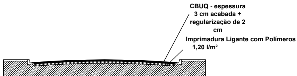
Perfil Genérico da Rua de paralelepípedo
