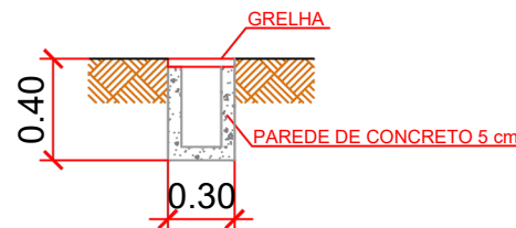
CORTE TRANSVERSAL SITUAÇÃO S/ ESCALA
