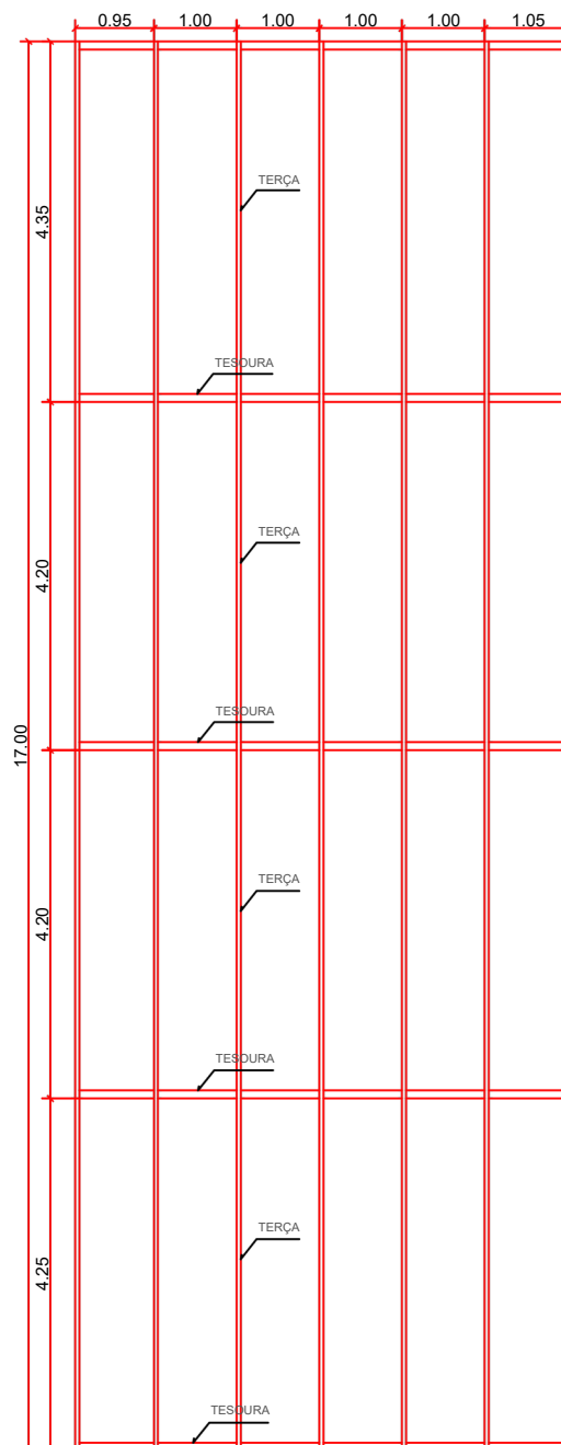
PLANTA BAIXA ESTRUTURA METÁLICA ESCALA 1:100
