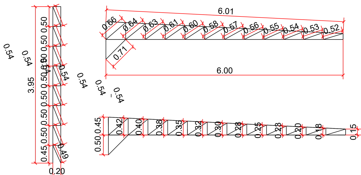
DETALHAMENTO ESTRUTURA METÁLICA ESCALA 1:50
