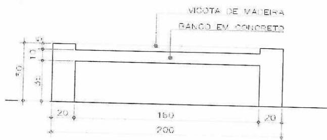
DETALHE — BANCO VISTA FRONTAL ESCALA 1:20 MEDIDAS EM CM
