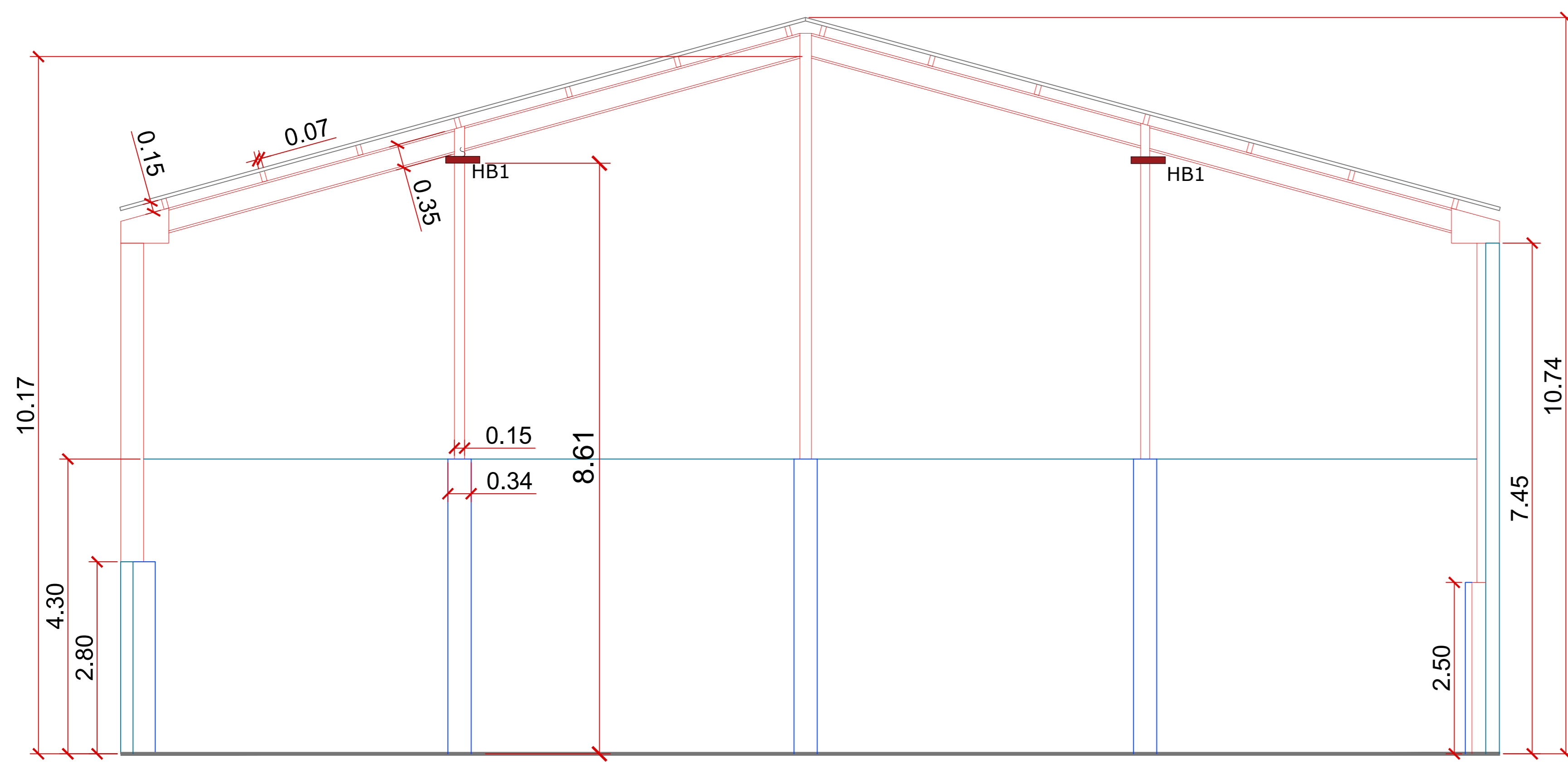
CORTE A-A - PISTA DE SKATE escala 1 : 50
