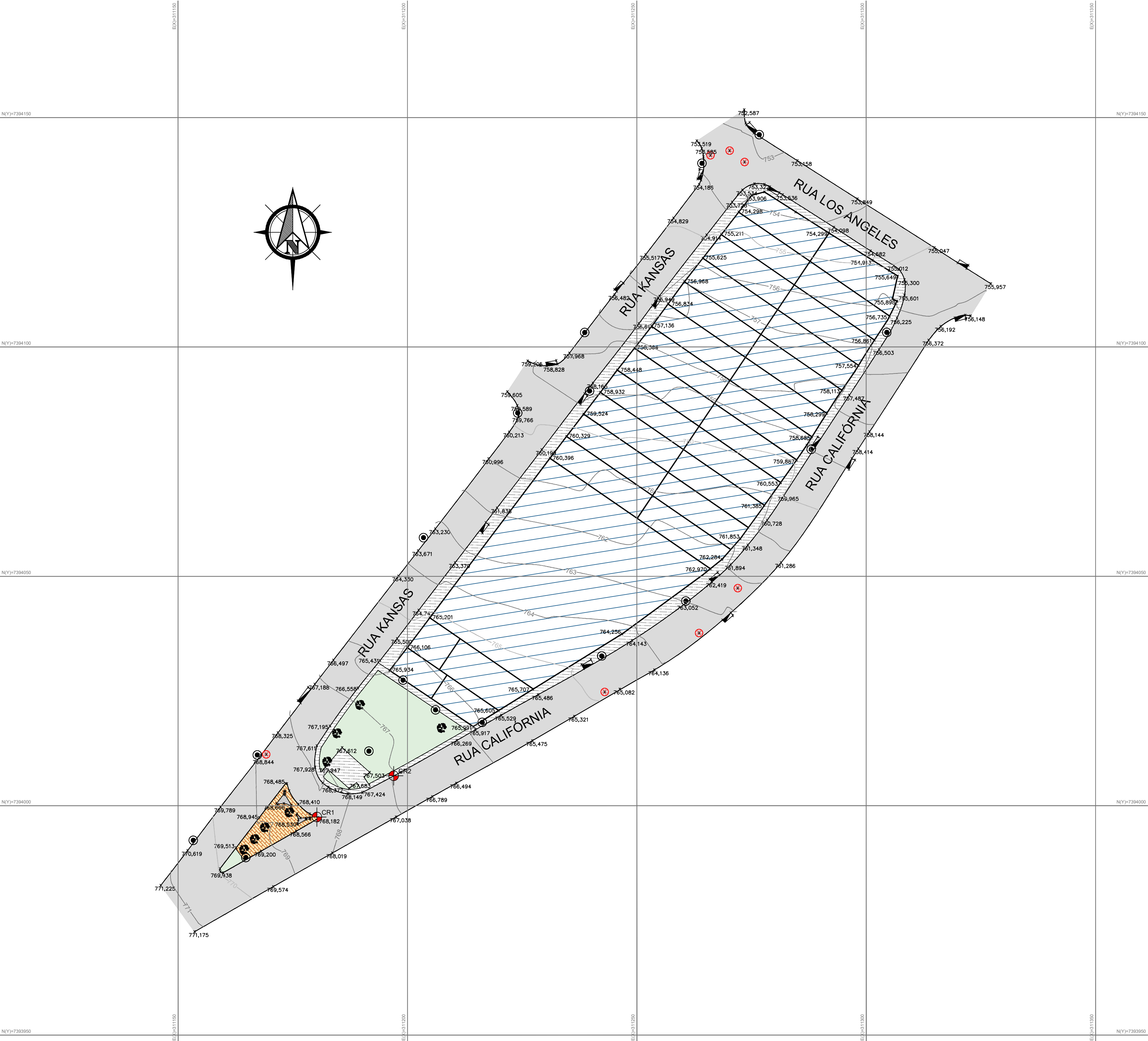
LEVANTAMENTO TOPOGRAFICO ESCALA: 1/500
